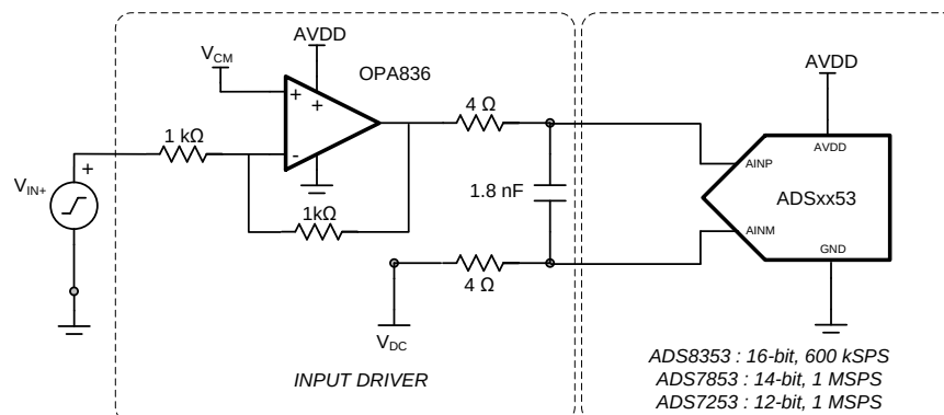
典型应用图
