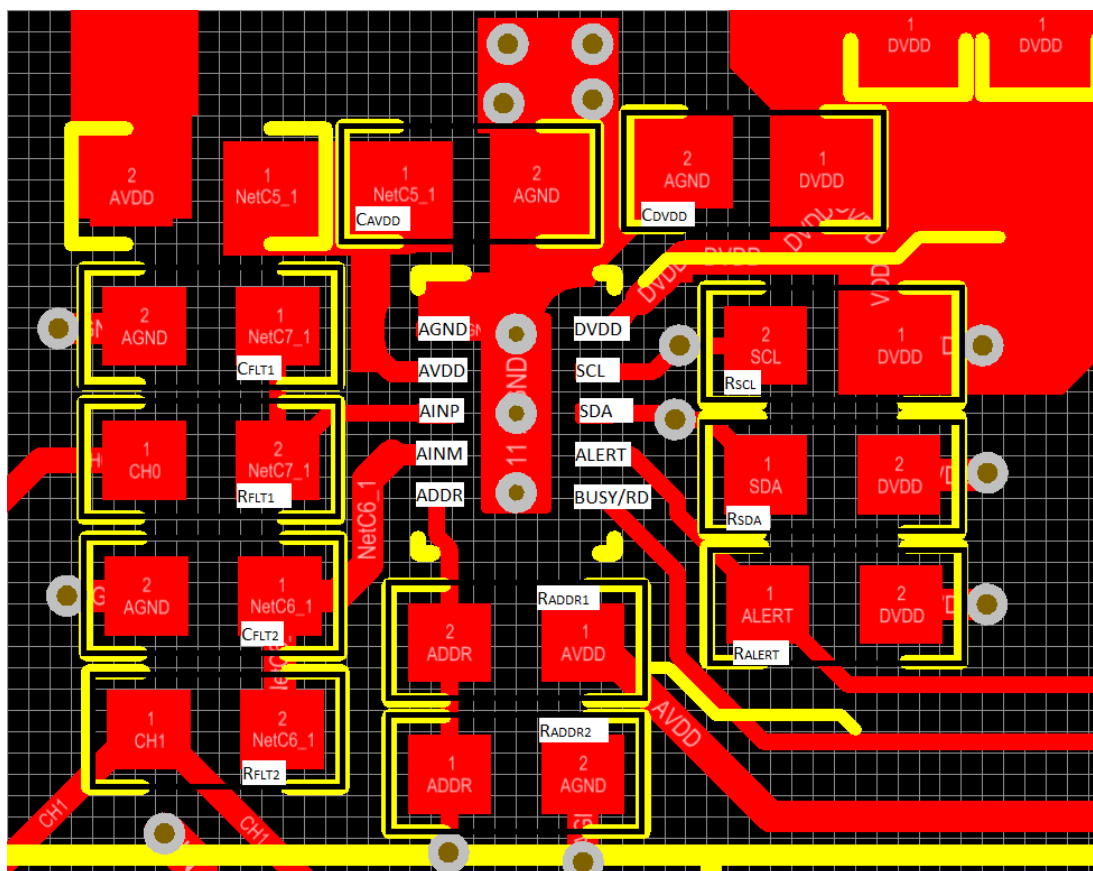
图 8-11. Example Layout
