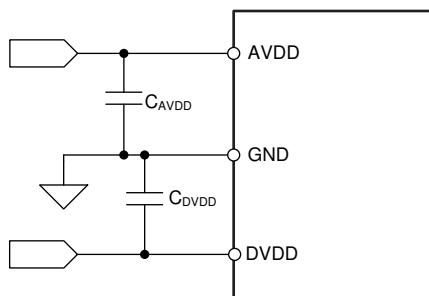
图 8-9. Power-Supply Decoupling
