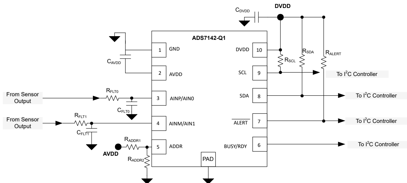
图 8-10. Example Schematic
