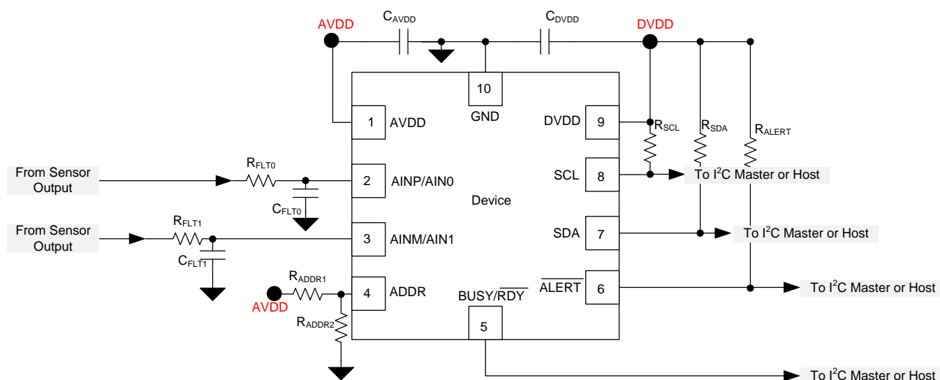
图 123. Example Circuit
