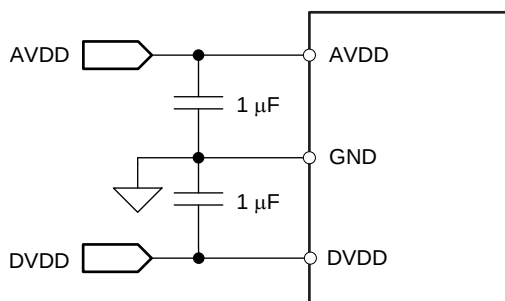
图 140. Power-Supply Decoupling
