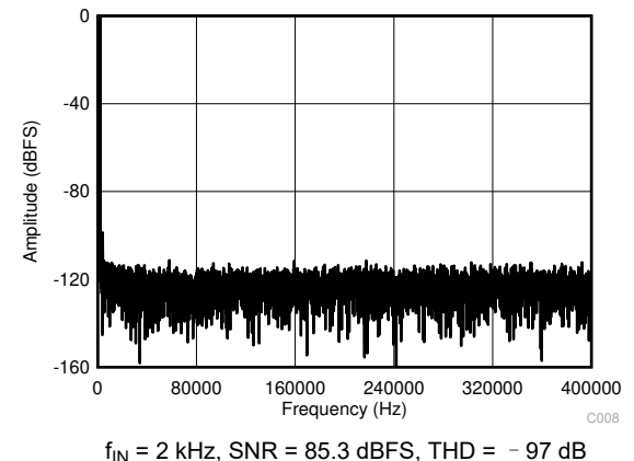
图 5-14. Typical FFT
