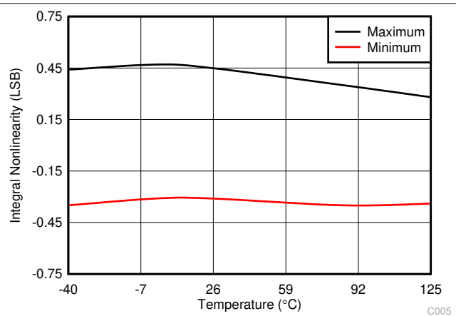
图 7-6. Typical INL
