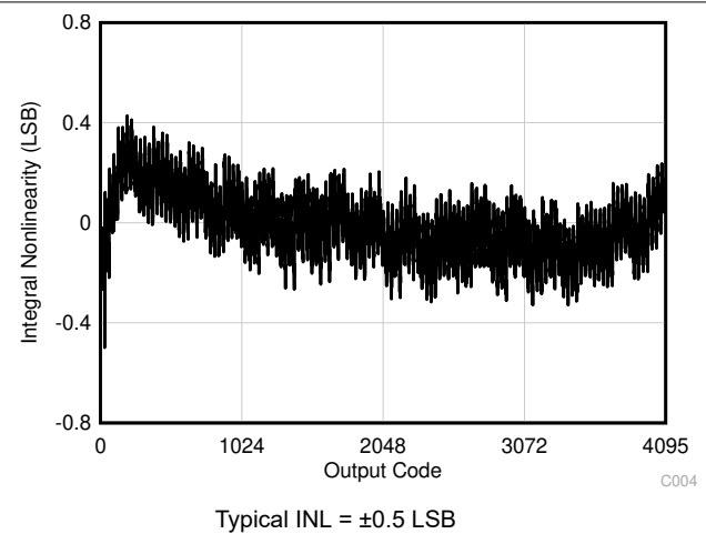
图 7-6. Typical INL
