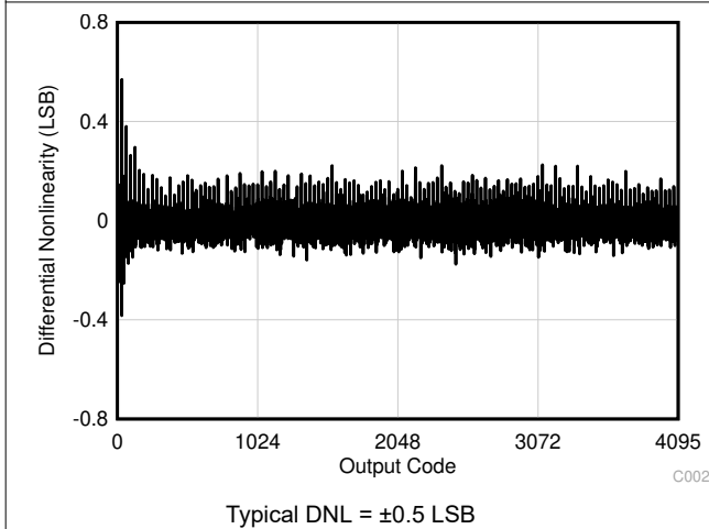
图 7-5. Typical DNL
