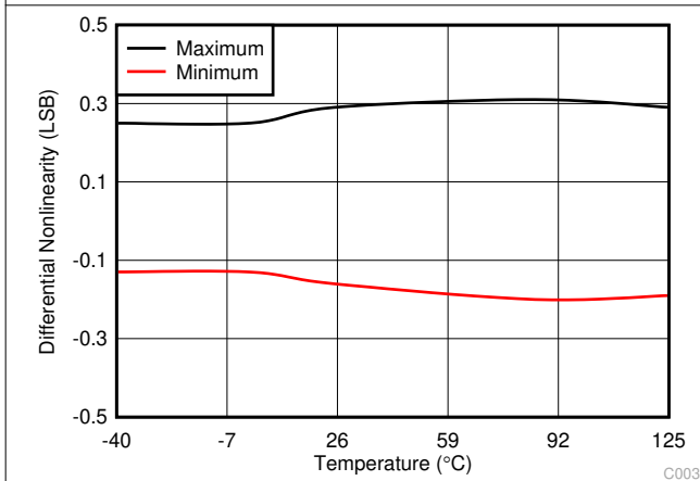
图 7-5. Typical DNL
