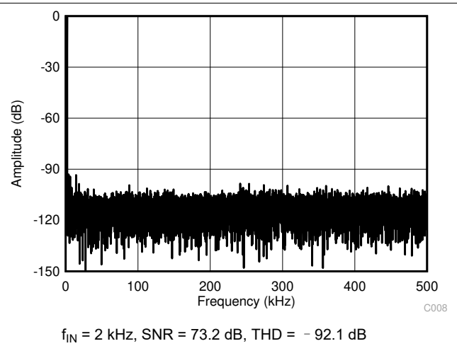
图 7-4. Typical FFT
