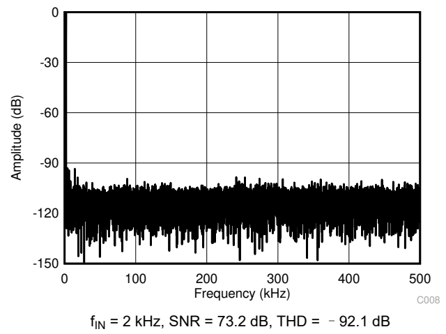
图 6-4. Typical FFT
