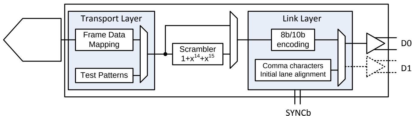
图 45. JESD204B Block
