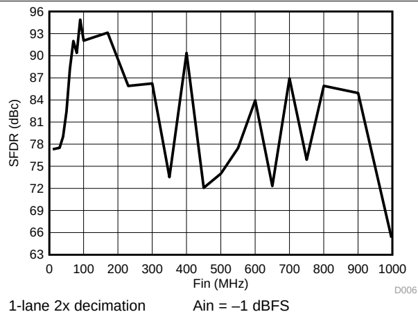
图 10. SFDR vs Frequency
