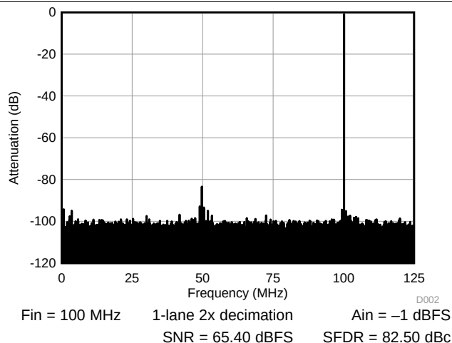
图 7. FFT 100 MHz
