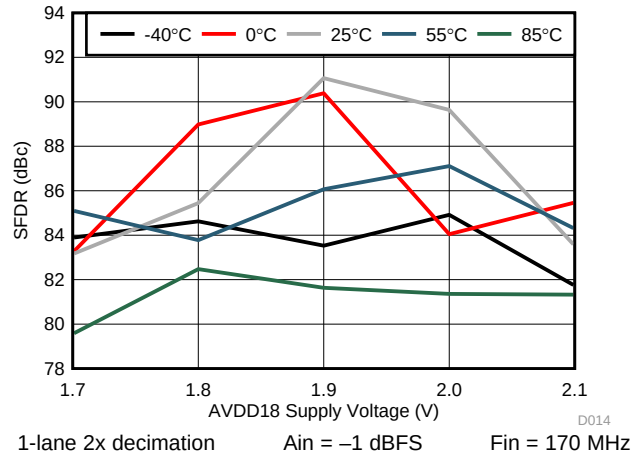
图 18. SFDR vs. AVDD18
