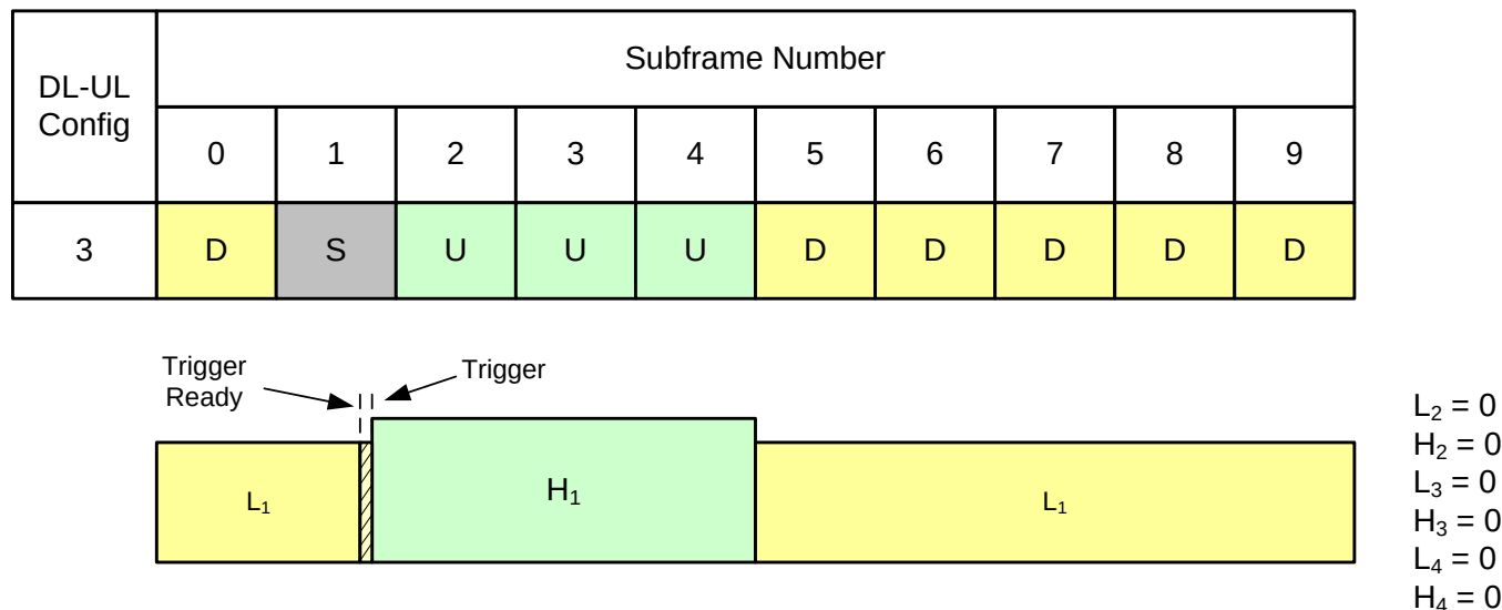
图 61. TDD Burst Mode Example 2
