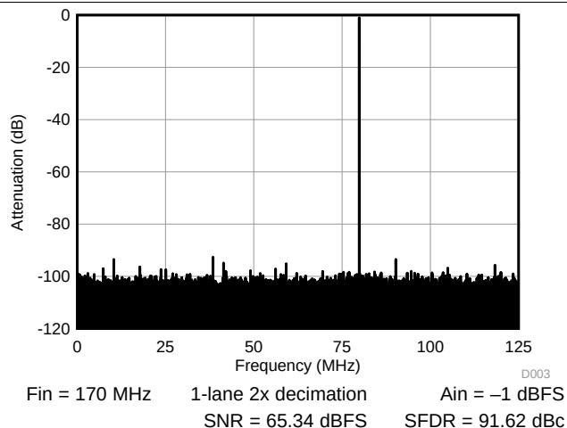
图 8. FFT 170 MHz
