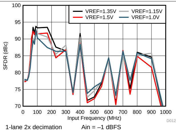
图 16. SFDR vs. VREF
