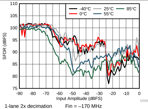
图 12. SFDR vs. Amplitude
