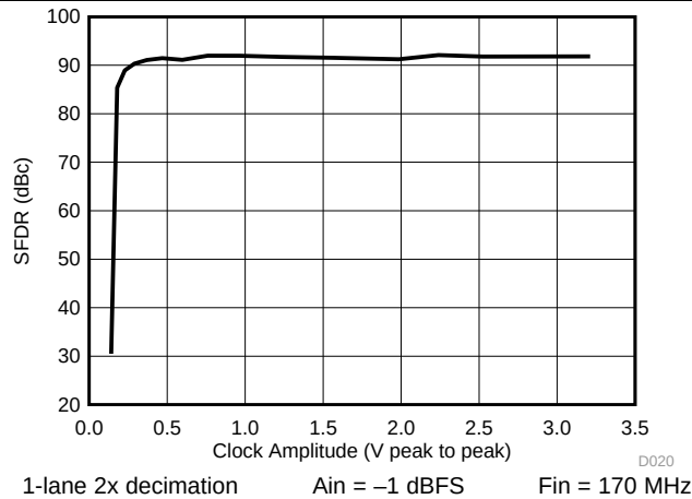
图 24. SFDR vs. Clock Amplitude
