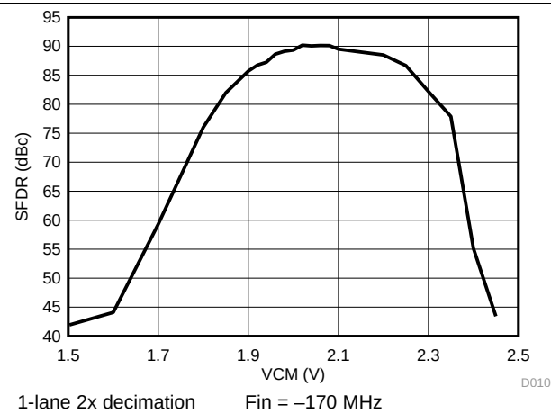
图 14. SFDR vs. VCM
