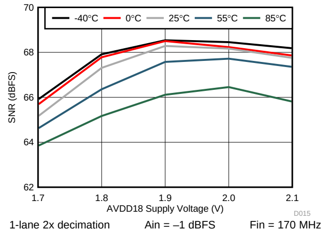
图 19. SNR vs. AVDD18
