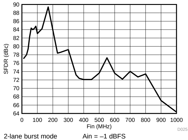
图 30. Burst Mode SFDR vs. Frequency
