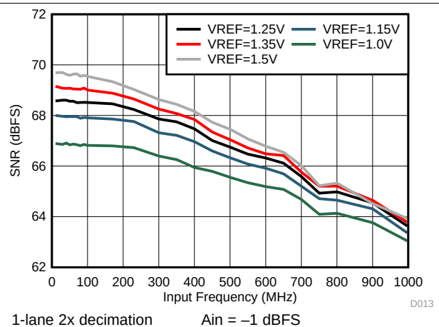
图 17. SNR vs. VREF
