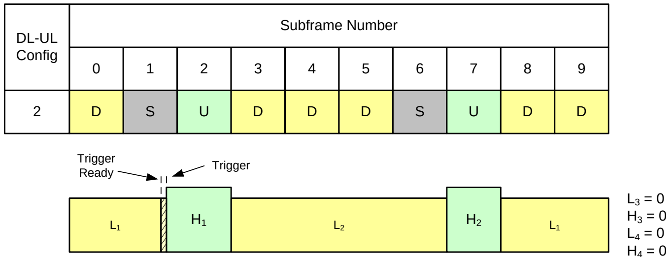
图 60. TDD Burst Mode Example 1
