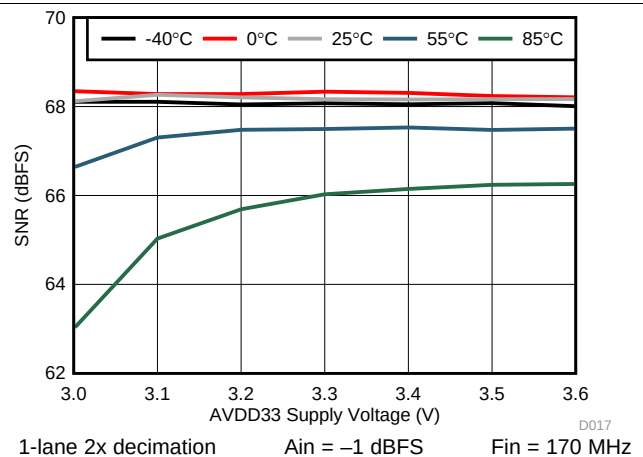
图 21. SNR vs. AVDD33
