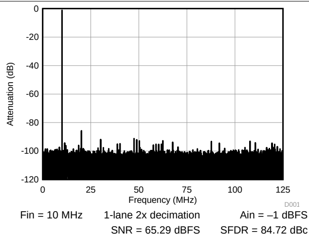
图 6. FFT 10 MHz
