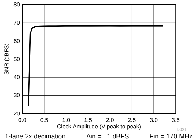
图 25. SNR vs. Clock Amplitude
