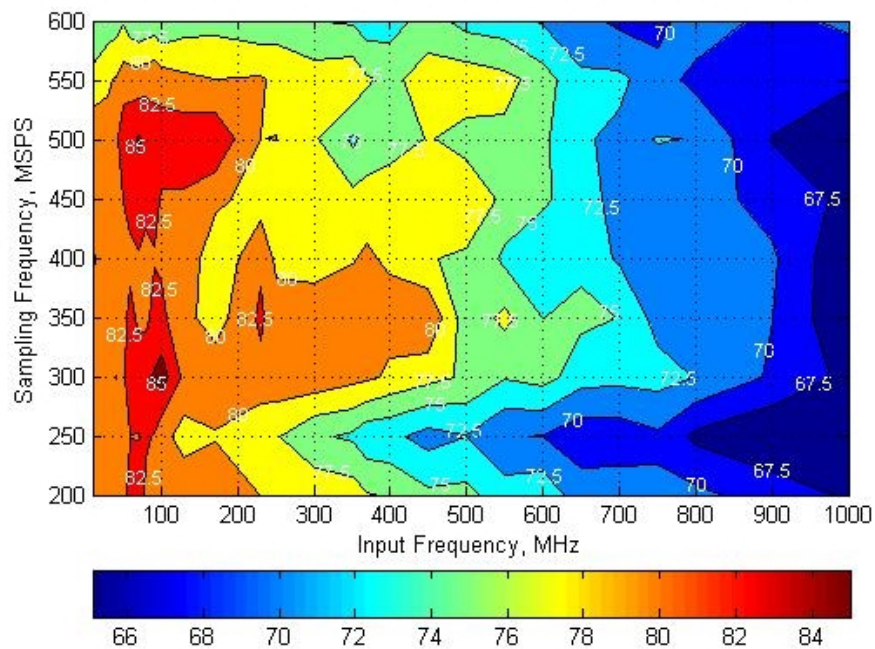
图 38. SFDR Contour Plot
