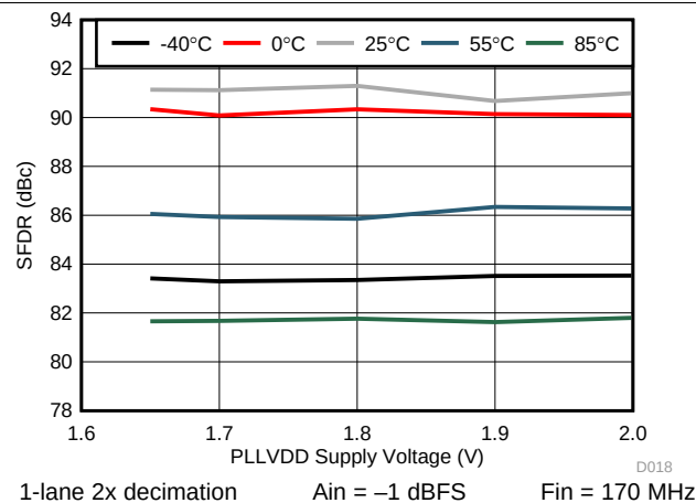
图 22. SFDR vs. PLLVDD
