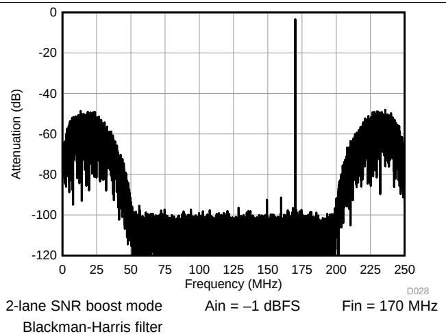
图 33. SNRBoost FFT 170MHz
