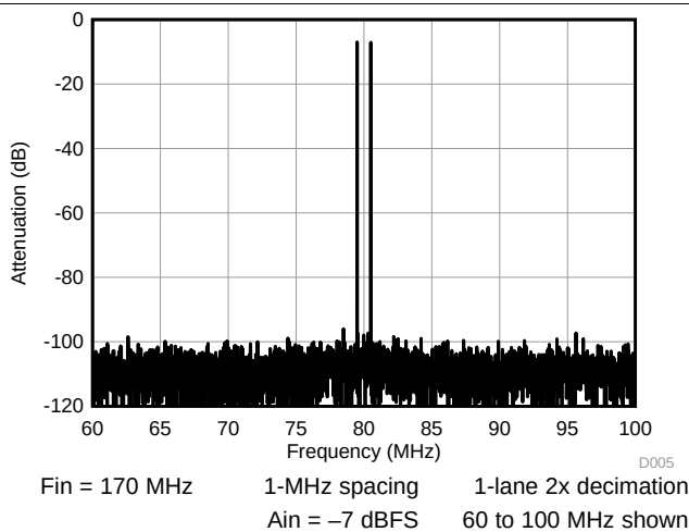
图 26. 2-Tone FFT
