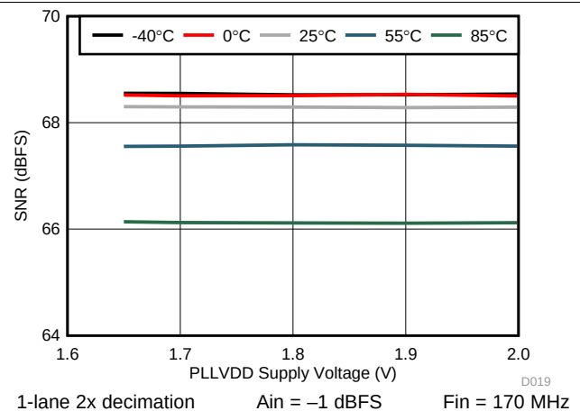
图 23. SNR vs. PLLVDD
