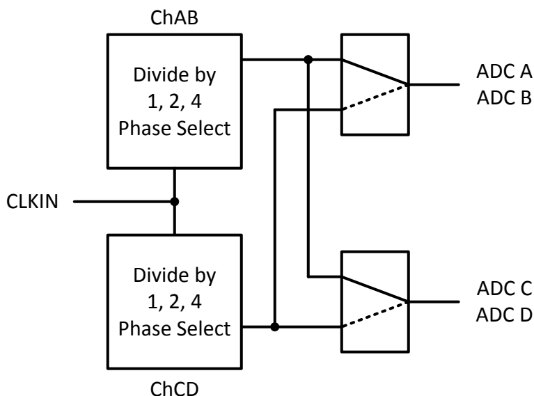
图 54. Input Clock Divider
