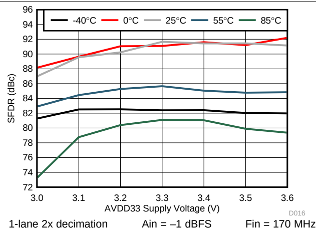
图 20. SFDR vs. AVDD33
