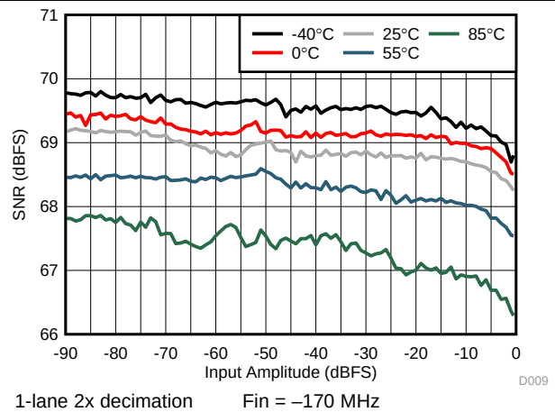
图 13. SNR vs. Amplitude
