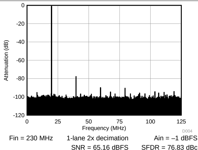
图 9. FFT 230 MHz
