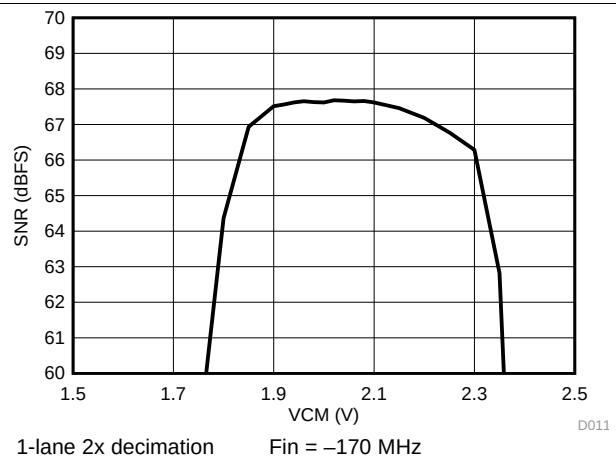
图 15. SNR vs. VCM
