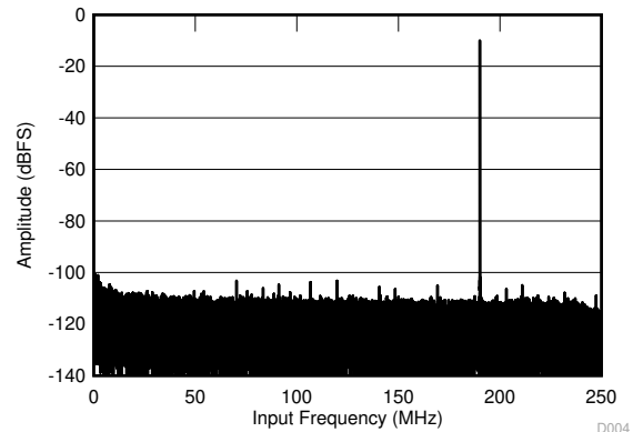
图 6-3. FFT for 190-MHz Input Signal
