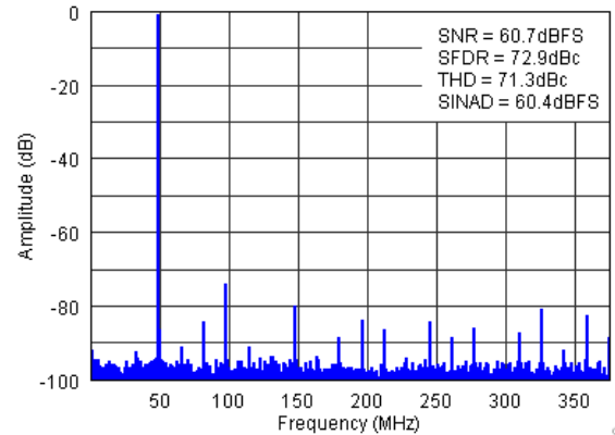
图 7-9. FFT for 700-MHz Input Signal (Auto Off)
