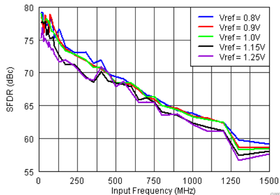
图 7-15. SFDR vs. Vref (Auto On)
