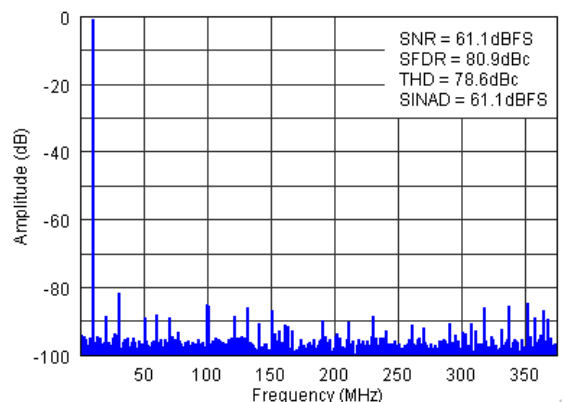
图 7-3. FFT for 10-MHz Input Signal (Auto Off)
