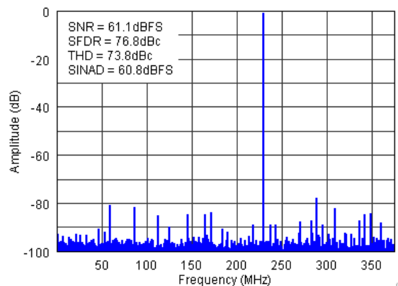
图 7-5. FFT for 230-MHz Input Signal (Auto Off)
