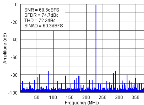
图 7-4. FFT for 230-MHz Input Signal (Auto On)
