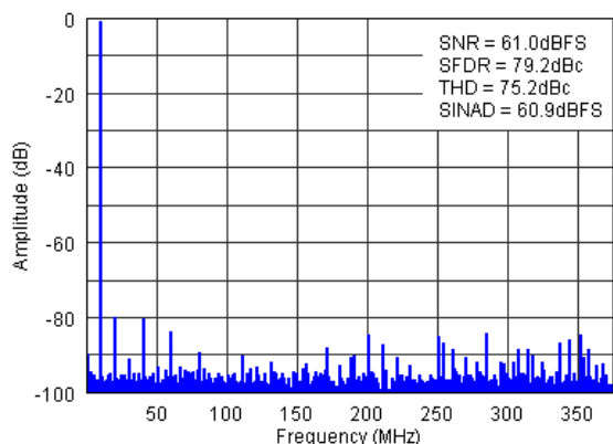
图 7-2. FFT for 10-MHz Input Signal (Auto On)
