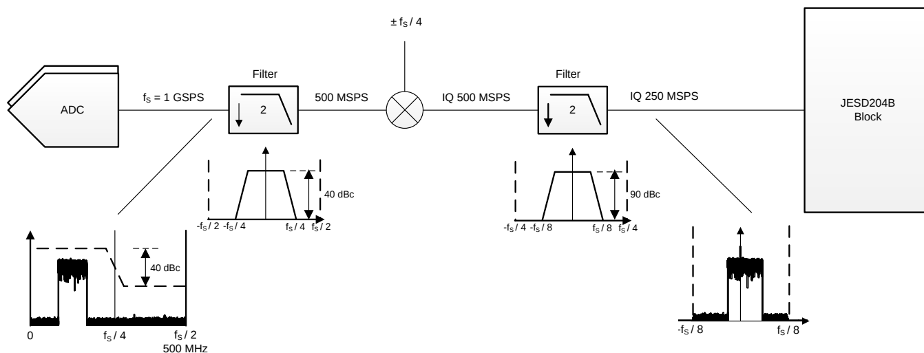
图 54. Operating Mode 0
