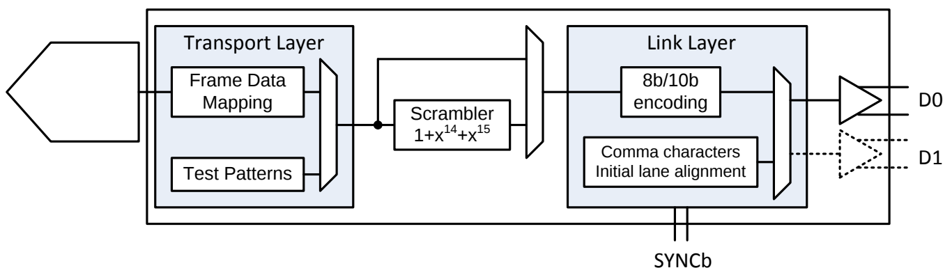
图 60. JESD204B Block
