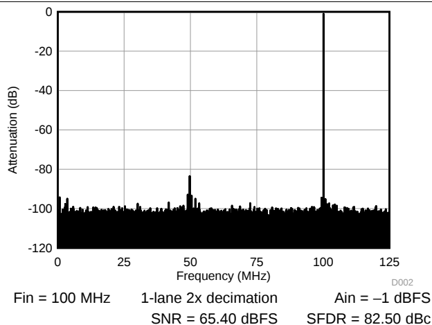
图 6. FFT 100 MHz
