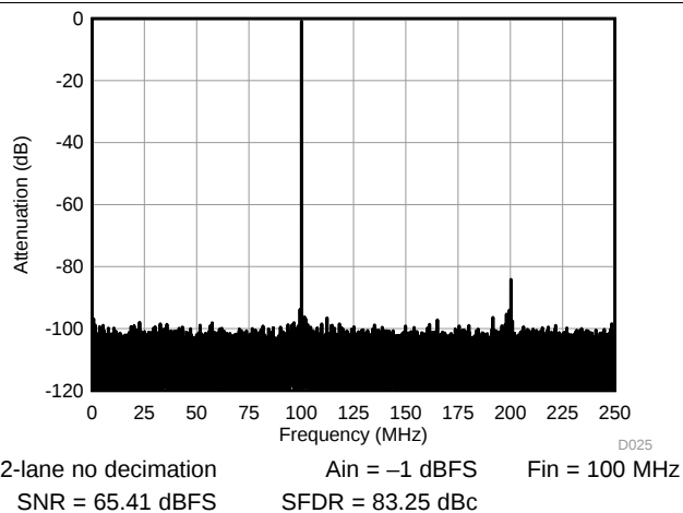
图 29. FFT 100 MHz
