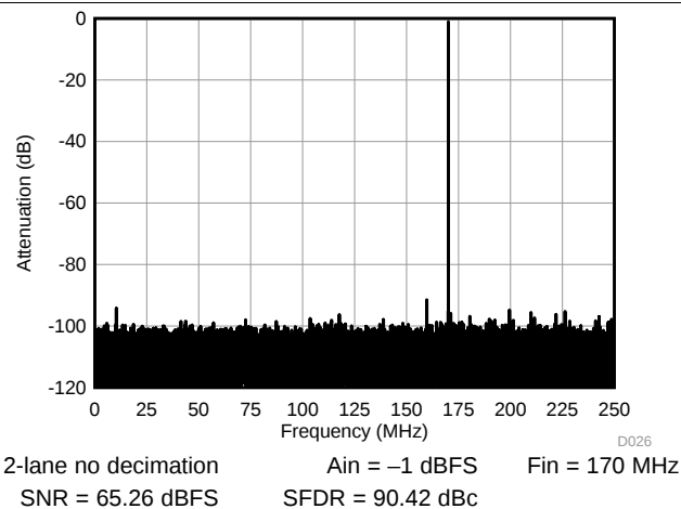
图 30. FFT 170 MHz
