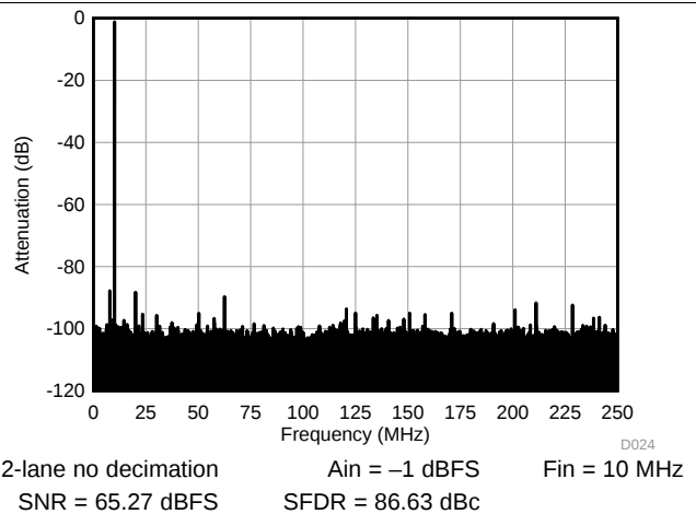
图 28. FFT 10 MHz
