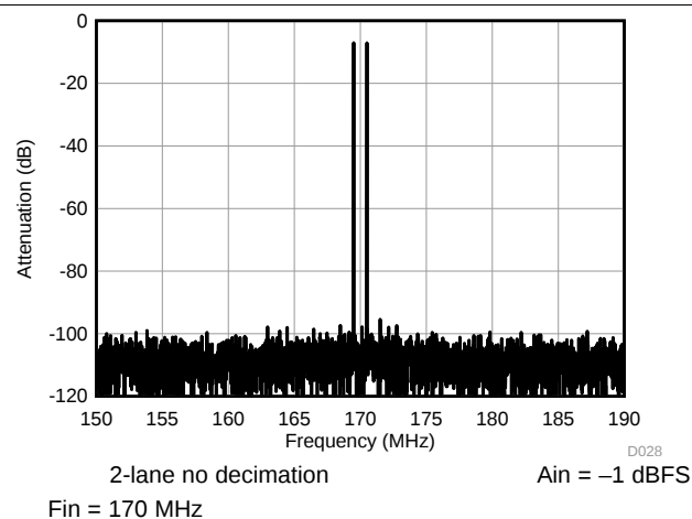
图 32. 2-Tone FFT
