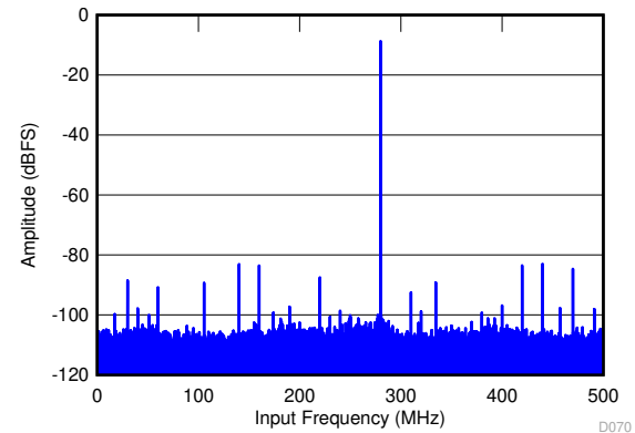
图 7-10. FFT for 720-MHz Input Signal at - 6 dBFS
