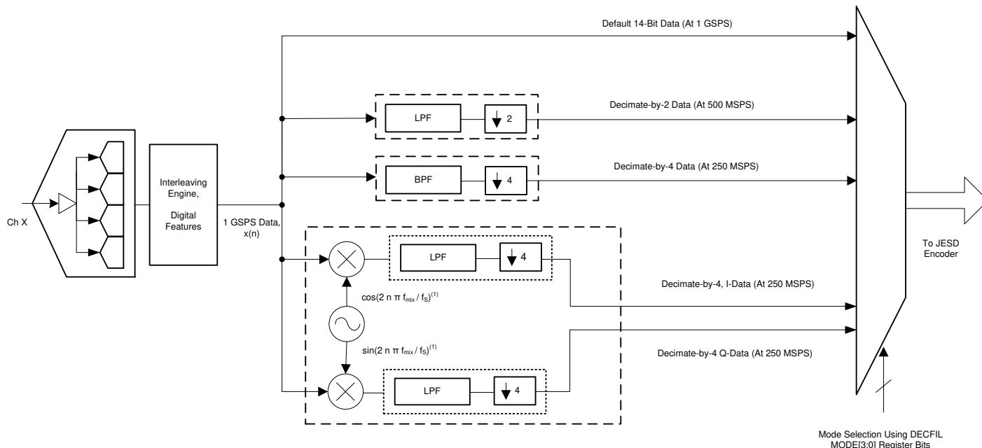
图 8-3. DDC Block
