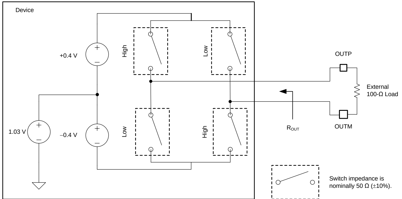
图 71. LVDS Output Circuit
