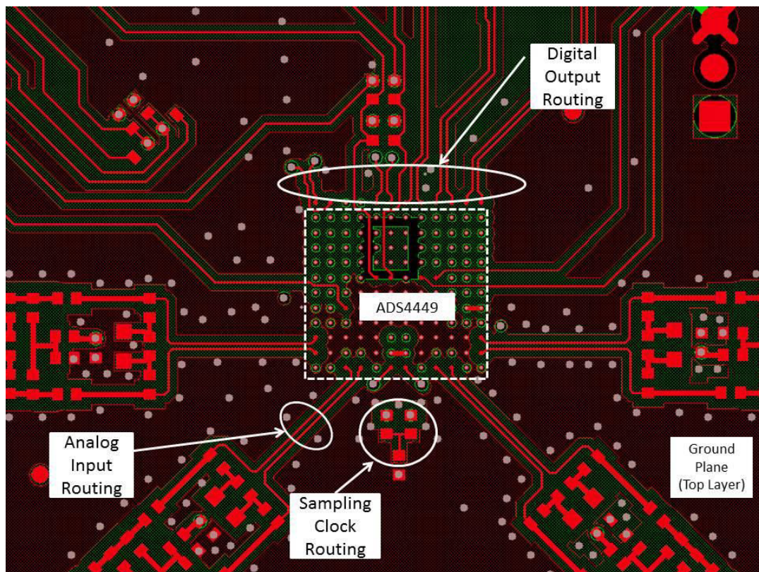
图 11-1. ADS4449 Layout
