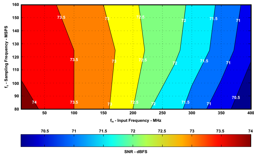
图 44. 0-dB Gain
