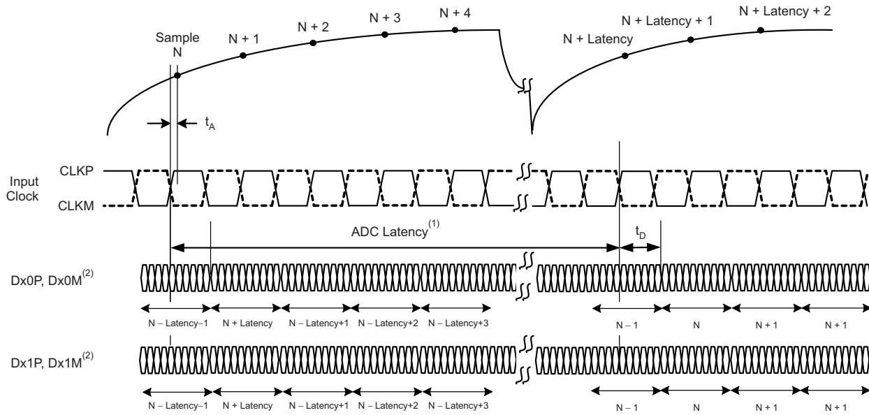
图 3. ADC Latency
