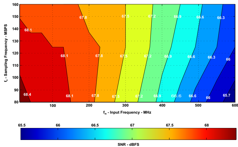
图 45. 6-dB Gain
