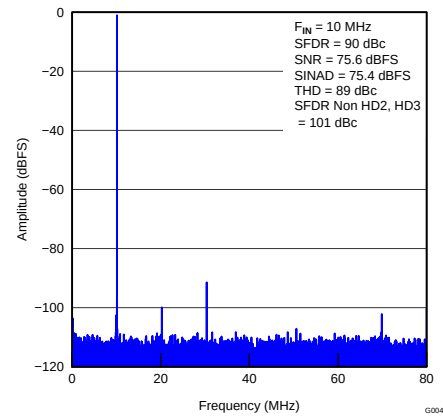
图 9. FFT for 10-MHz Input Signal ( 2.5\text{-V}_{\text{PP}} Full-Scale)
