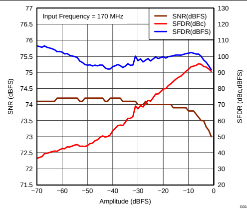
图 23. Performance vs Input Amplitude (170 MHz)
