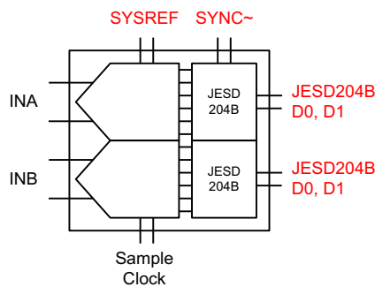
图 46. JESD204B Interface
