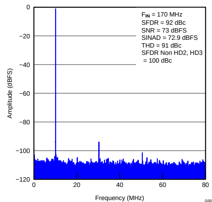
160 MSPS 时采样的 170MHz 输入信号的快速傅立叶变换 (FFT)
