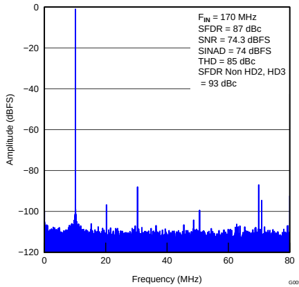
图 10. FFT for 170-MHz Input Signal ( 2.5\text{-V}_{\text{PP}} Full-Scale)
