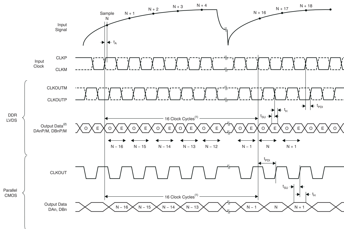
图 7-1. CMOS Interface Timing Diagram
