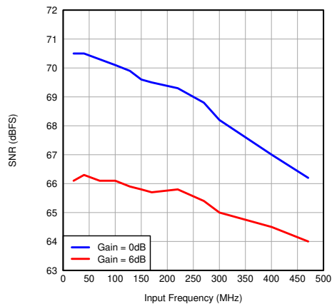
图 7-92. SNR vs Input Frequency
