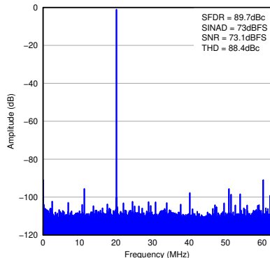
图 7-28. FFT for 20-MHz Input Signal
