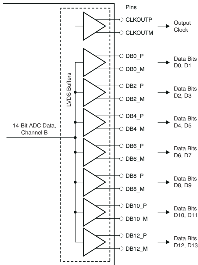
图 8-20. LVDS Interface
