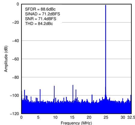
图 7-49. FFT for 170-MHz Input Signal
