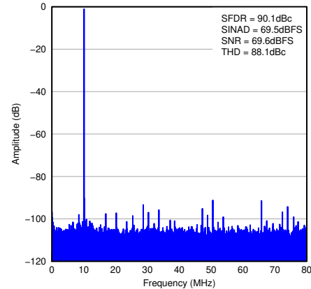
图 7-71. FFT for 170-MHz Input Signal
