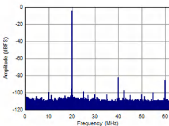
图 9-4. FFT for 270-MHz Input Signal
