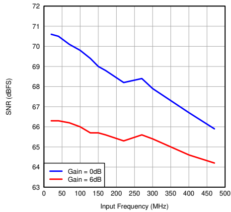
图 7-76. SNR vs Input Frequency (CMOS)
