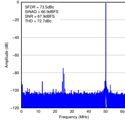
图 7-89. FFT for 300-MHz Input Signal
