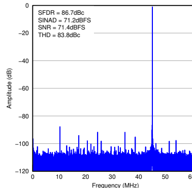
图 7-29. FFT for 170-MHz Input Signal
