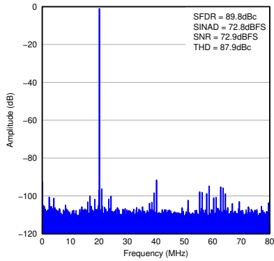
图 7-6. FFT for 20-MHz Input Signal
