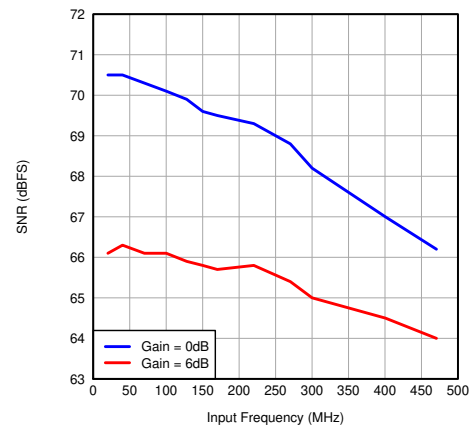
图 7-75. SNR vs Input Frequency
