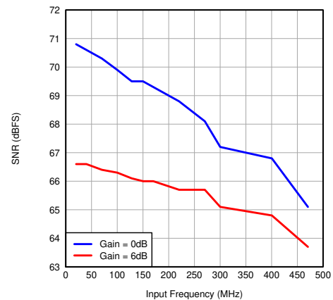
图 7-93. SNR vs Input Frequency (CMOS)
