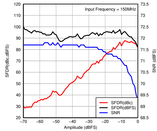
图 7-115. Performance vs Input Amplitude
