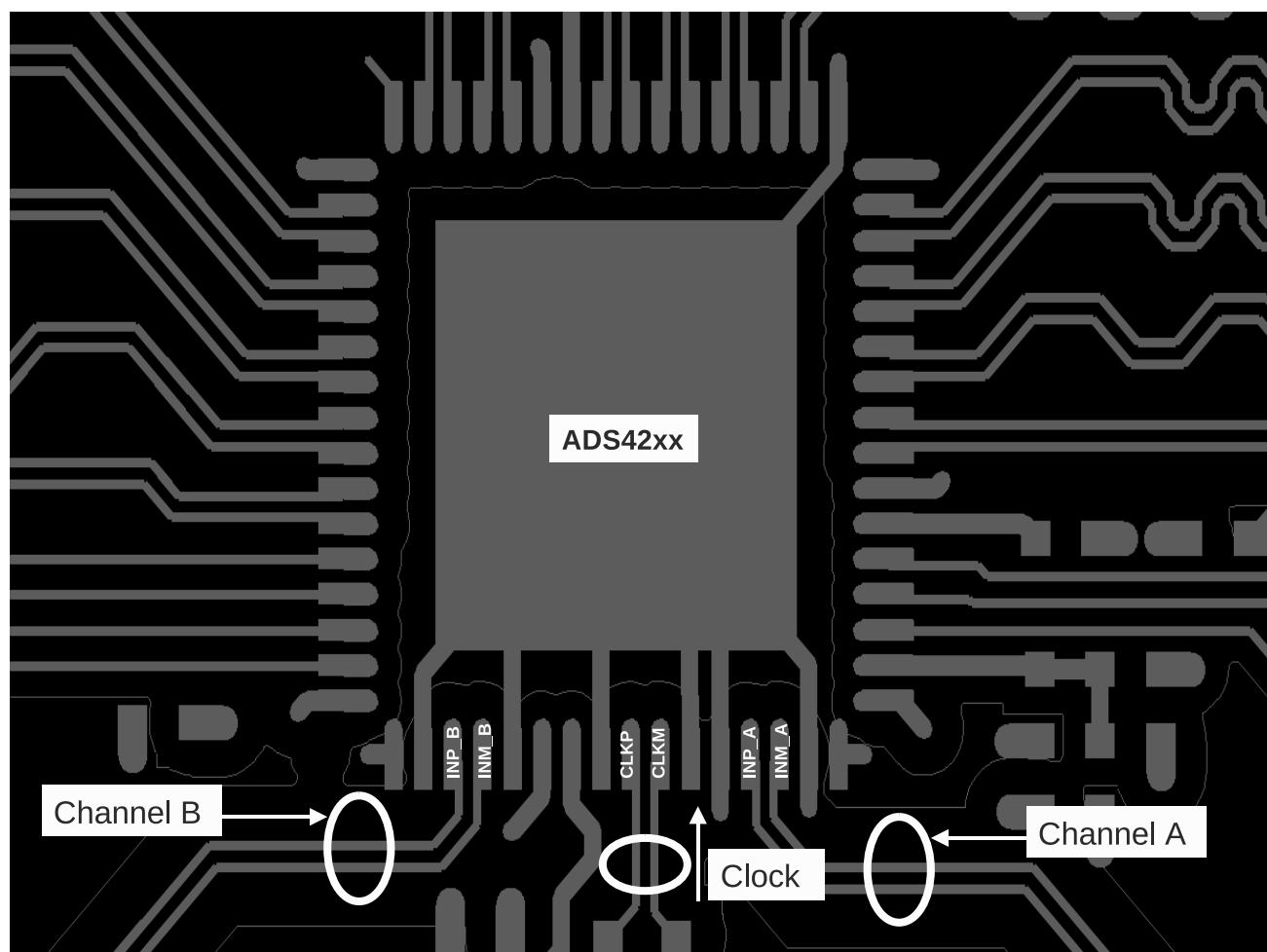
图 9-5. ADS42xx EVM PCB Layout
