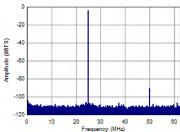
图 9-3. FFT for 100-MHz Input Signal
