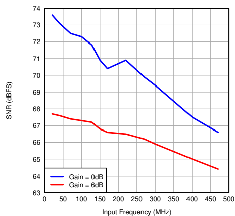
图 7-54. SNR vs Input Frequency
