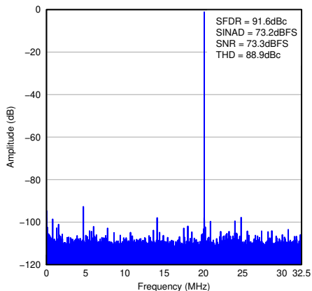
图 7-48. FFT for 20-MHz Input Signal
