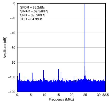
图 7-105. FFT for 170-MHz Input Signal
