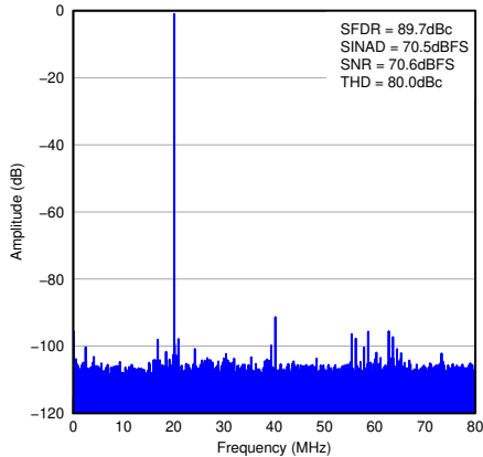
图 7-70. FFT for 20-MHz Input Signal
