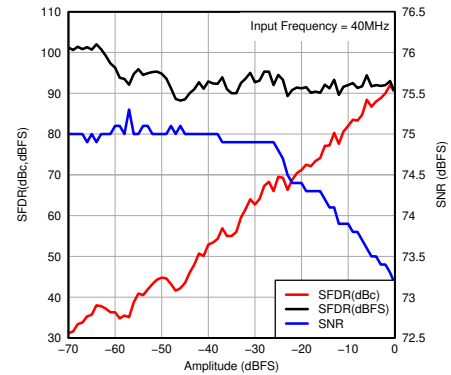
图 7-37. Performance vs Input Amplitude
