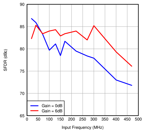
图 7-74. SFDR vs Input Frequency
