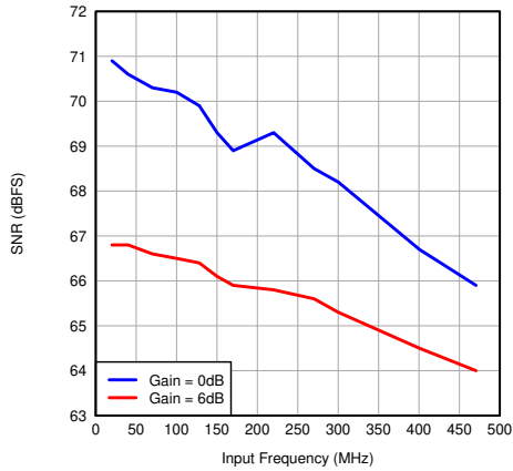
图 7-110. SNR vs Input Frequency
