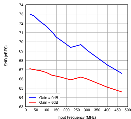
图 7-13. SNR vs Input Frequency (CMOS)
