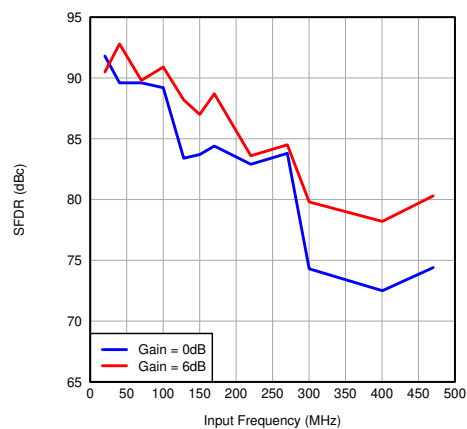
图 7-53. SFDR vs Input Frequency
