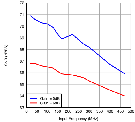
图 7-111. SNR vs Input Frequency (CMOS)
