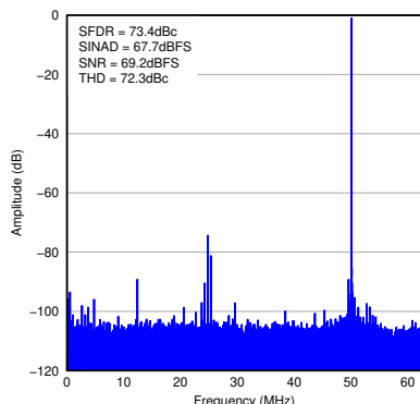
图 7-30. FFT for 300-MHz Input Signal
