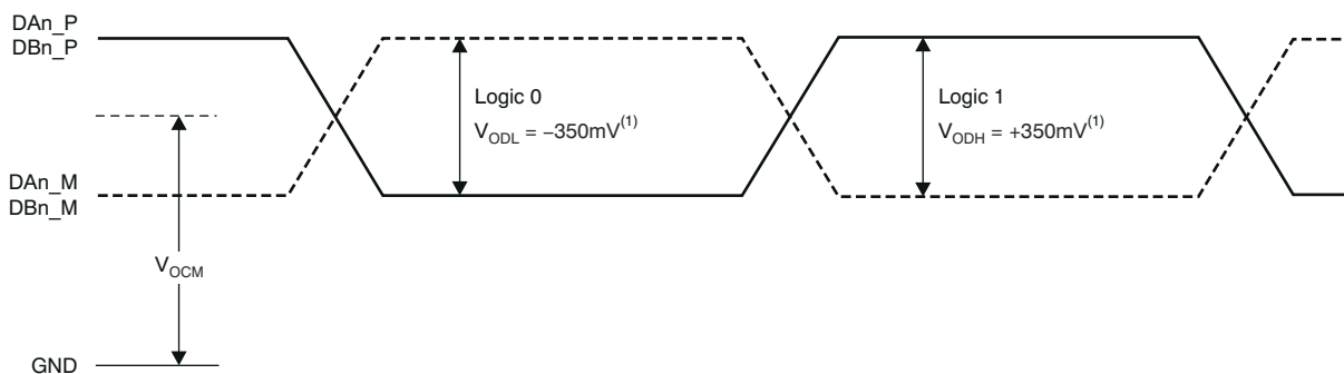
图 7-5. LVDS Output Voltage Levels
