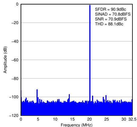
图 7-104. FFT for 20-MHz Input Signal
