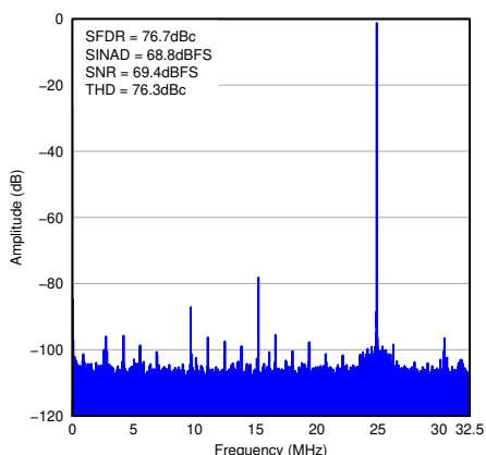
图 7-50. FFT for 300-MHz Input Signal
