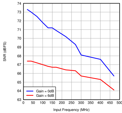
图 7-34. SNR vs Input Frequency (CMOS)
