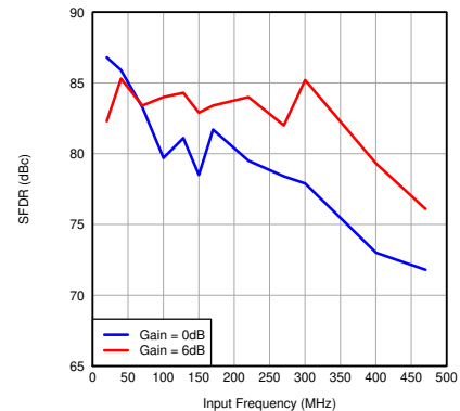
图 7-11. SFDR vs Input Frequency
