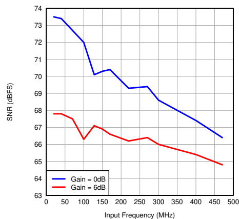
图 7-55. SNR vs Input Frequency (CMOS)
