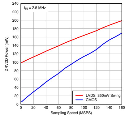
图 7-127. Digital Power LVDS CMOS
