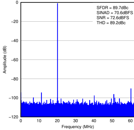
图 7-88. FFT for 20-MHz Input Signal
