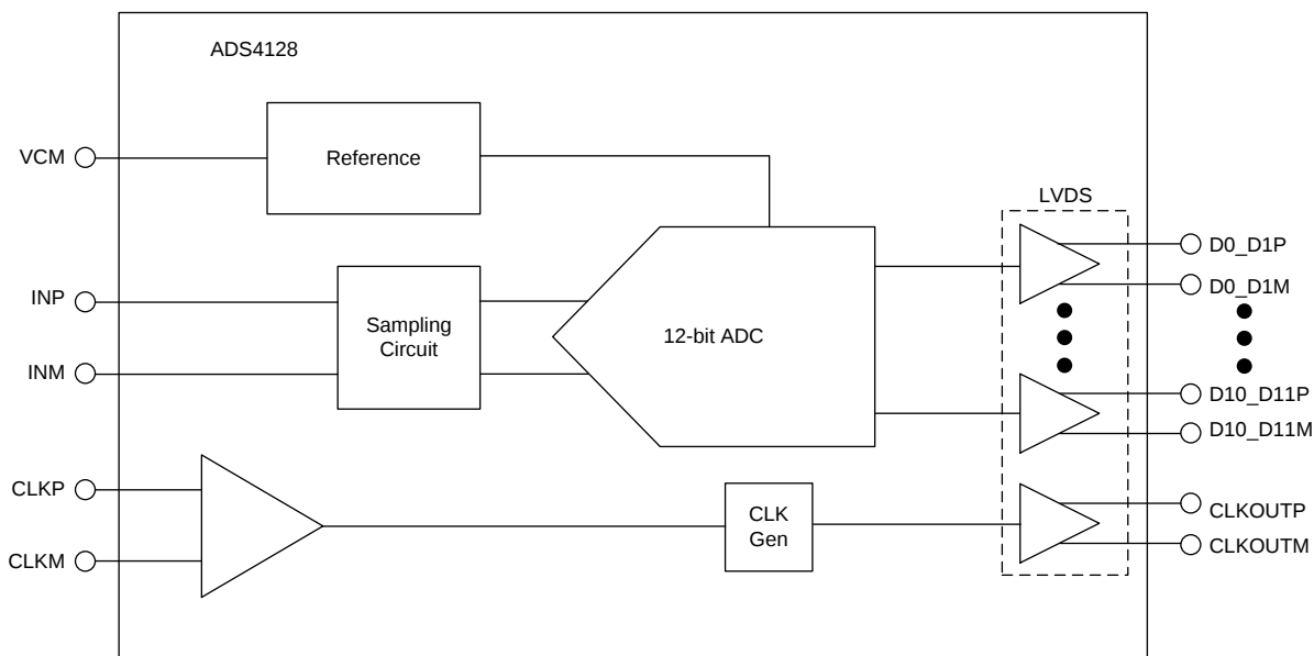
ADS4128 框图
