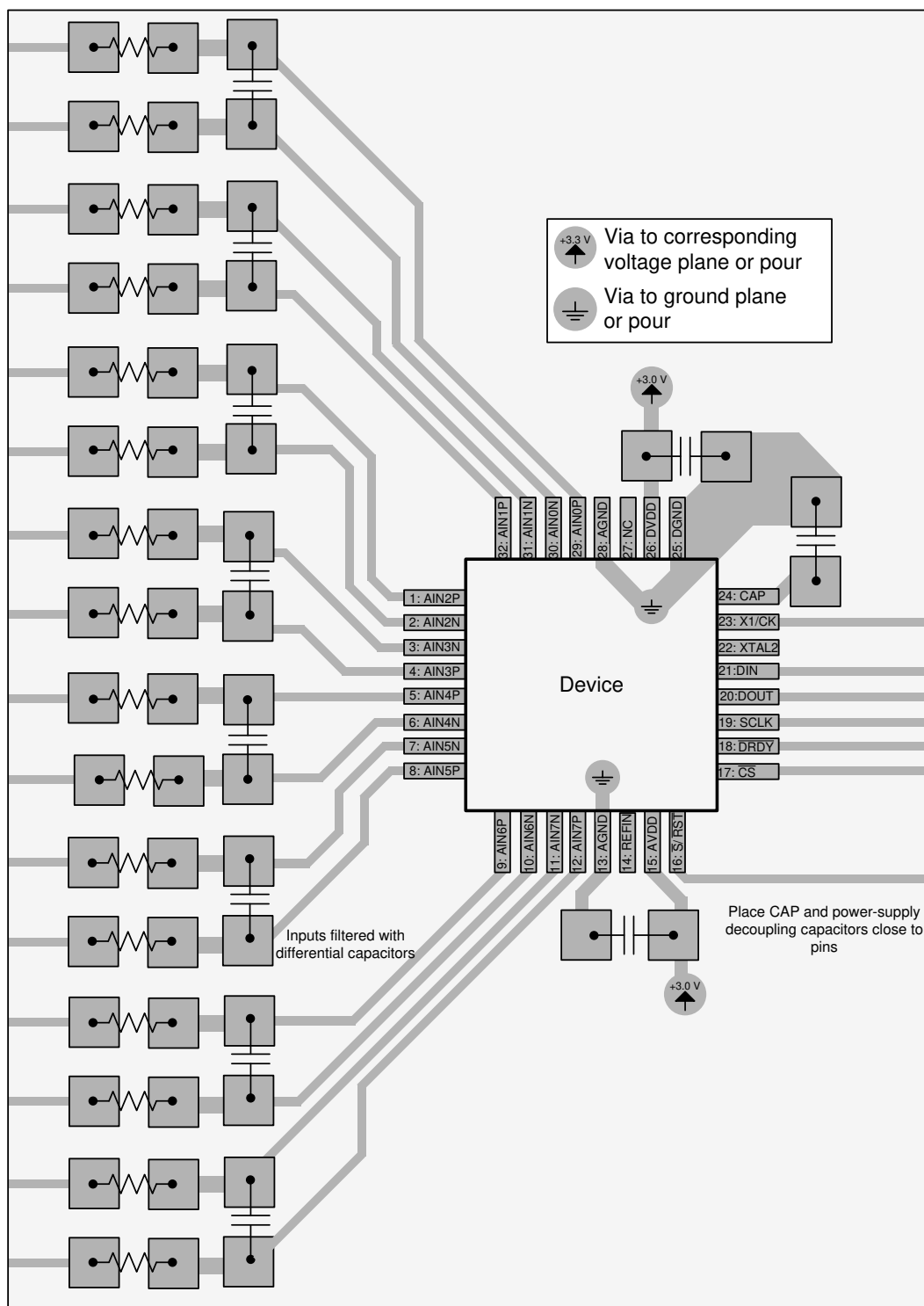
图 9-6. Layout Example
