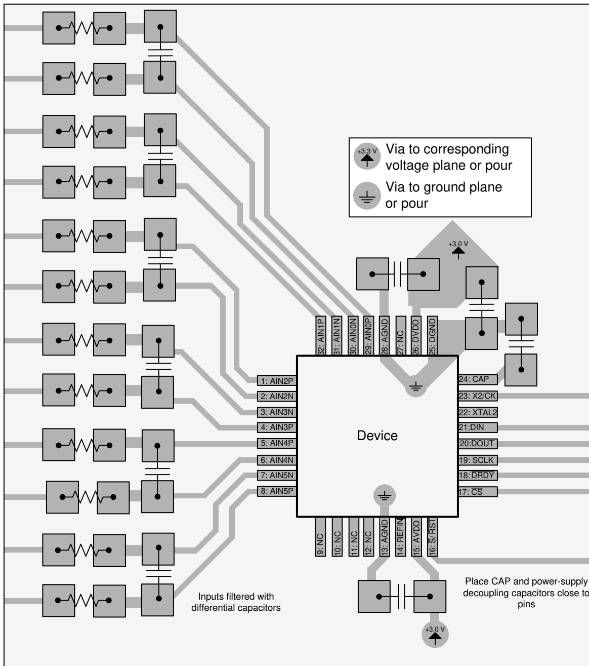
图 9-6. Layout Example
