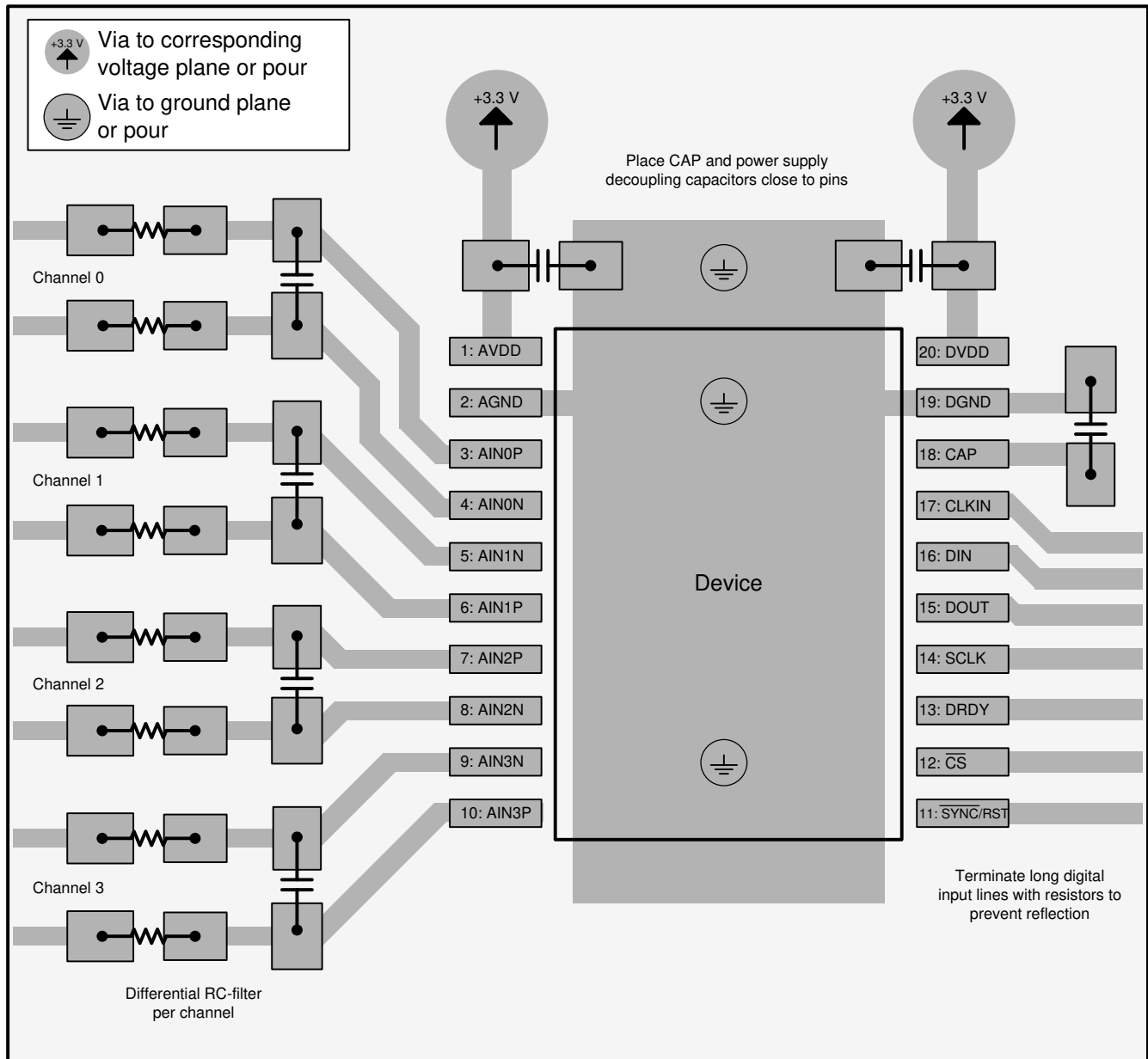
图 9-6. Layout Example
