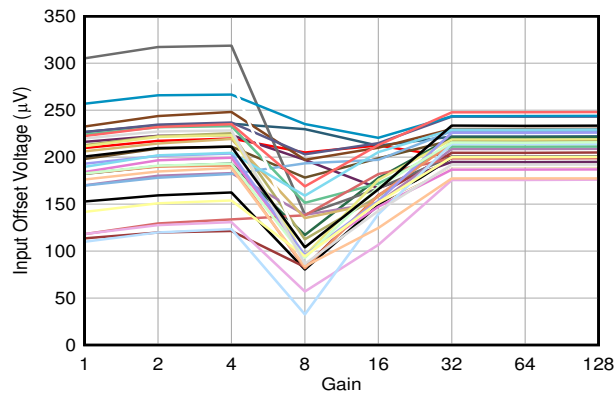
图 6-7. Input Offset Voltage vs Gain
