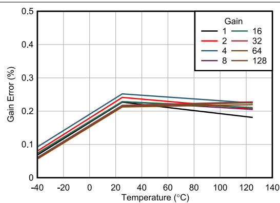
图 6-9. Gain Error vs Temperature
