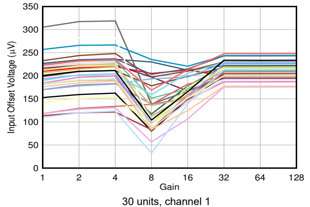
图 6-7. Input Offset Voltage vs Gain
