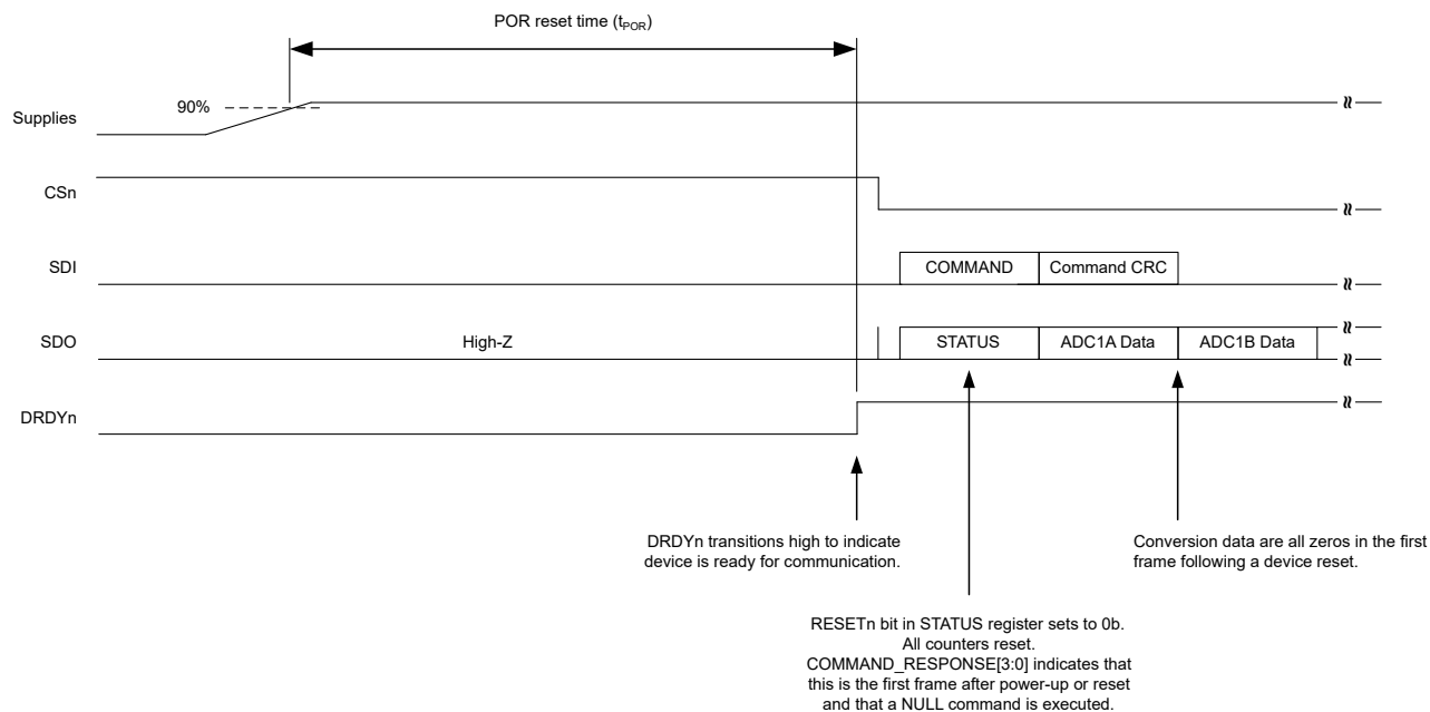
图 7-26. POR 后的 DRDYn 引脚行为
