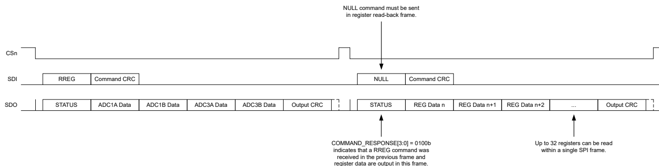
图 7-37. RREG 命令帧
