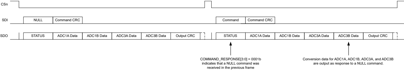
图 7-31. NULL 命令帧
