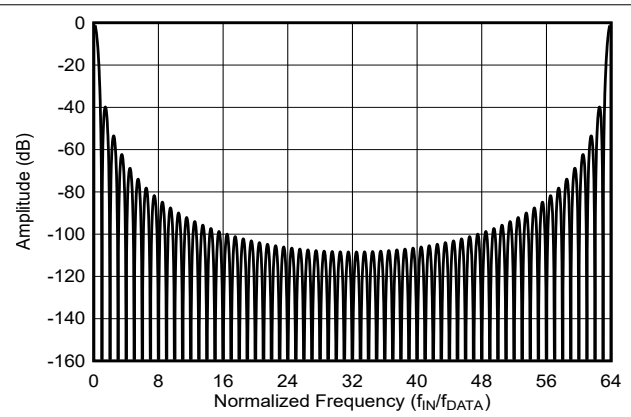
图 7-4. f_{MOD} 的 Sinc3 滤波器频率响应 (OSR = 64)
