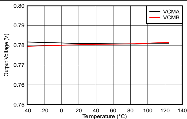
图 5-38. VCM y 输出电压与温度间的关系
