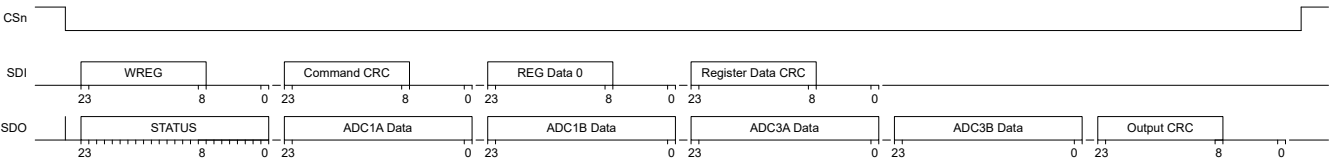
图 7-29. 位对齐、24 位字大小、WREG 命令
