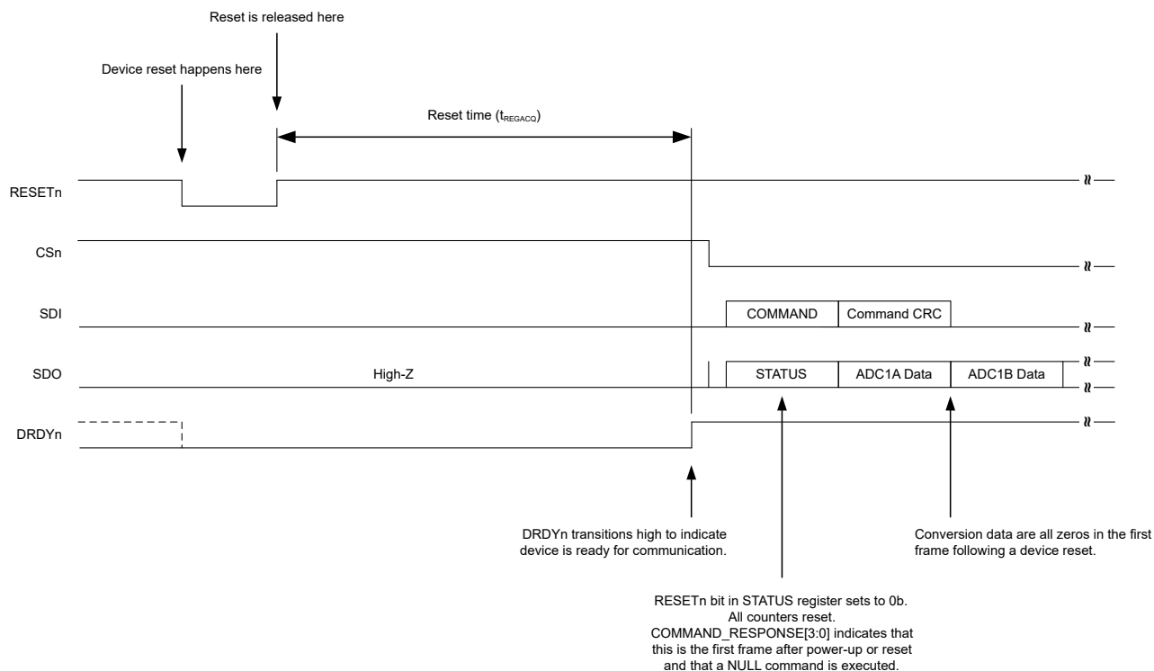
图 7-27. 器件复位后的 DRDYn 引脚行为
