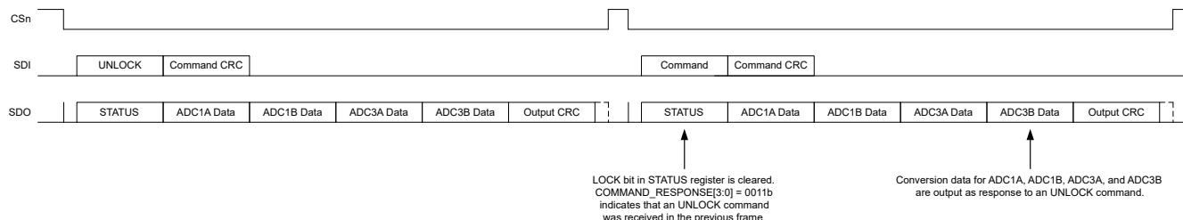
图 7-34. UNLOCK 命令帧
