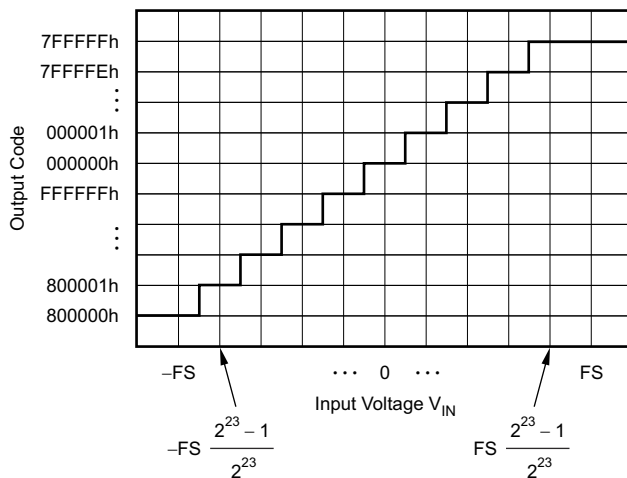
图 7-6. 代码转换图 (24 位转换数据)
