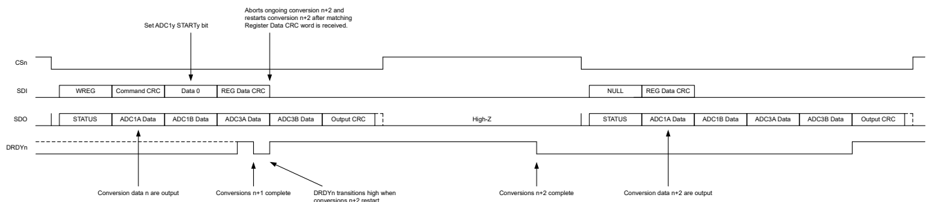
图 7-45. DRDYn 引脚行为：设置 STARTy 位并在新的转换完成时读取转换数据
