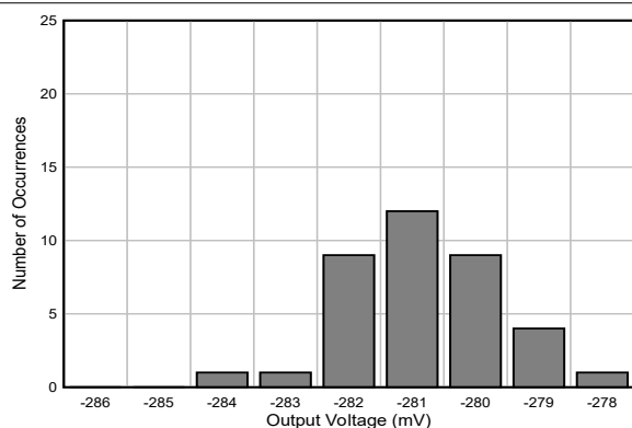
图 5-28. 测试 DACy 输出电压直方图
