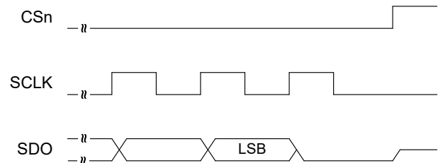
图 7-25. 有额外 SCLK 脉冲时的 SDO 行为
