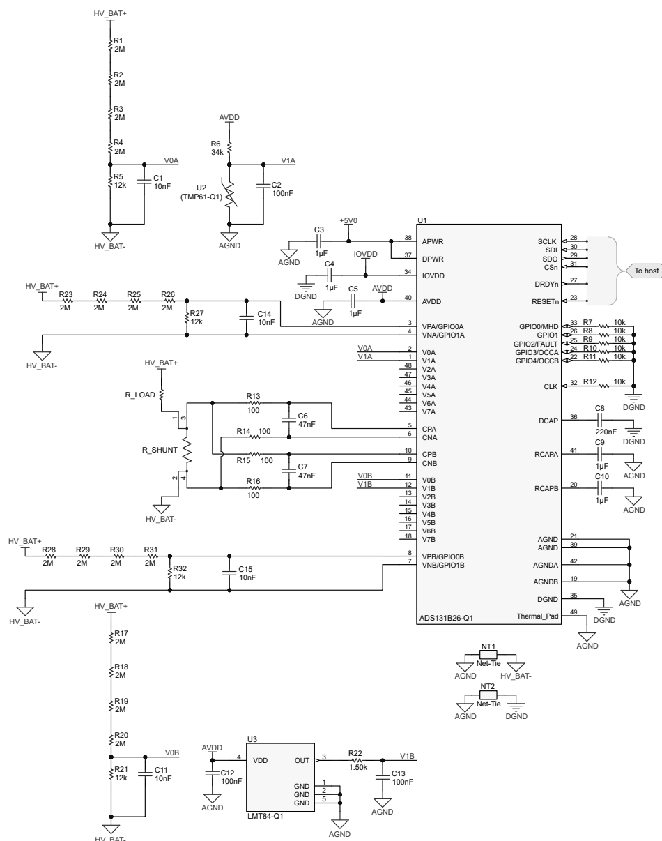
图 9-1. 典型电池管理系统应用中的 ADS131B26-Q1
