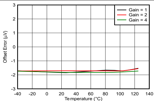
图 5-15. ADC3y 失调电压误差与温度间的关系
