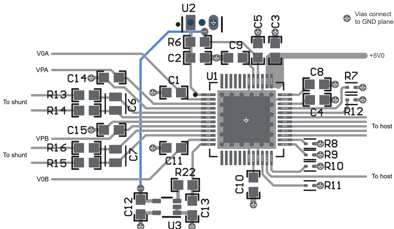
图 9-8. 布局示例
