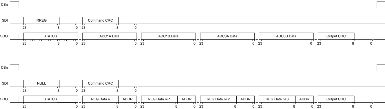
图 7-30. 位对齐、24 位字大小、RREG 命令
