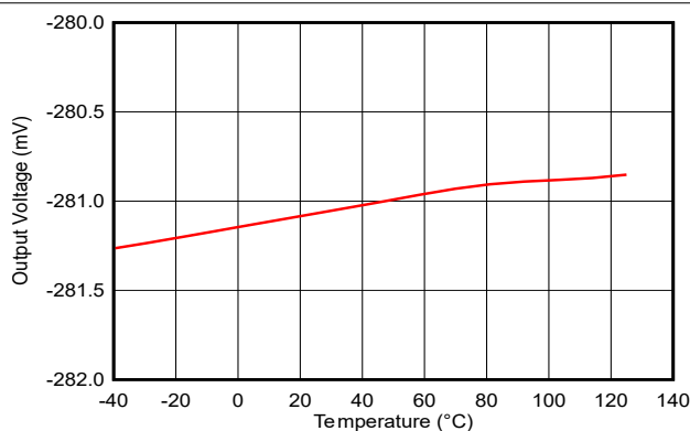
图 5-29. 测试 DACy 输出电压与温度间的关系
