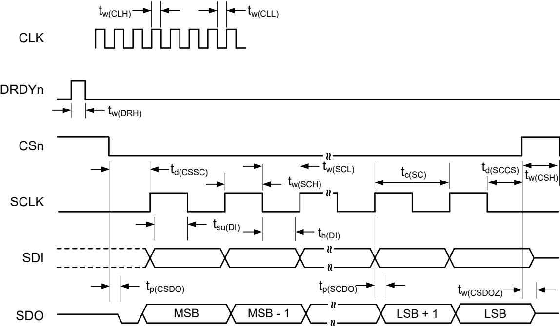
图 5-1. SPI 时序要求和开关特性
