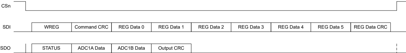
图 7-36. WREG 命令帧 ( 6 个寄存器 )
