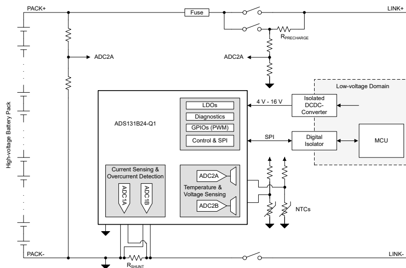
EV BMS 电池包监测系统方框图
