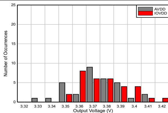
图 5-33. AVDD 和 IOVDD LDO 输出电压直方图
