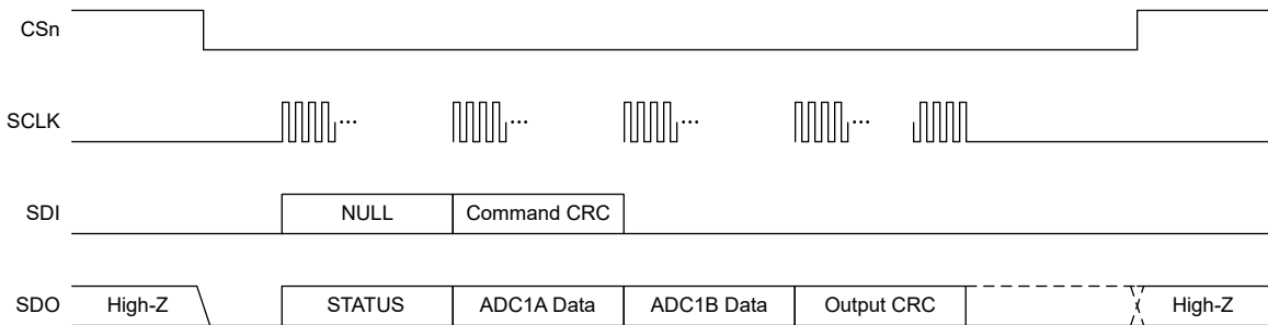
图 7-28. 典型通信帧
