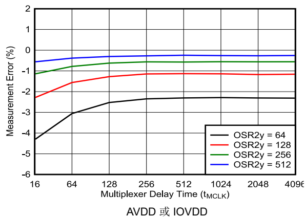
图 5-27. ADC2y 电源电压回馈测量精度
