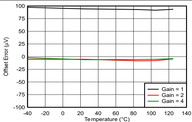
图 5-9. ADC2y 失调电压误差与温度间的关系
