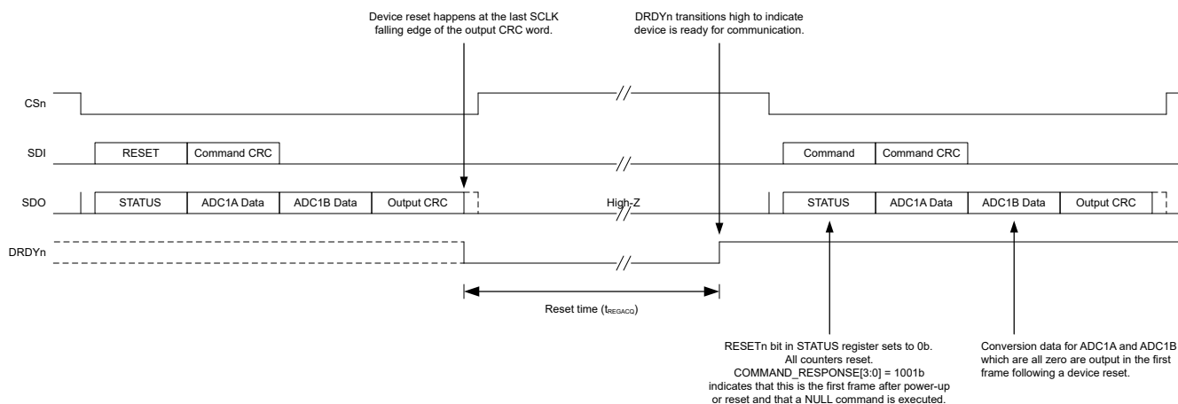
图 7-32. RESET 命令帧
