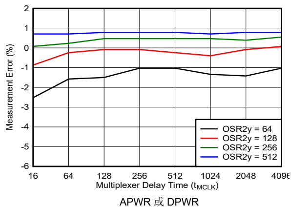
图 5-26. ADC2y 电源电压回馈测量精度
