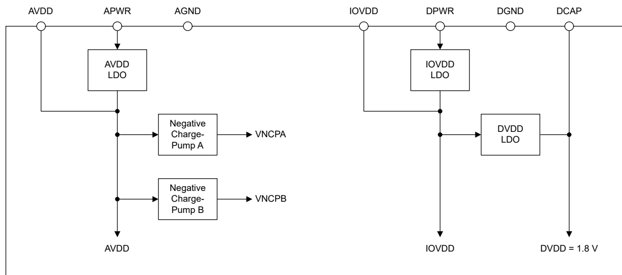
图 9-4. 电源架构
