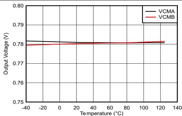
图 5-32. VCM y 输出电压与温度间的关系
