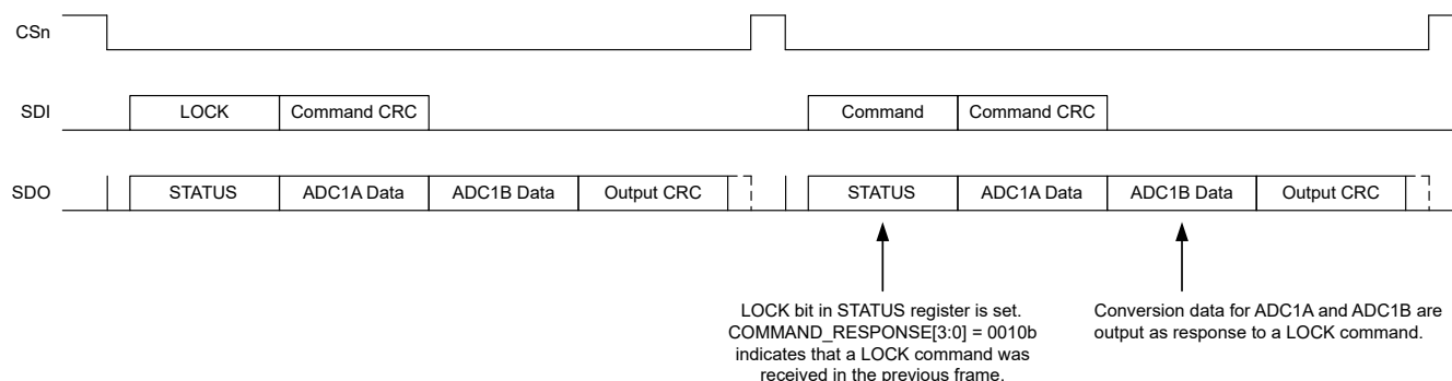
图 7-33. LOCK 命令帧
