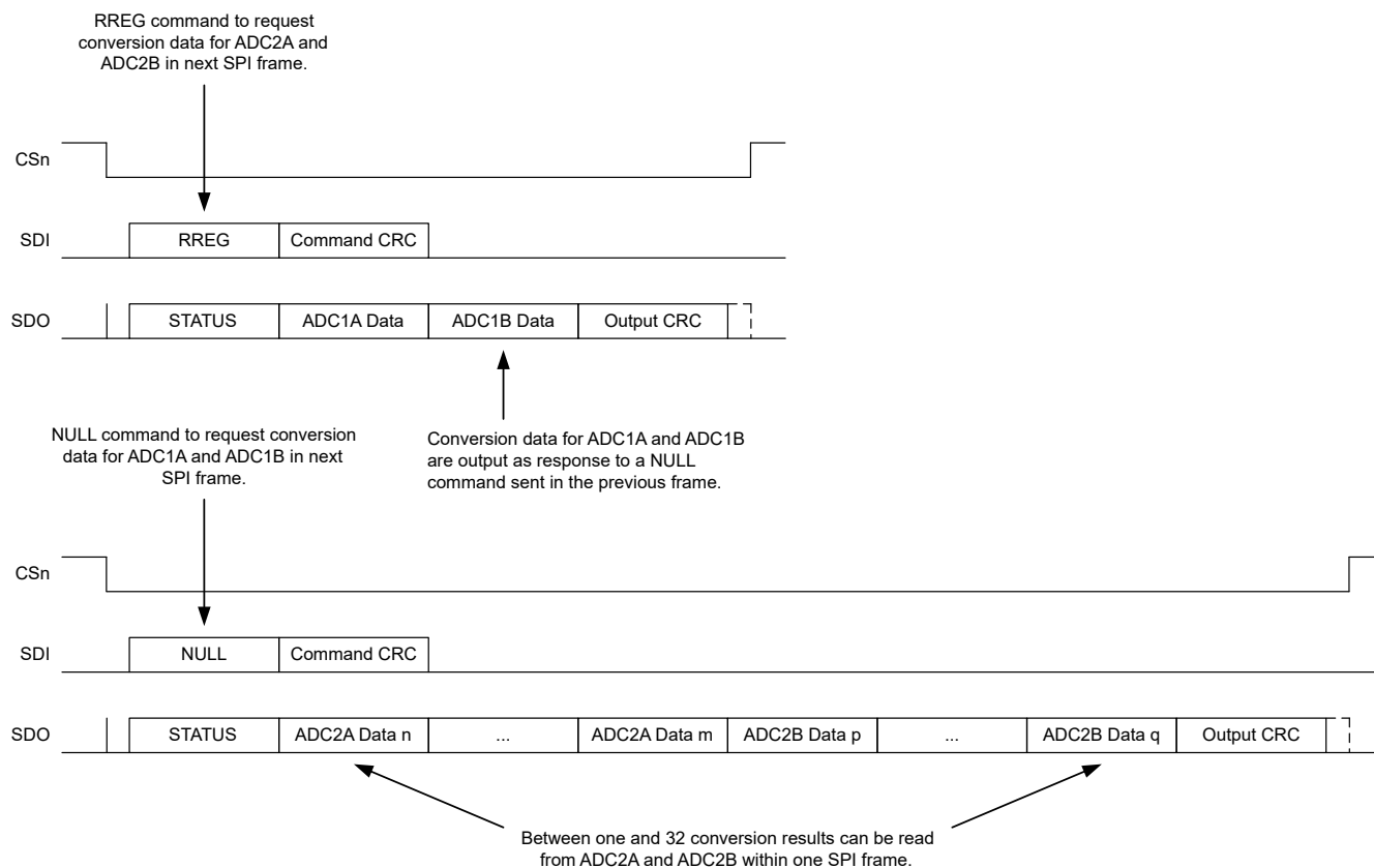
图 7-38. 从两个 SPI 帧内的 ADC1A、ADC1B、ADC2A 和 ADC2B 读取转换数据
