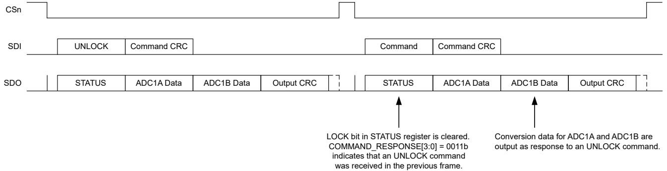
图 7-34. UNLOCK 命令帧
