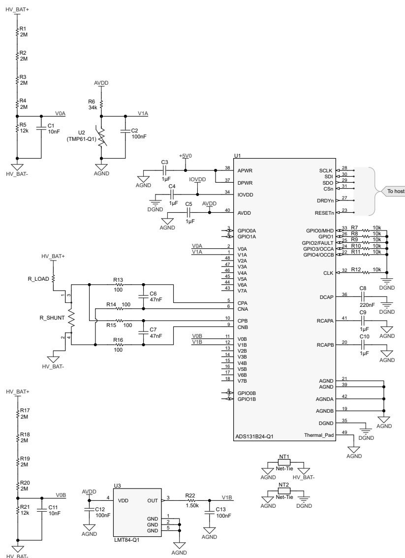
图 9-1. 典型电池管理系统应用中的 ADS131B24-Q1
