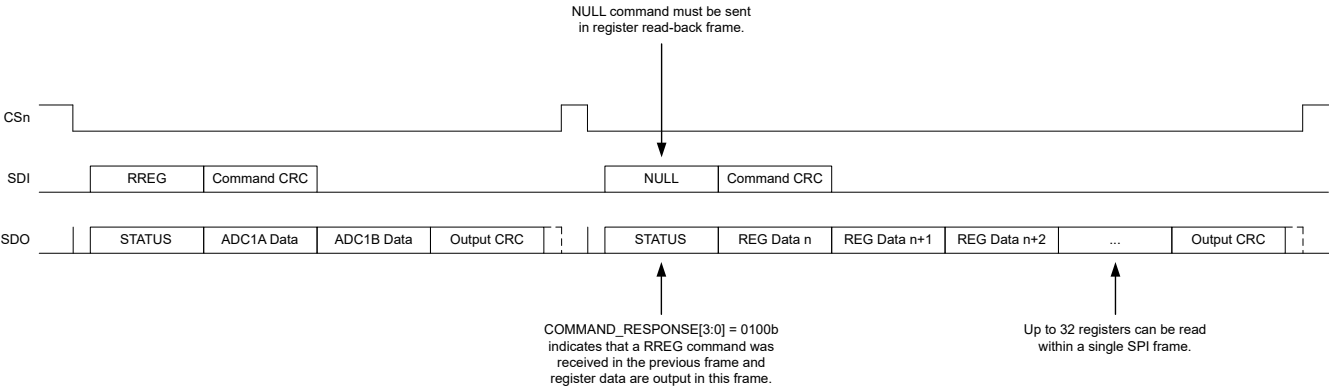
图 7-37. RREG 命令帧
