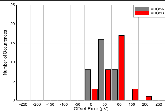
图 5-8. ADC2y 失调电压误差直方图
