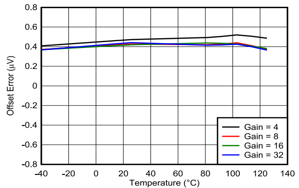
图 5-3. ADC1y 失调电压误差与温度间的关系
