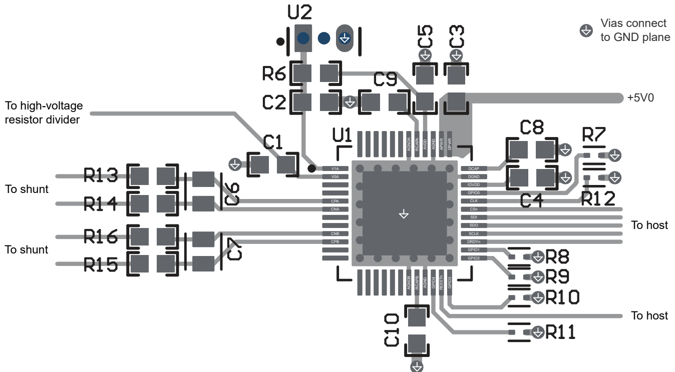
图 9-8. 布局示例
