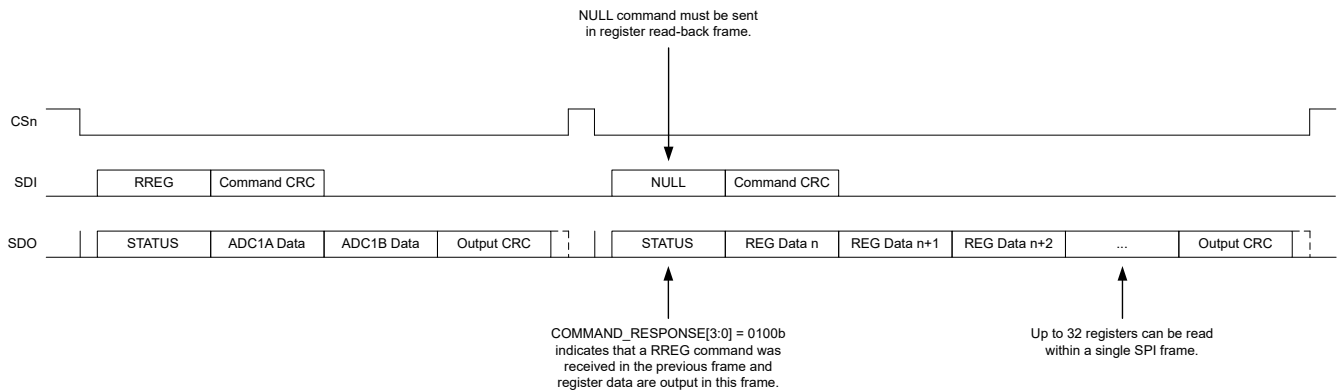
图 7-37. RREG 命令帧
