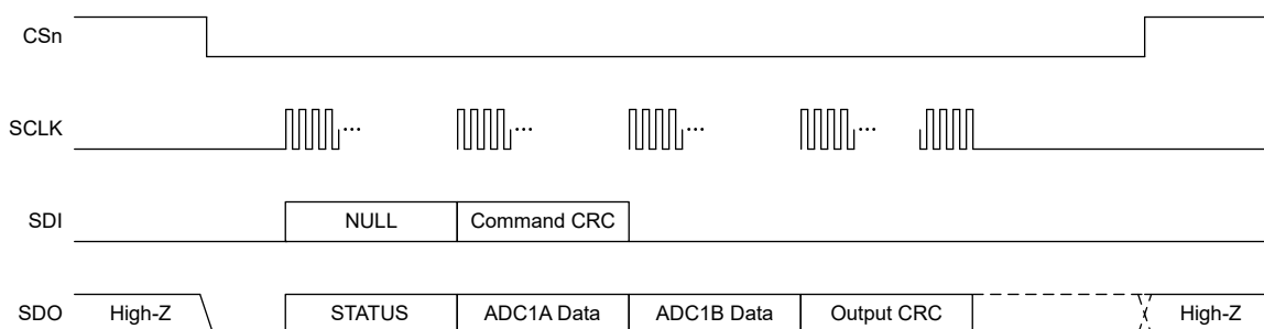
图 7-28. 典型通信帧
