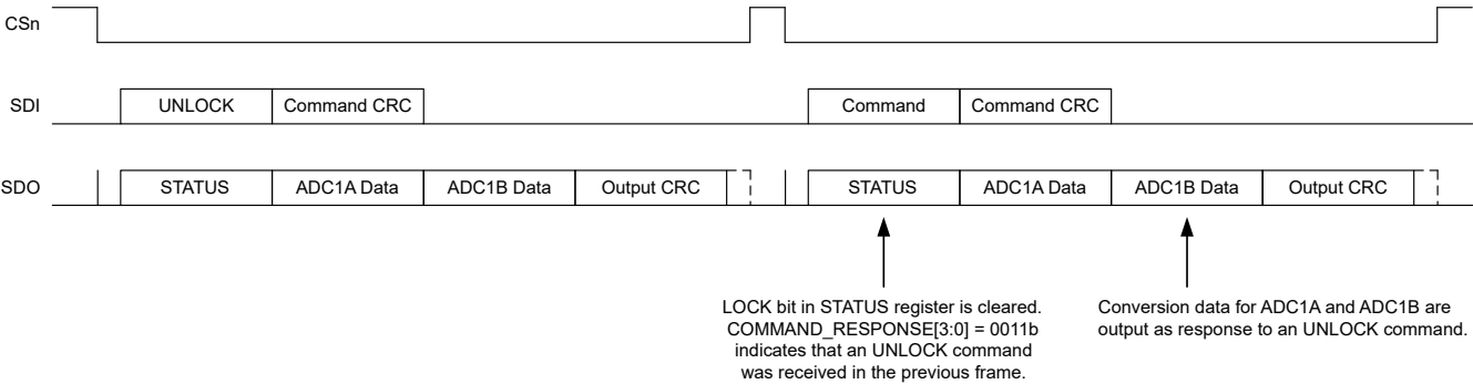
图 7-34. UNLOCK 命令帧
