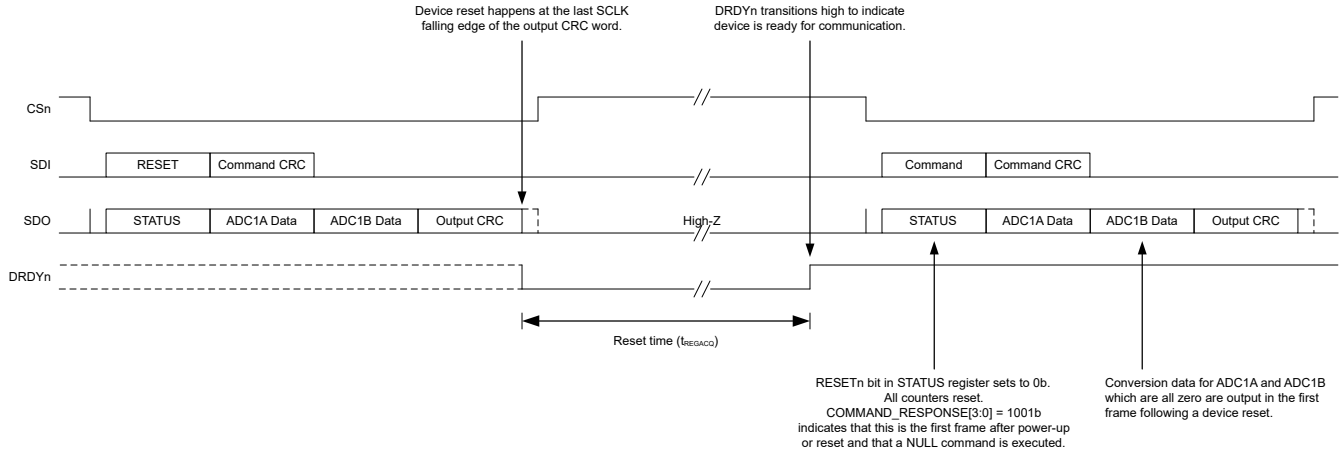
图 7-32. RESET 命令帧
