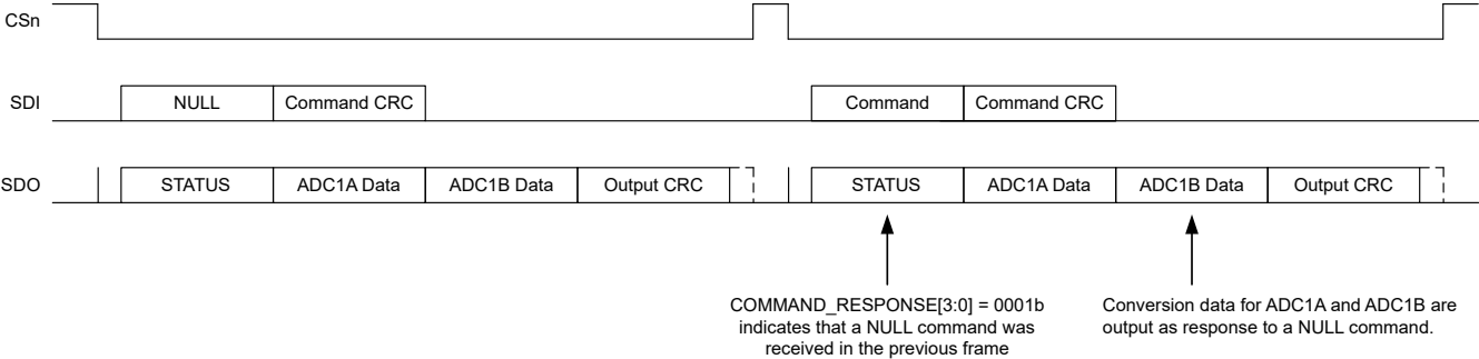
图 7-31. NULL 命令帧
