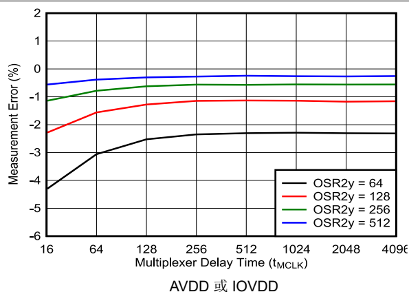
图 5-27. ADC2A 电源电压回读测量精度
