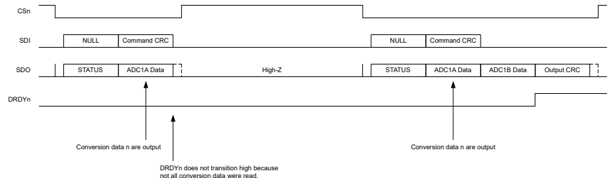
图 7-41. DRDYn 引脚行为：转换数据的未完成读取后跟相同转换数据的完全读取
