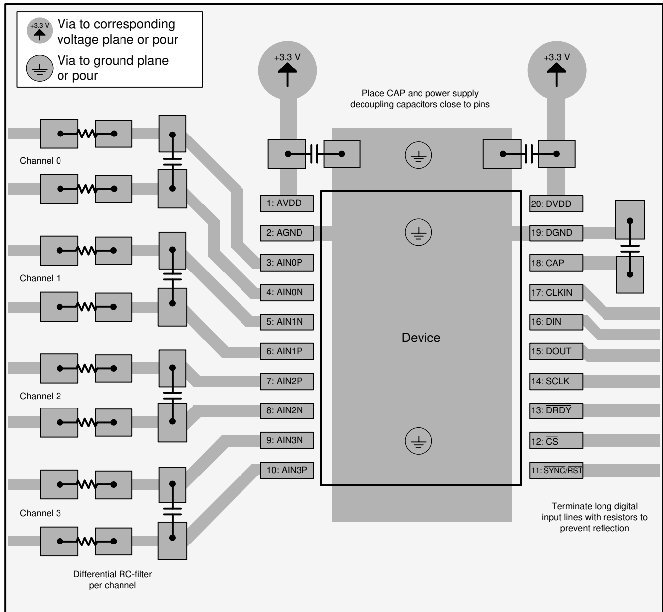
图 11-1. Layout Example
