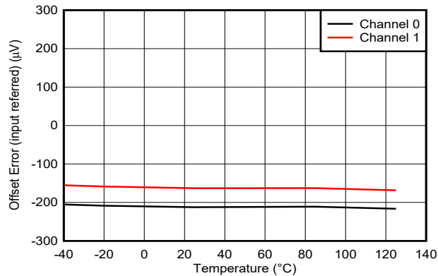
图 6-4. Offset Error vs Temperature
