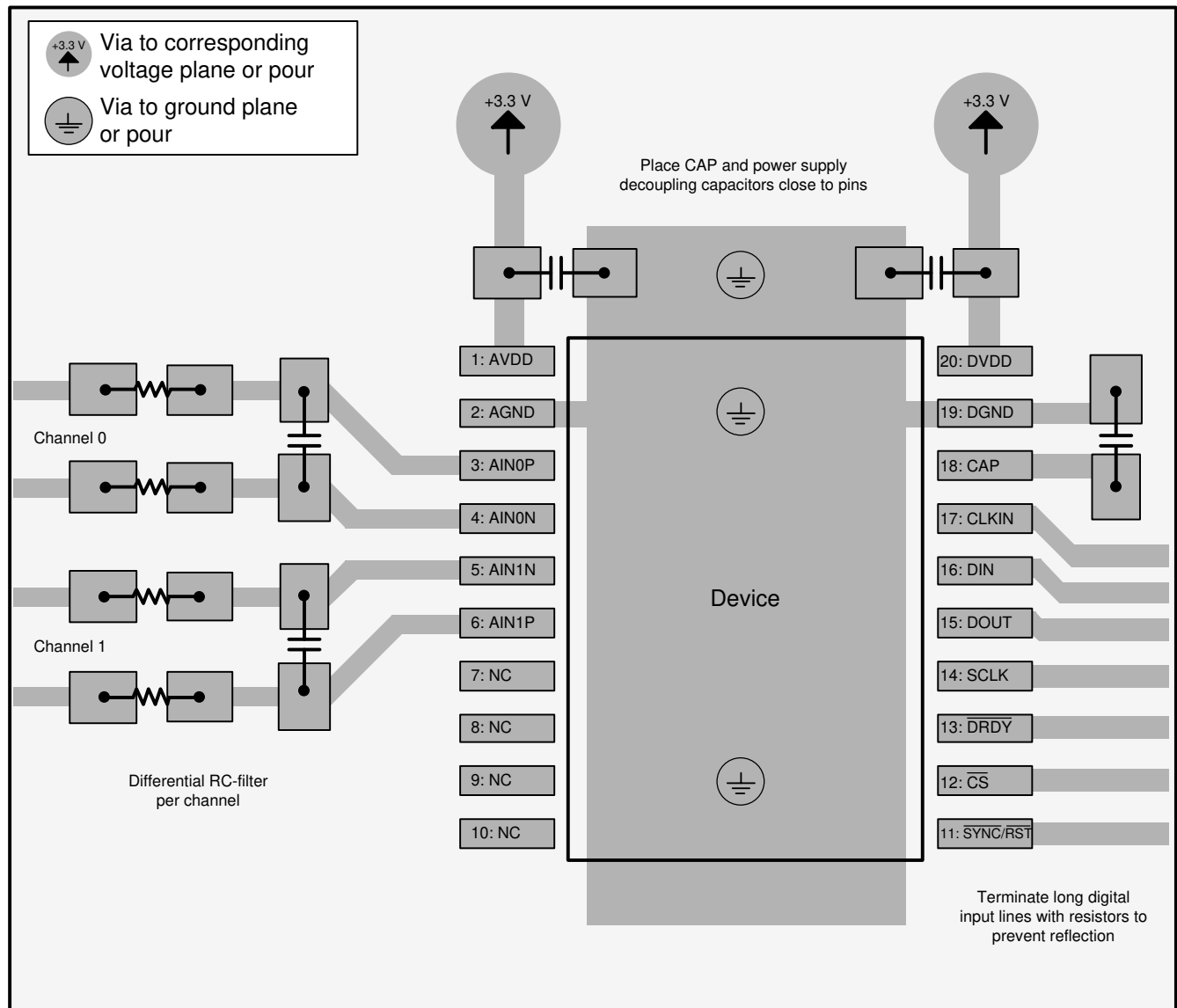
图 11-1. Layout Example
