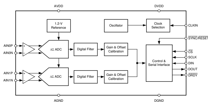
简化方框图
