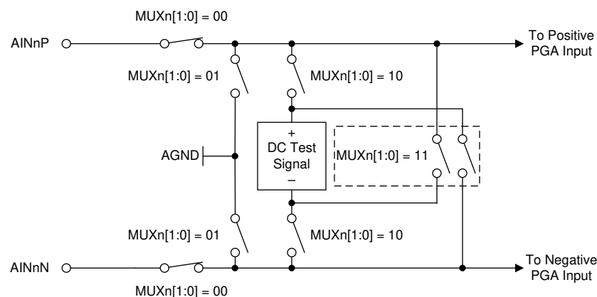
图 8-2. Input Multiplexer
