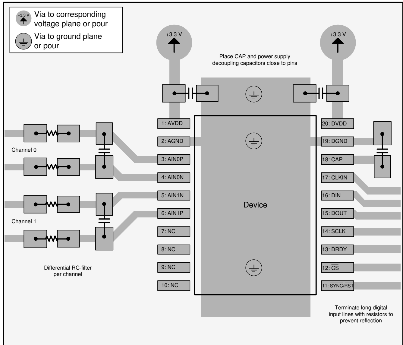
图 11-1. Layout Example
