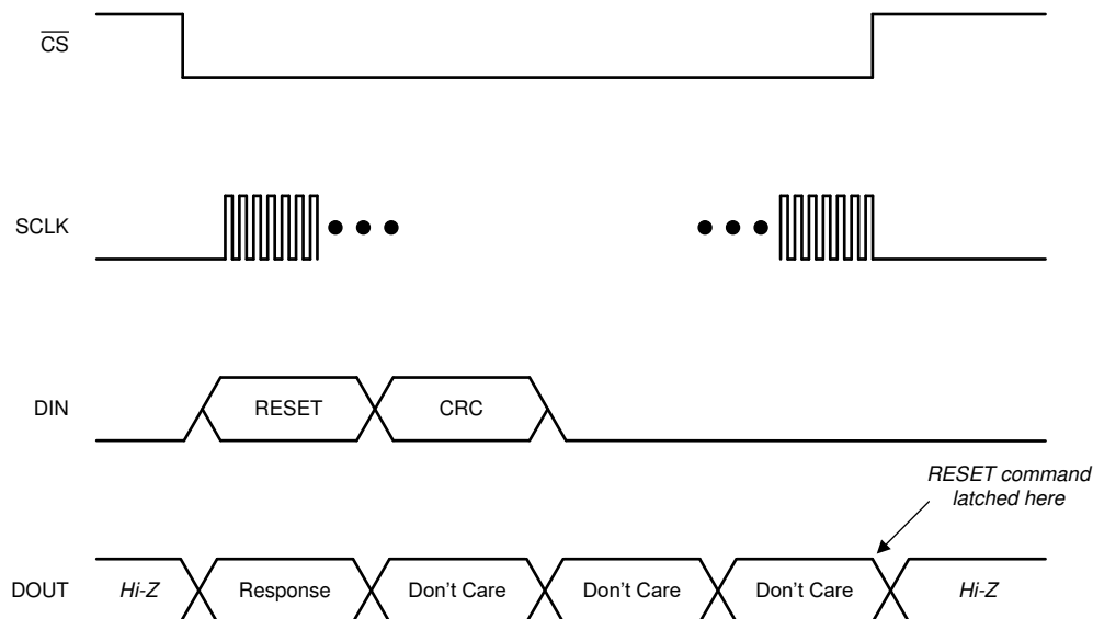
图 8-18. RESET Command Frame
