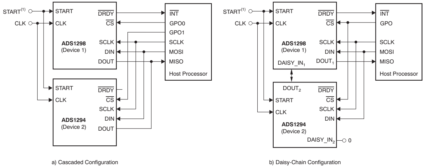
Figure 66. 多器件配置
