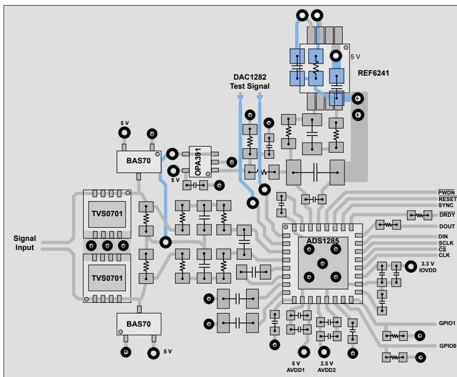
图 9-3. Example Layout
