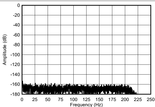
图 6-9. High-Power Mode FFT Spectrum
