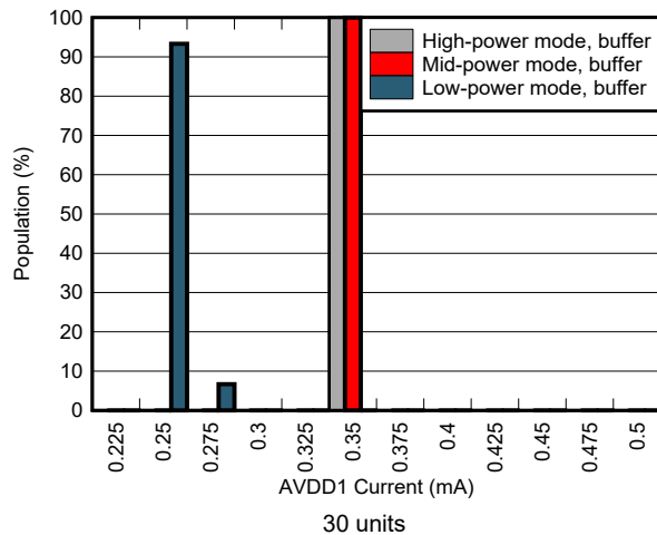
图 6-61. AVDD1 Current Distribution
