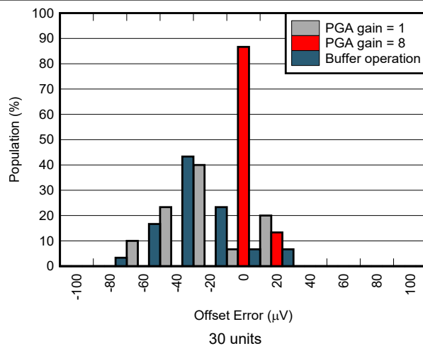
图 6-39. Offset Error Distribution
