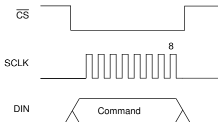
图 8-23. Single Byte Command Format
