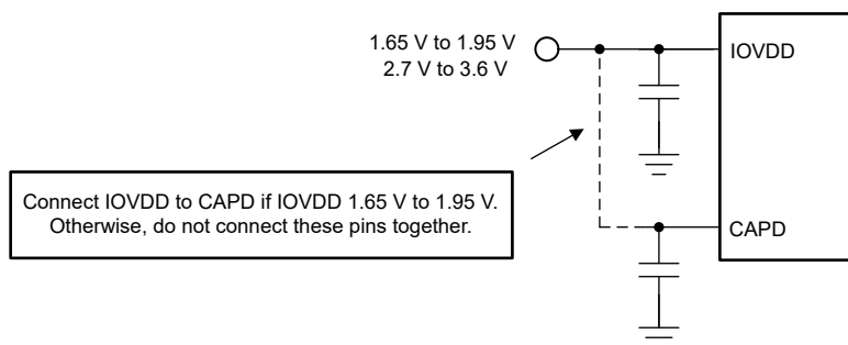
图 8-9. IOVDD Power-Supply Connection
