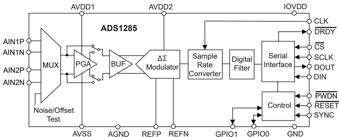
功能方框图
