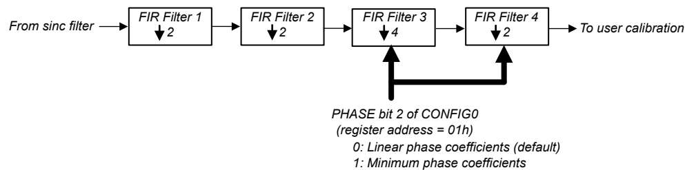
图 8-14. FIR Filter
