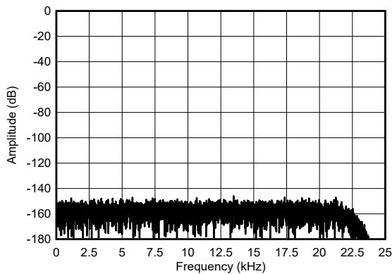
V_{REF} = 2.5V ，宽带滤波器，2 倍范围 图 5-27. 低速模式，短接输入 FFT
