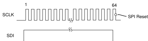
图 7-46. 3 线模式 SPI 复位模式
