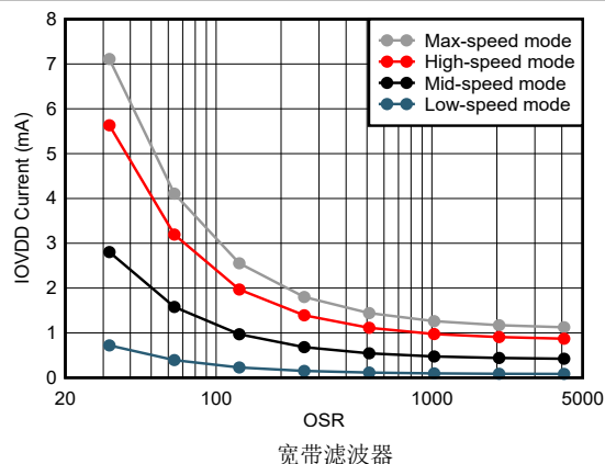
宽带滤波器 图 5-92. IOVDD 电流与过采样率间的关系
