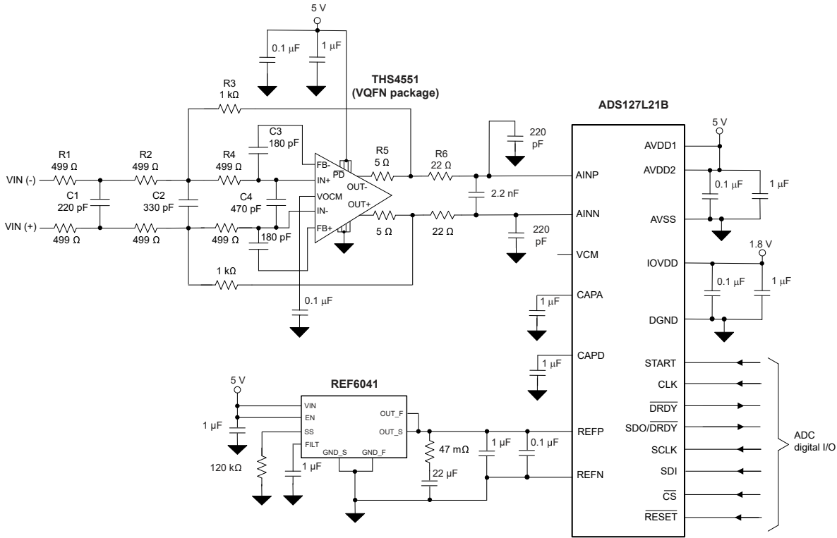
图 9-8. ADS127L21B 电路图
