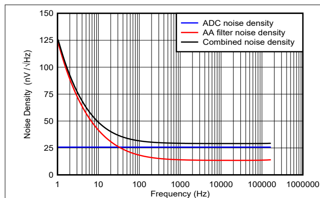
图 9-11. 噪声密度
