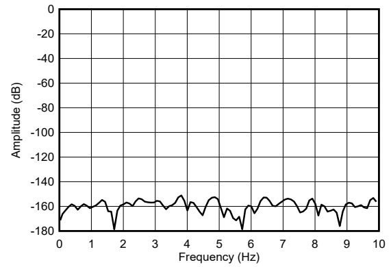
0Hz 至 10Hz 图 5-26. 低速模式，短接输入 FFT
