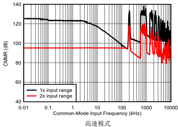
图 5-77. CMRR 与频率间的关系
