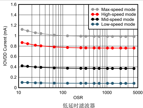
低延时滤波器 图 5-93. IOVDD 电流与过采样率间的关系
