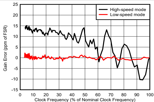
图 5-56. 增益误差与时钟频率间的关系
