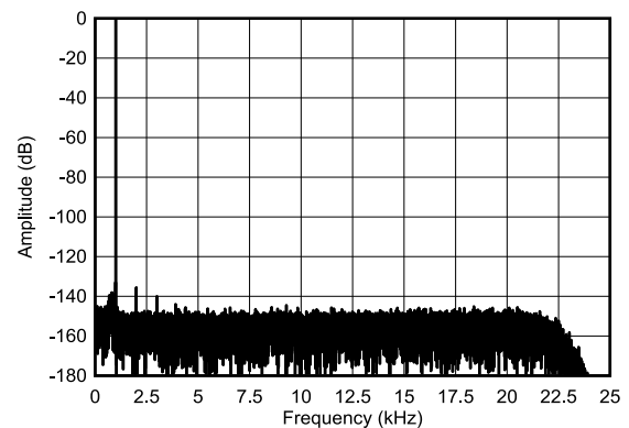
V_{IN} = -0.2dBFS ，1kHz，宽带滤波器 图 5-30. 低速模式，满量程 FFT
