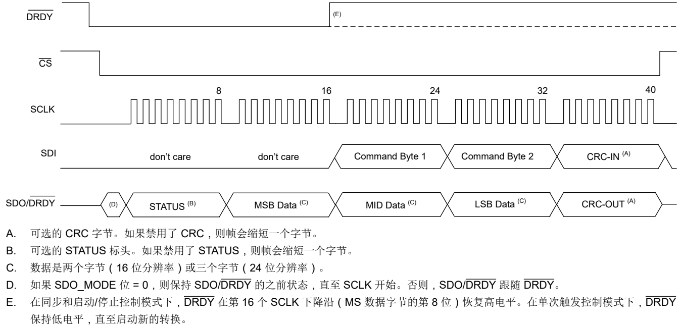
图 7-40. 转换数据读取，长格式
