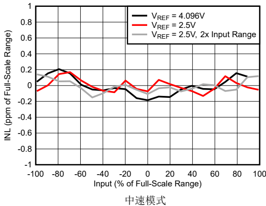
图 5-65. INL 误差与输入电压间的关系
