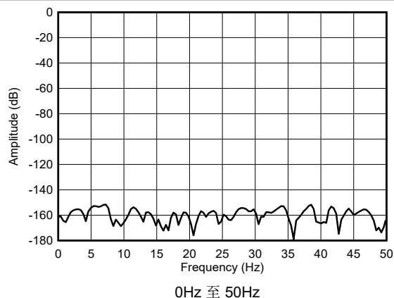
0Hz 至 50Hz 图 5-20. 中速模式，短接输入 FFT
