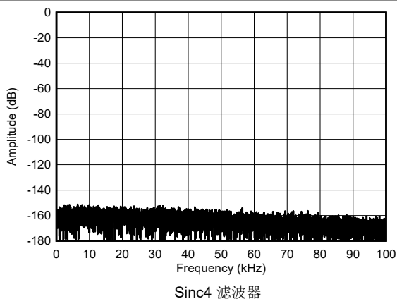
Sinc4 滤波器 图 5-22. 中速模式，短接输入 FFT
