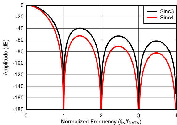
图 7-24. Sinc3 和 Sinc4 频率响应 (OSR = 32)
