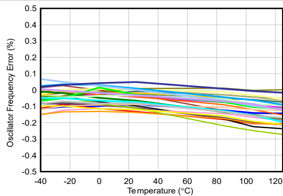
图 5-80. 振荡器频率与温度间的关系
