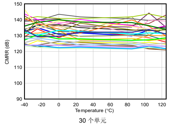
图 5-76. 直流 CMRR 与温度间的关系
