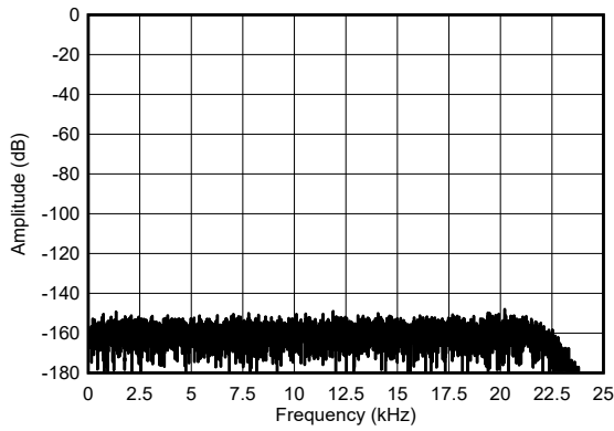
宽带滤波器 图 5-25. 低速模式，短接输入 FFT
