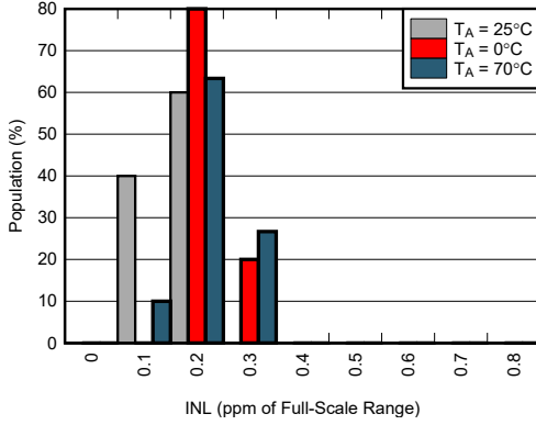
图 5-73. INL 分布图
