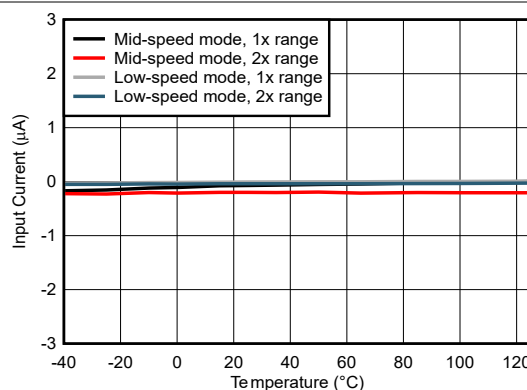
图 5-46. 输入电流与温度间的关系
