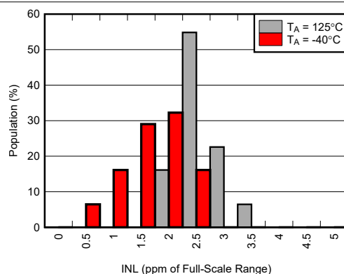
图 5-68. INL 分布图
