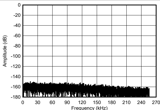
Sinc4 滤波器
