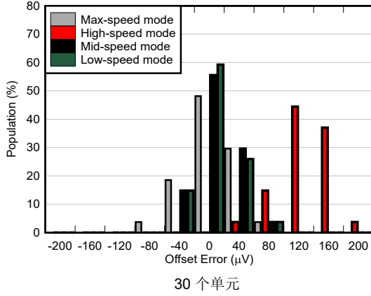
图 5-49. 偏移误差分布图
