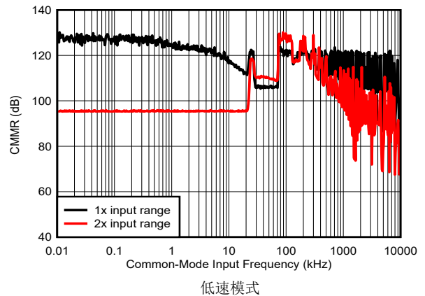
图 5-78. CMRR 与频率间的关系
