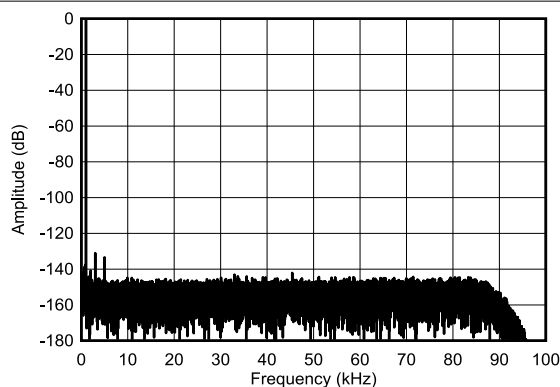
V_{IN} = -0.2dBFS ，1kHz，宽带滤波器 图 5-24. 中速模式，满量程 FFT
