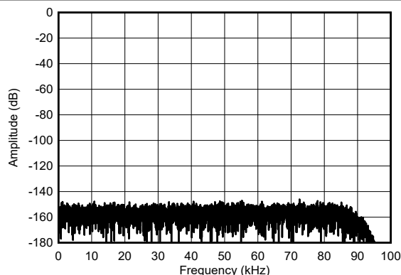
V_{REF} = 2.5V ，宽带滤波器，2 倍范围 图 5-21. 中速模式，短接输入 FFT
