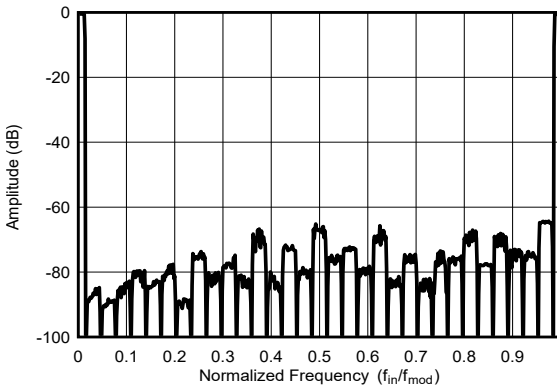
图 7-17. 宽带滤波器阻带衰减
