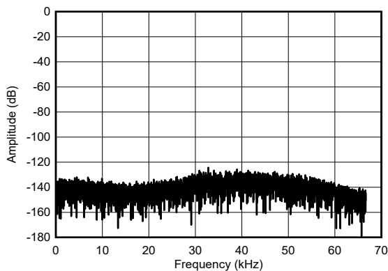
Sinc4 滤波器，OSR = 12 图 5-29. 低速模式，短接输入 FFT
