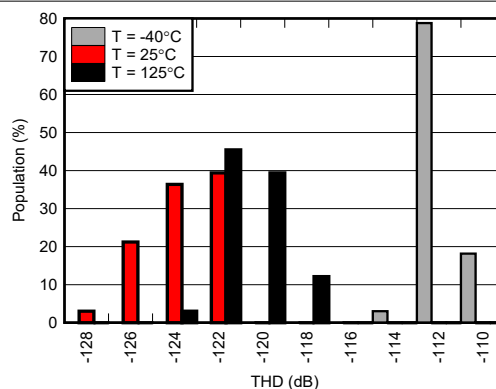
图 5-58. THD 分布图
