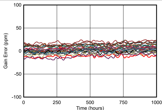
图 5-55. 增益漂移分布图
