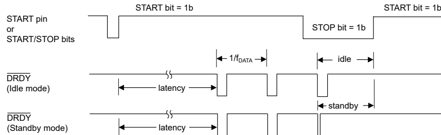
图 7-32. 启动/停止控制模式
