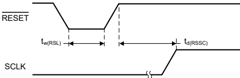
图 5-5. RESET 引脚时序
