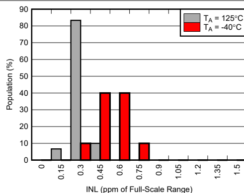
图 5-70. INL 分布图
