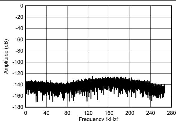
Sinc4 滤波器，OSR = 12 图 5-23. 中速模式，短接输入 FFT
