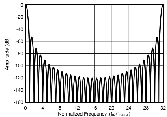
图 7-25. f_{MOD} 的 sinc4 频率响应 (OSR = 32)
