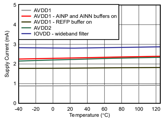
图 5-88. 电源电流与温度间的关系
