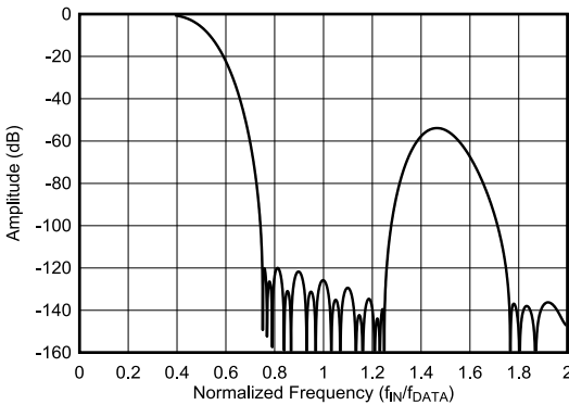
图 7-12. FIR2 滤波器频率响应 (OSR = 32)
