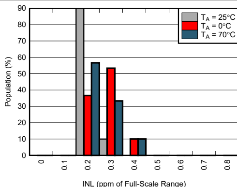
图 5-67. INL 分布图
