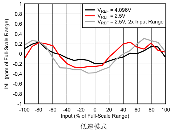
图 5-66. INL 误差与输入电压间的关系
