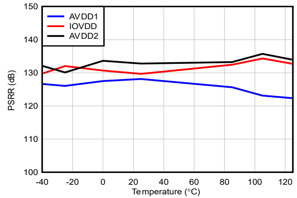
图 5-86. 直流 PSRR 与温度间的关系
