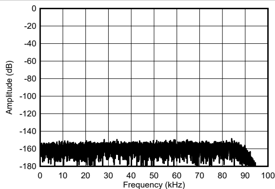
宽带滤波器 图 5-19. 中速模式，短接输入 FFT
