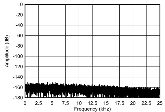
Sinc4 滤波器 图 5-28. 低速模式，短接输入 FFT
