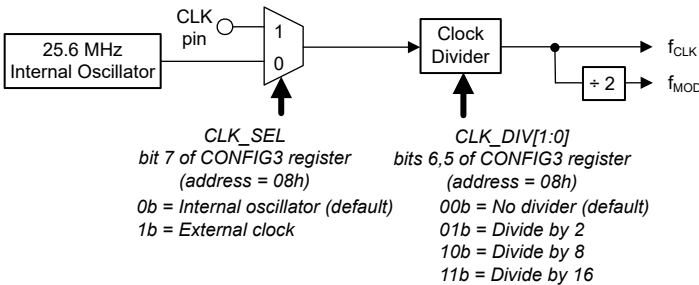
图 7-6. 时钟方框图
