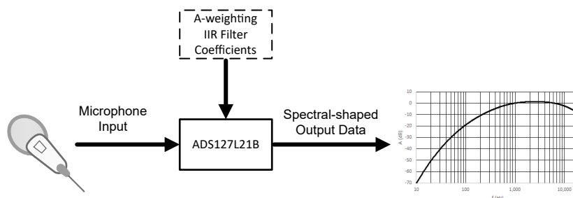
图 9-1. ADS127L21B A 加权补偿
