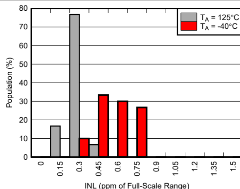
图 5-68. INL 分布图
