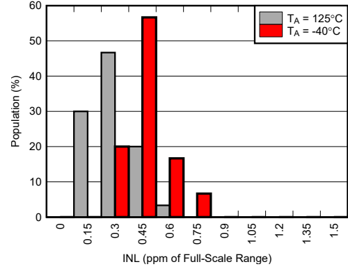
图 5-74. INL 分布图
