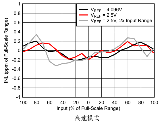
图 5-64. INL 误差与输入电压间的关系
