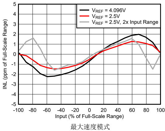
图 5-63. INL 误差与输入电压间的关系
