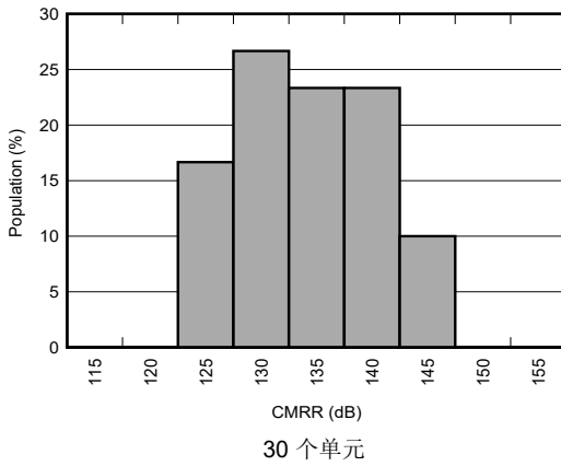
图 5-75. 直流 CMRR 分布图
