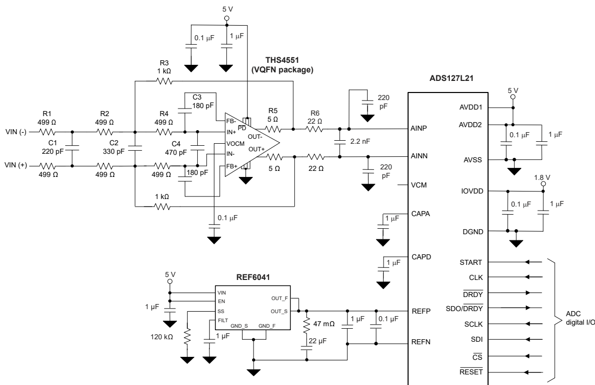
图 9-8. ADS127L21 电路图
