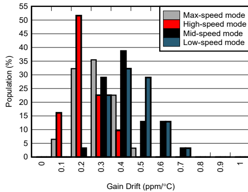
图 5-55. 增益漂移分布图
