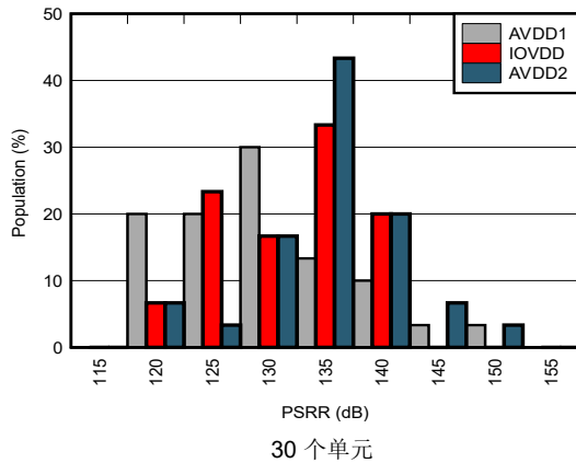
图 5-79. 直流 PSRR 分布图
