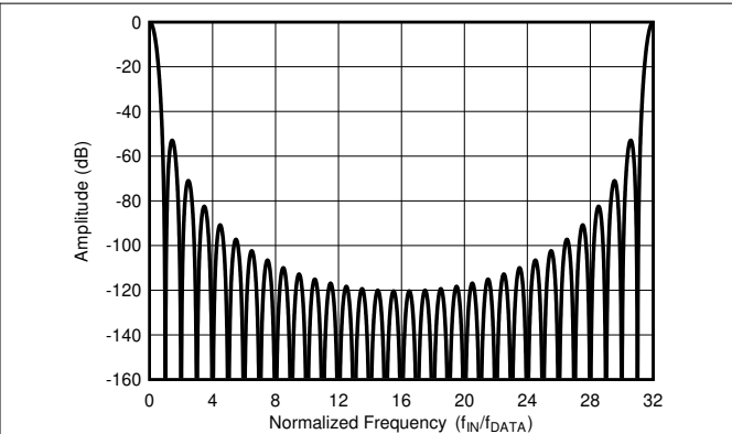
图 7-25. f_{\text{MOD}} 的 Sinc4 频率响应 (OSR = 32)
