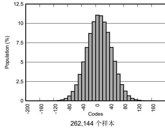
图 5-32. 高速模式代码分布图
