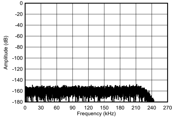
图 5-7. 最大速度模式，短接输入 FFT
