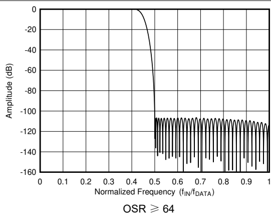
图 7-16. 宽带滤波器频率响应
