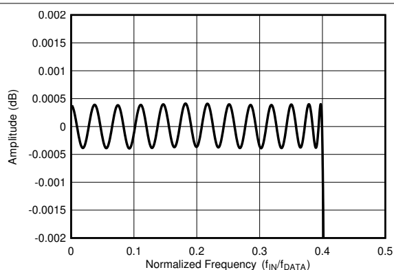
图 7-14. 宽带滤波器通带纹波
