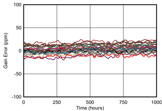
图 5-55. 增益漂移分布图
