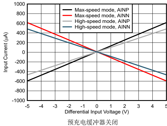
图 5-43. 输入电流与差分电压间的关系
