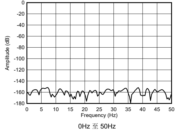
图 5-20. 中速模式，短接输入 FFT
