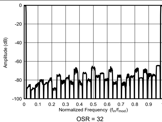
图 7-17. 宽带滤波器阻带衰减
