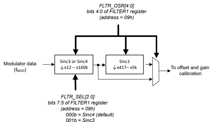
图 7-23. Sinc 滤波器方框图
