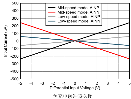
图 5-44. 输入电流与差分电压间的关系
