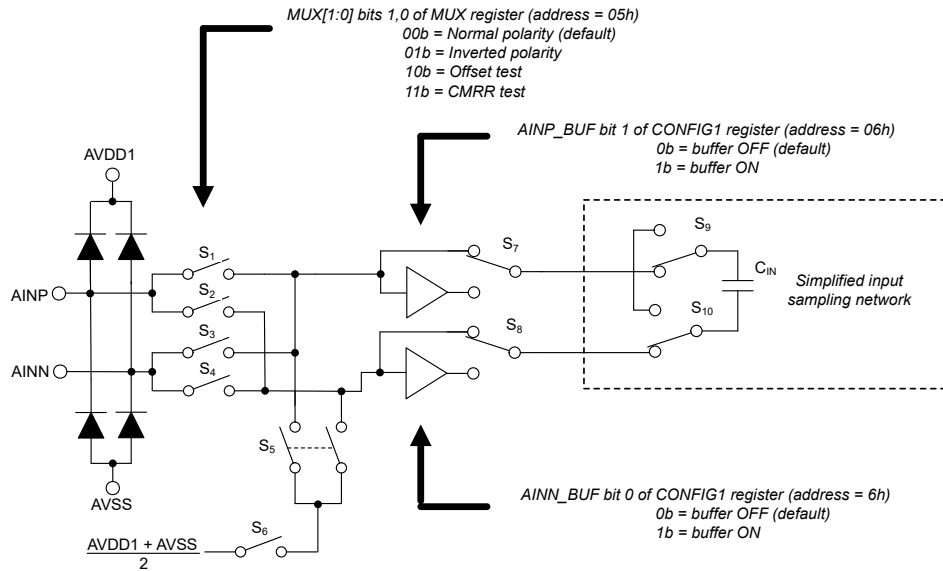
图 7-3. 模拟输入电路
