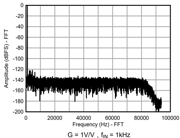
图 9-5. 宽带滤波器性能
