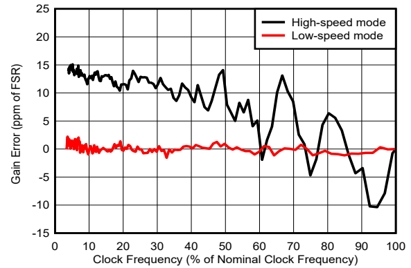
图 5-56. 增益误差与时钟频率间的关系
