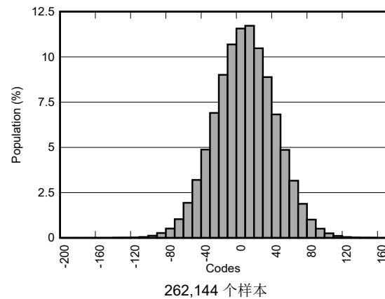
图 5-34. 低速模式代码分布图
