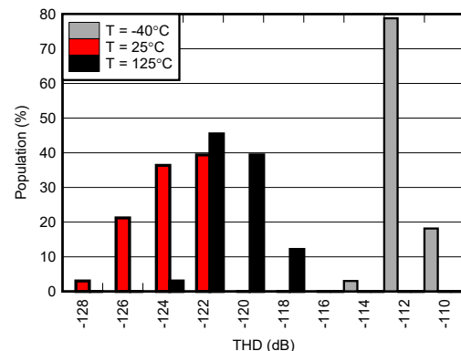
图 5-58. THD 分布图
