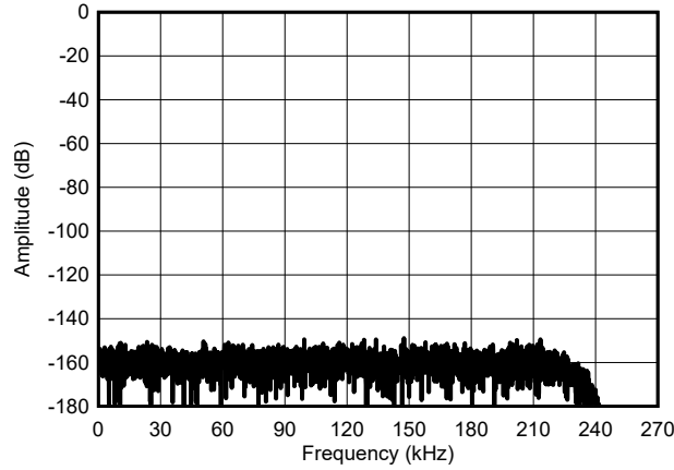
图 5-8. 最大速度模式，短接 FFT
