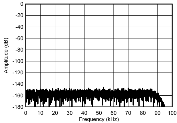
图 5-20. 中速模式，短接 FFT
