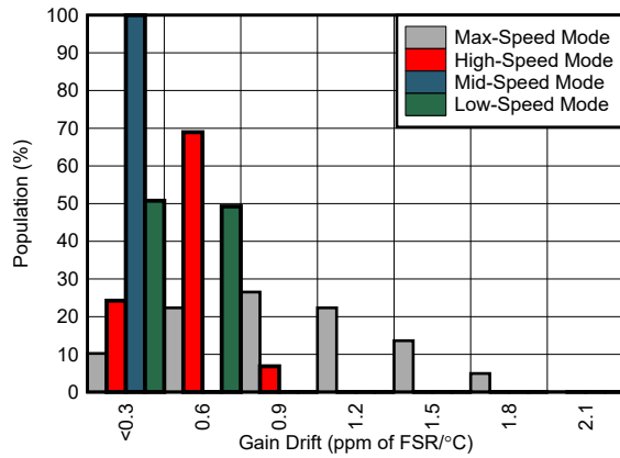
图 5-44. 增益漂移直方图
