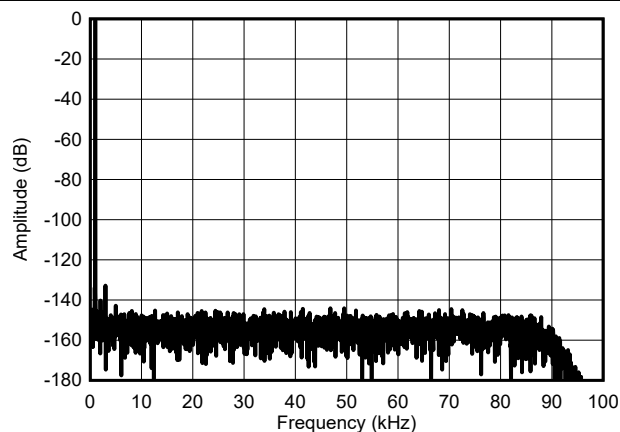
图 5-22. 中速模式，短接 FFT
