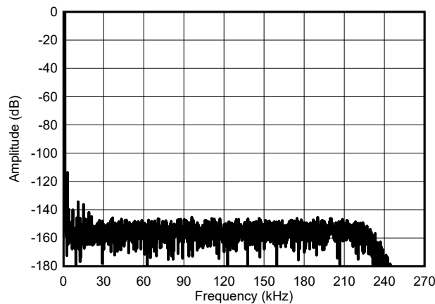
图 5-10. 最大速度模式，短接 FFT
