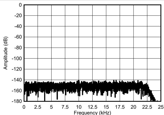
图 5-26. 低速模式，短接 FFT
