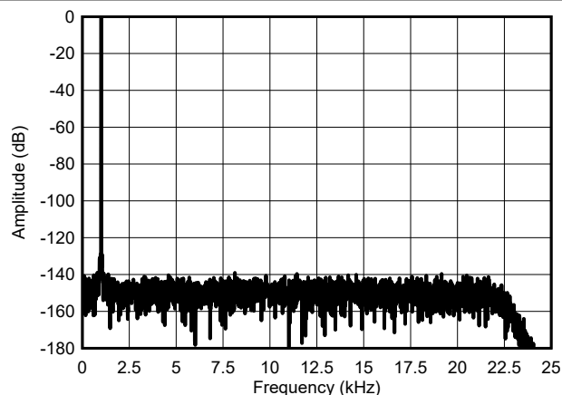
图 5-28. 低速模式，短接 FFT
