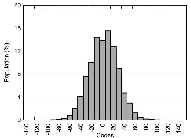
图 5-11. 最大速度模式，短接 FFT
