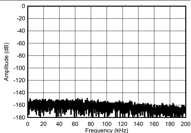
图 5-15. 高速模式，短接 FFT
