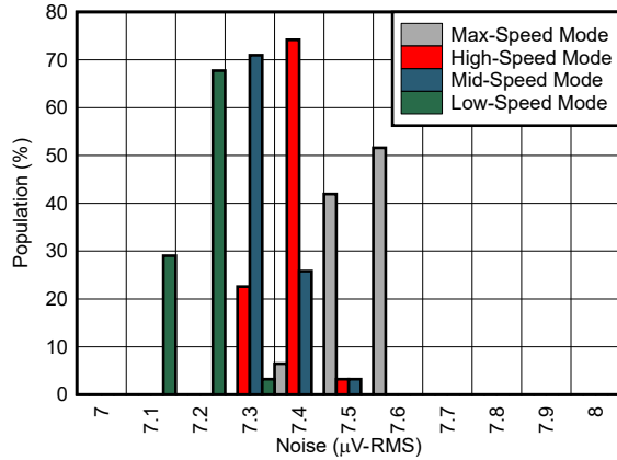
图 5-32. 集成噪声直方图
