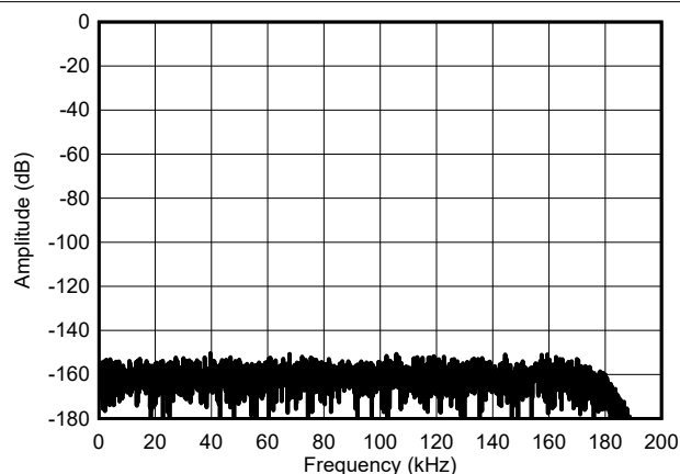
图 5-14. 高速模式，短接 FFT
