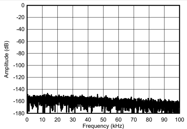
图 5-21. 中速模式，短接 FFT
