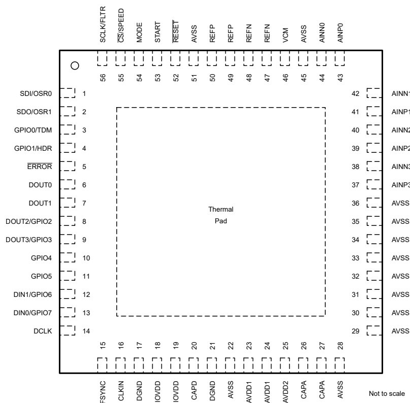
图 4-1. ADS127L14 RSH 封装，56 引脚 VQFN（顶视图）
