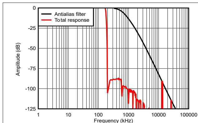
图 9-2. 抗混叠滤波器频率响应
