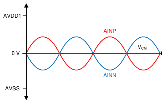
图 7-2. 双极差分输入信号
