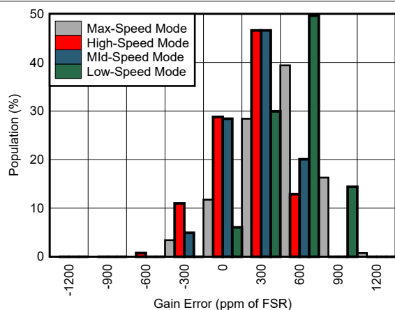
图 5-42. 增益误差直方图
