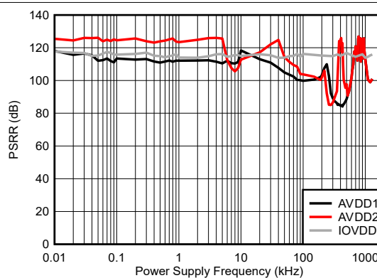
高速模式, sinc4 滤波器
