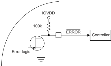
图 7-29. \overline{\text{ERROR}} 引脚
