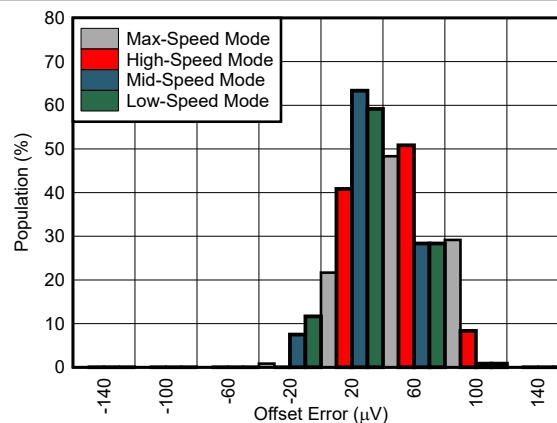
图 5-39. 失调电压直方图
