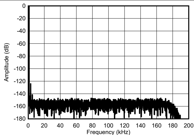
图 5-16. 高速模式，短接 FFT
