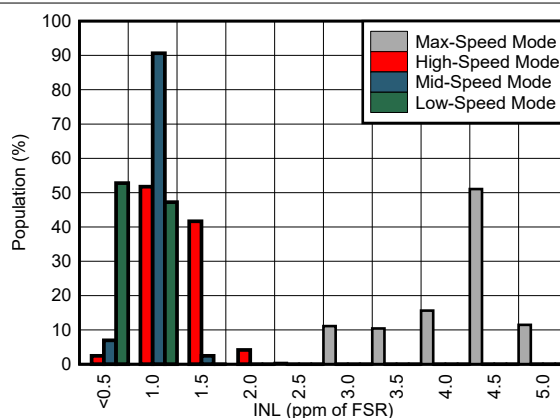
图 5-55. INL 直方图
