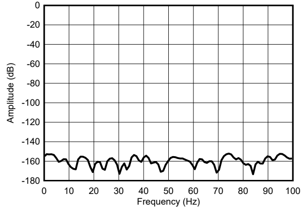
图 5-9. 最大速度模式，短接 FFT
