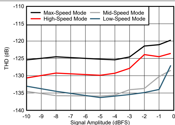
图 5-50. THD 与信号幅值间的关系
