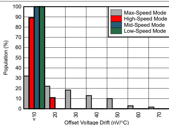
图 5-40. 失调电压漂移直方图
