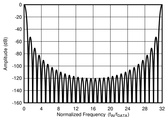
图 7-19. f MOD 的 Sinc4 频率响应 (OSR = 32)
