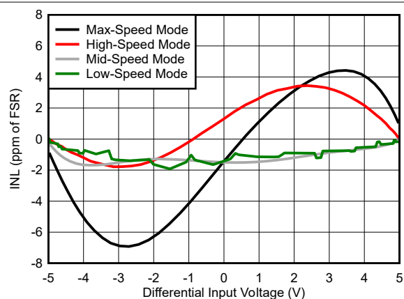
图 5-54. INL 与输入电压间的关系
