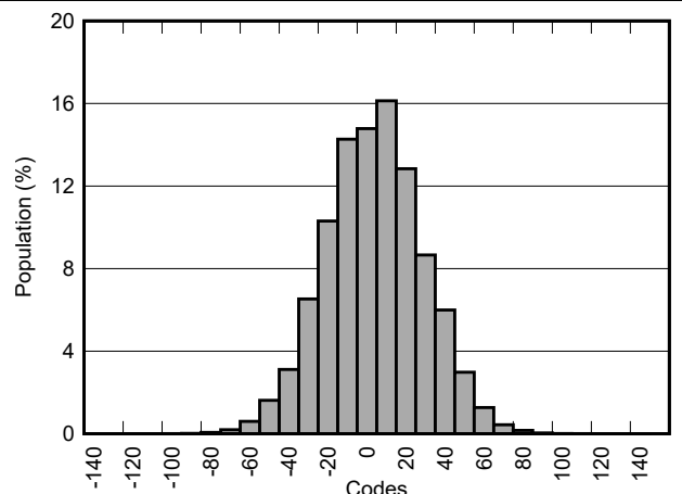
图 5-23. 中速模式，短接 FFT
