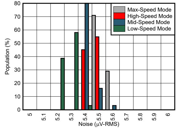
图 5-33. 集成噪声直方图
