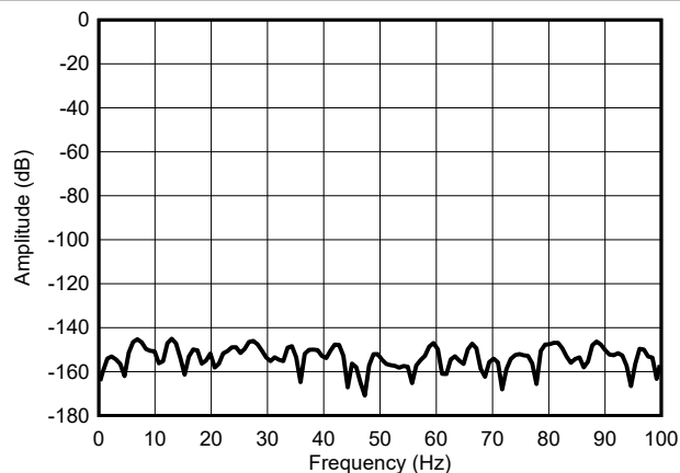
图 5-27. 低速模式，短接 FFT
