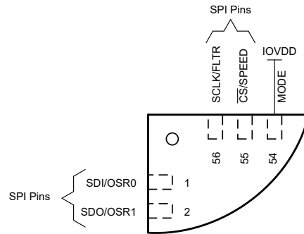
图 7-45. SPI 引脚
