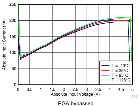
图 7-26. ADC1 Absolute Input Current
