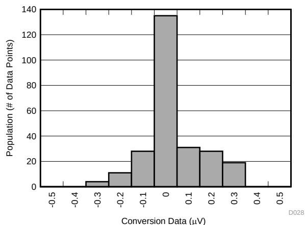
图 22. Conversion Data Histogram
