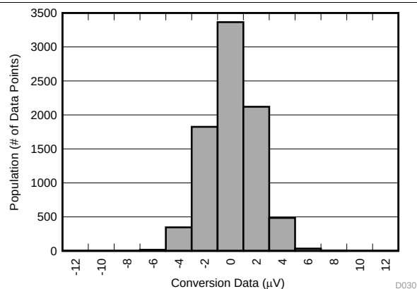
图 22. Conversion Data Histogram
