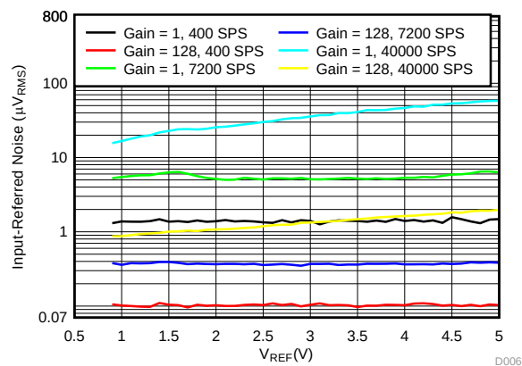
图 21. Noise vs Reference Voltage
