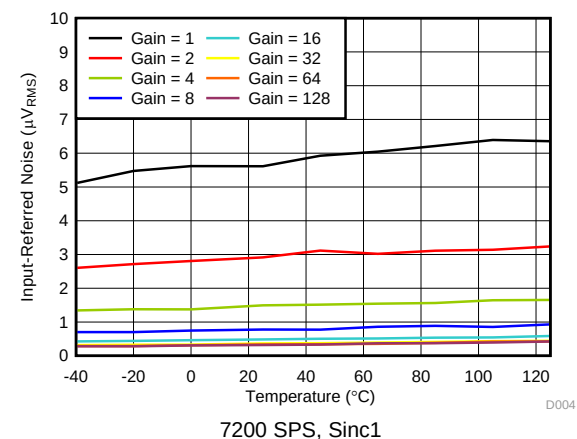
图 19. Noise vs Temperature
