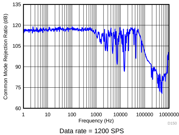
图 39. CMRR vs Frequency
