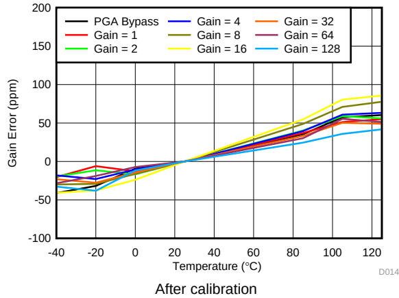
图 15. Gain Error vs Temperature
