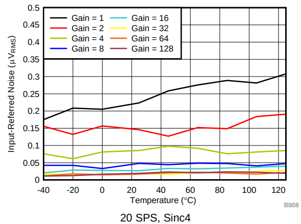
图 18. Noise vs Temperature
