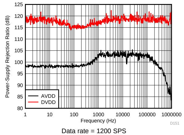
图 40. PSRR vs Frequency
