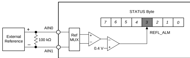
图 54. Reference Monitor
