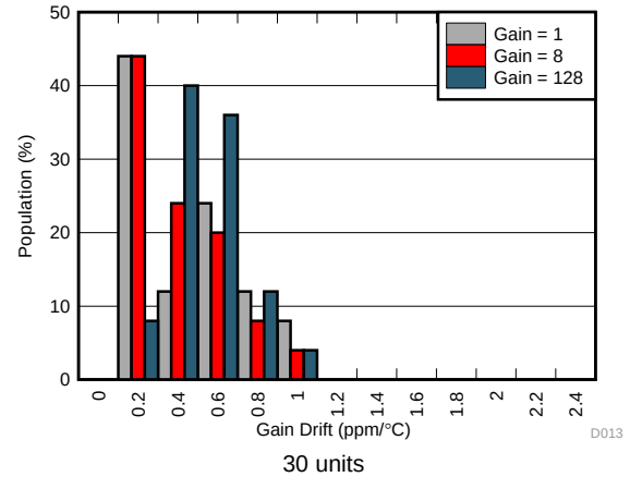
图 16. Gain Error Drift Distributions
