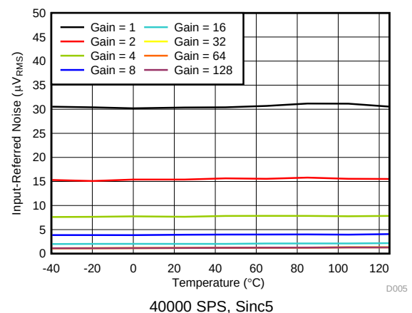
图 20. Noise vs Temperature
