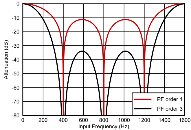
图 7-32. 并行后置滤波器频率响应，4 个平均值和 1.6kHz 扫描速率
