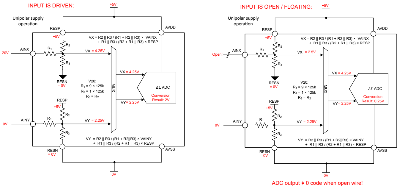
图 7-28. 开路条件下的 ADC 输出，RESP 连接至 AVDD
