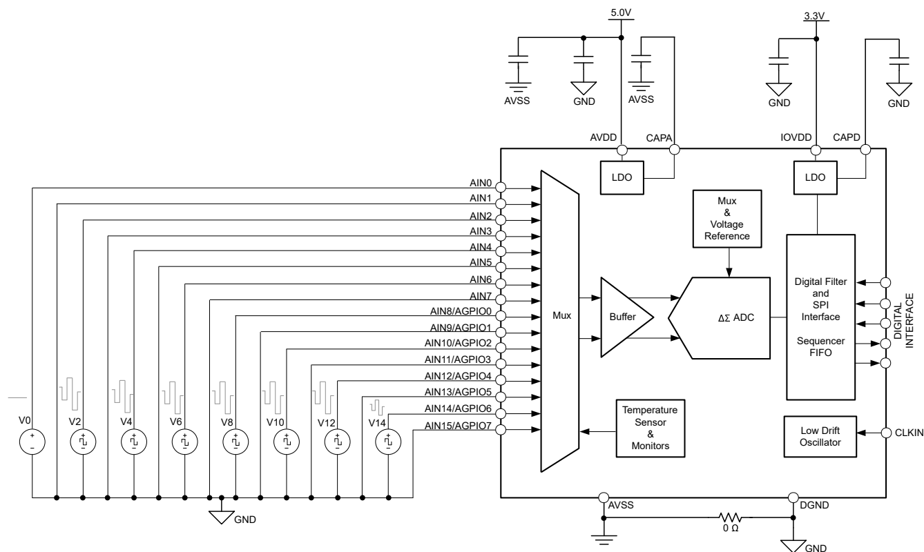
图 8-5. 串扰测试设置
