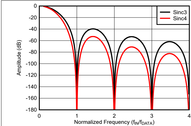
图 7-12. Sinc3 和 Sinc4 频率响应
