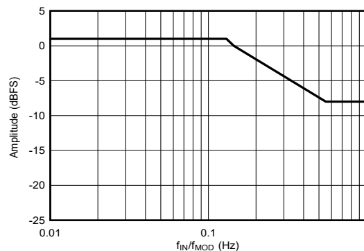
图 7-9. 为避免调制器饱和而设置的振幅限制
