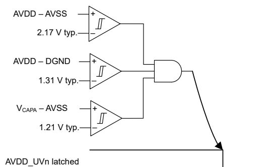
图 7-7. 模拟电源阈值
