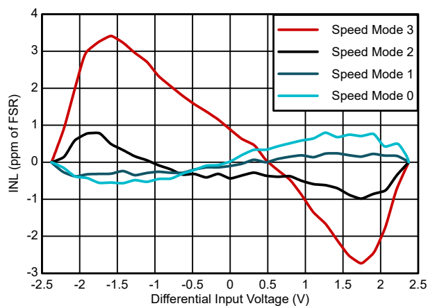
图 5-6. INL 与差分输入电压间的关系
