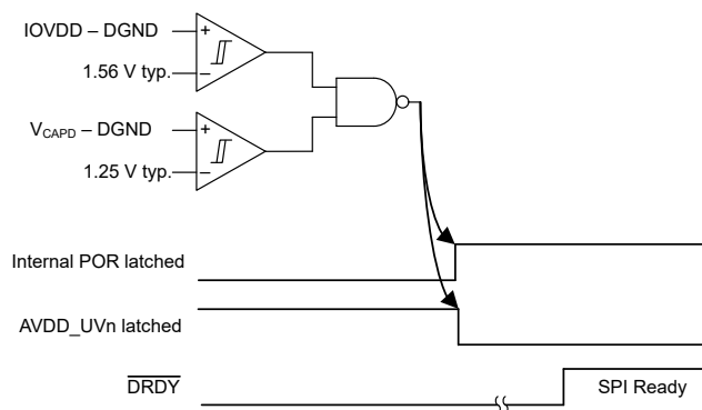
图 7-6. 数字电源阈值
