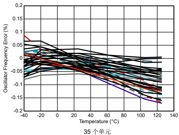
图 5-11. 内部振荡器频率与温度间的关系
