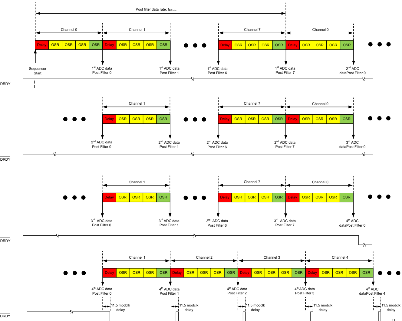
图 7-34. 使用后置滤波器时的 \overline{\text{DRDY}} 行为
