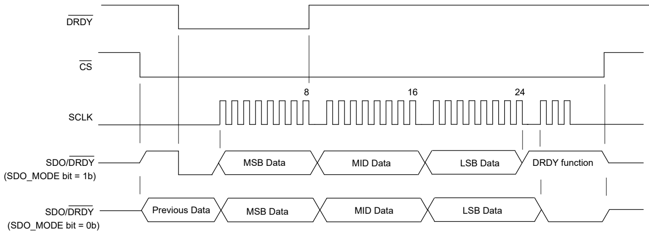
图 7-42. 具有额外 SCLK 脉冲时的 SDO/DRDY 和 DRDY 功能
