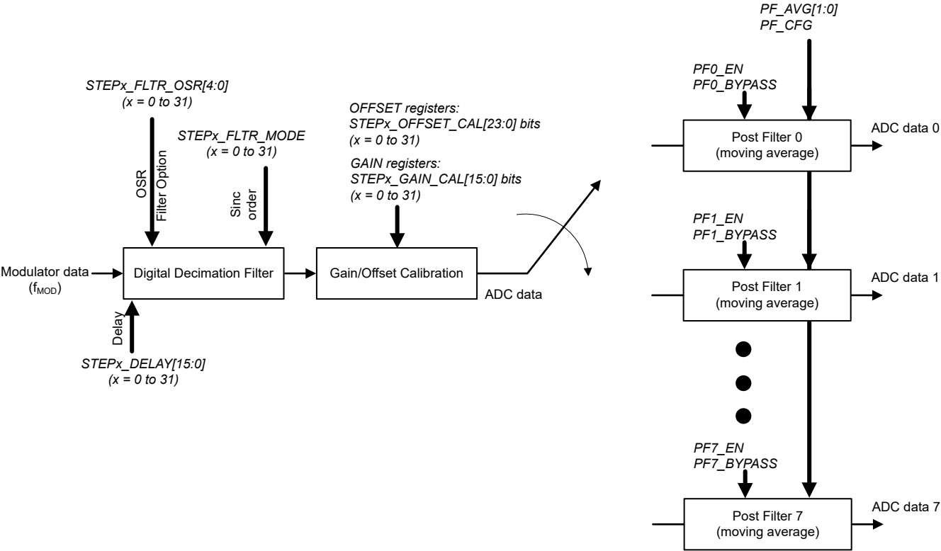
图 7-30. 并行后置滤波器方框图
