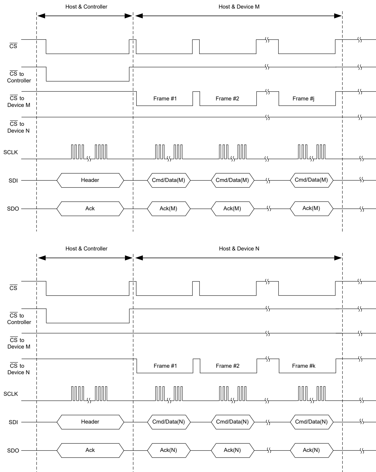
图 7-37. CS 转发时序图
