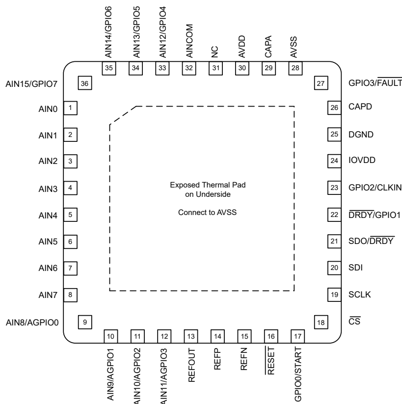
图 4-1. RHB 封装，36 引脚 VQFN（顶视图）
