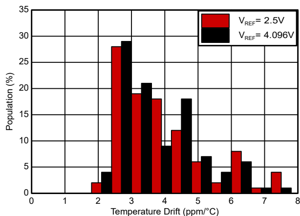
图 5-7. 内部基准温漂
