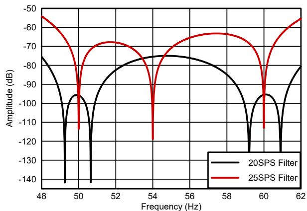
图 7-16. 20SPS 滤波器和 25SPS 滤波器频率响应， 48Hz 至 62Hz
