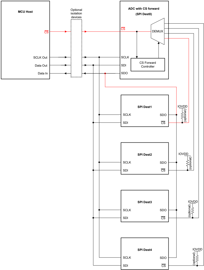
图 7-35. CS 转发方框图
