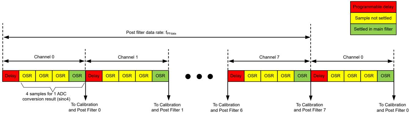
图 7-31. 并行后置滤波器计时示意图
