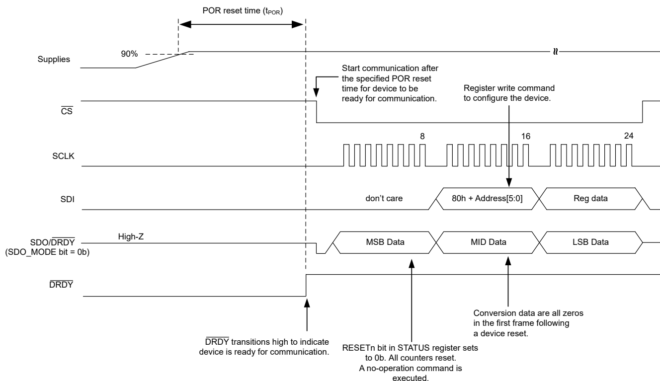
图 7-60. 上电复位后的 SPI 通信
