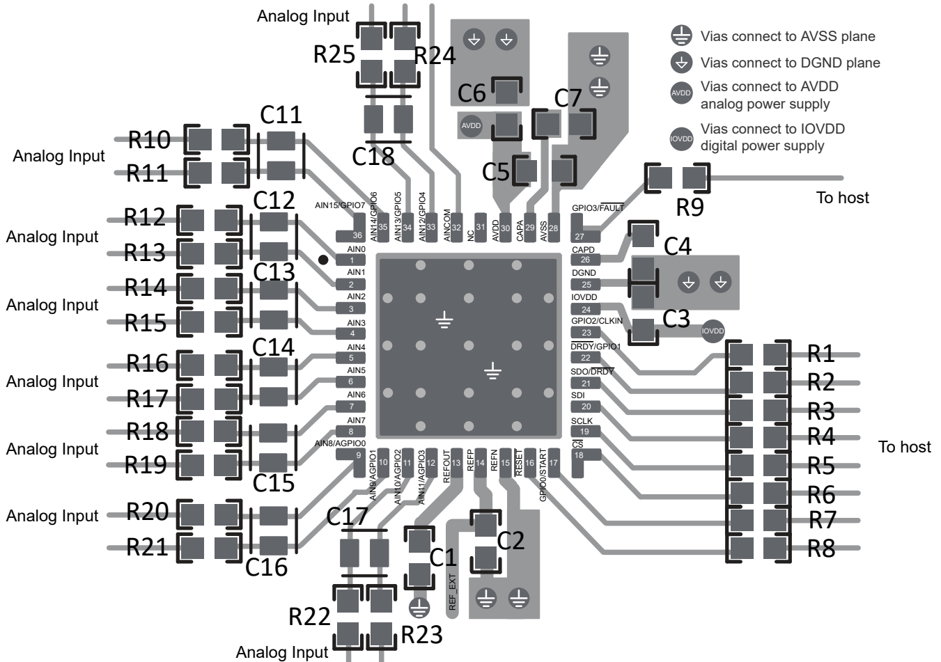
图 8-10. 布局示例
