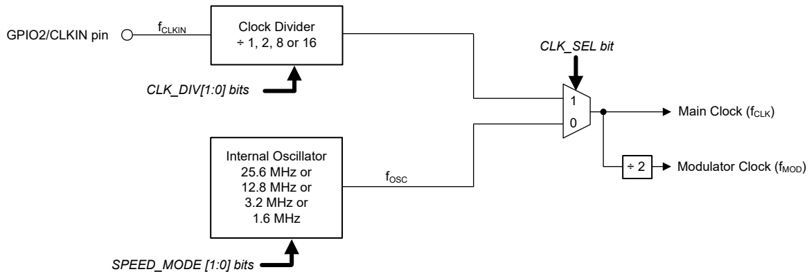
图 7-8. 时钟方框图
