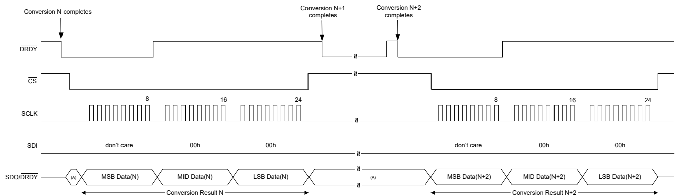
图 7-65. DRDY 引脚行为：在新的转换完成时读取转换数据
