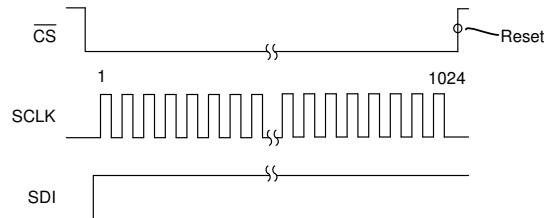
图 7-40. 复位模式 2 ( 4 线 SPI 模式 )
