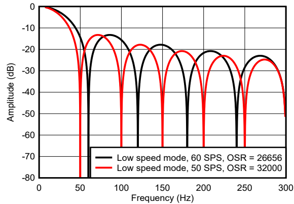
图 7-14. Sinc4 + Sinc1 级联滤波器频率响应
