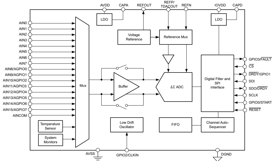
简化版方框图
