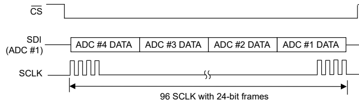
图 7-70. 24 位数据输入序列
