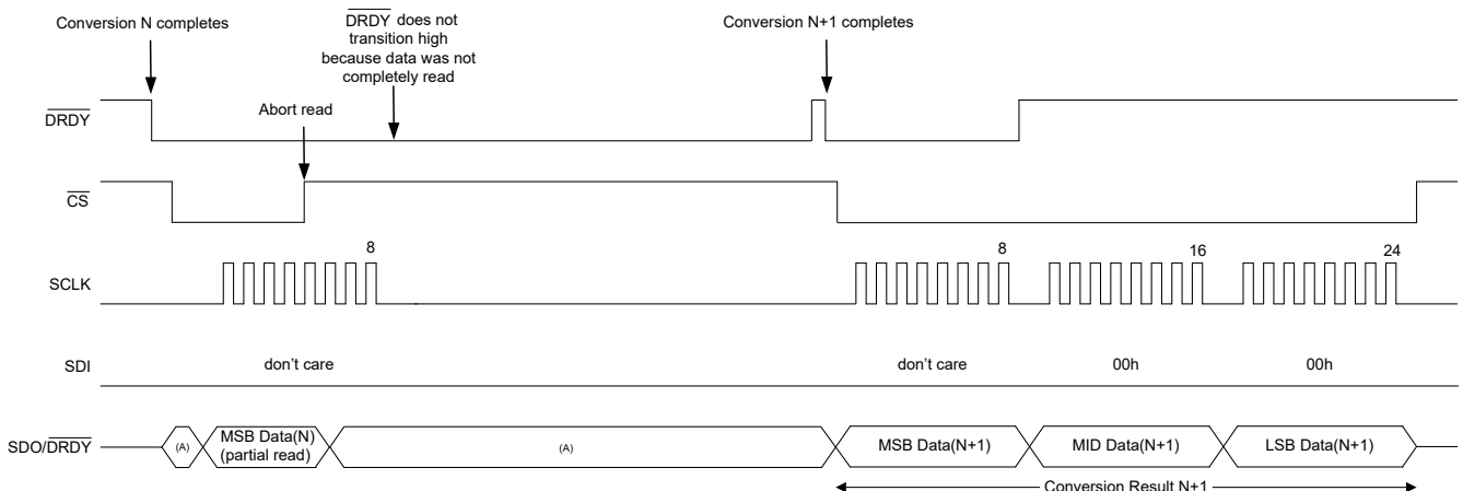
图 7-62. \overline{\text{DRDY}} 引脚行为：在新的转换完成之前读取转换数据
