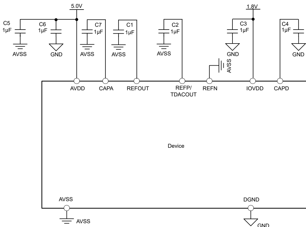
图 8-9. 电源去耦
