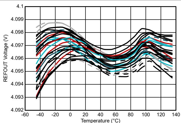
图 5-7. 内部基准温漂
