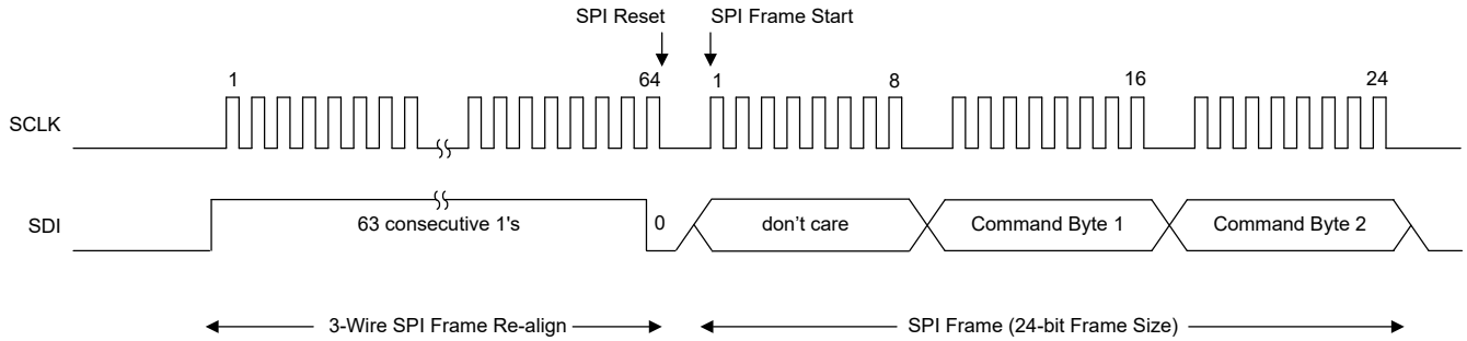
图 7-74. 3 线模式 SPI 重新对齐模式
