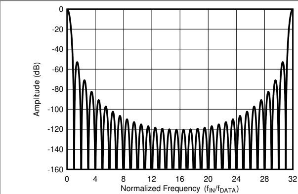
图 7-13. f_{\text{MOD}} 的 Sinc4 频率响应 (OSR = 32)
