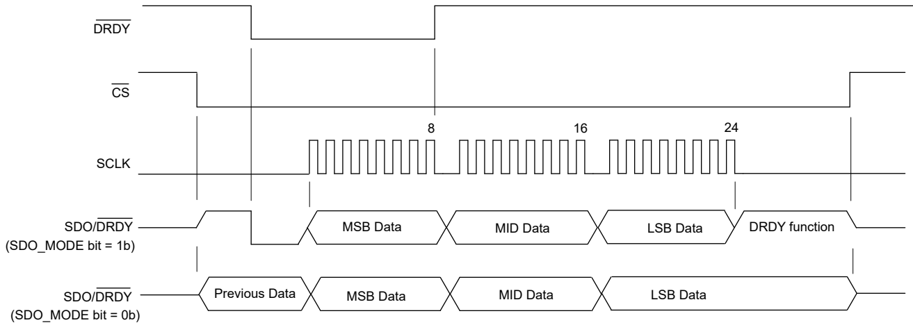
图 7-41. SDO/DRDY 和 DRDY 功能
