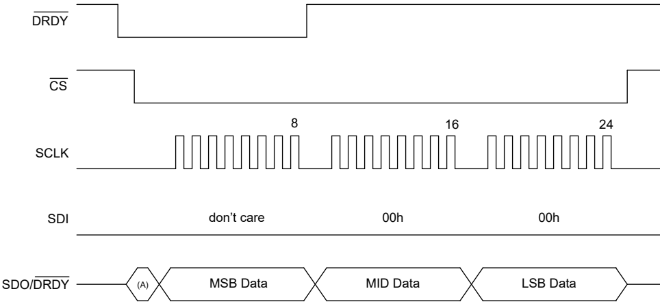
图 7-45. 读取转换数据，24 位帧大小
