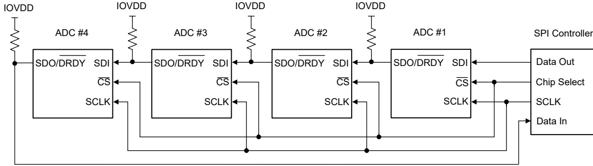
图 7-69. 菊花链连接
