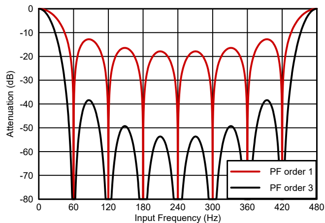
图 7-33. 并行后置滤波器频率响应，8 个平均值和 480Hz 扫描速率
