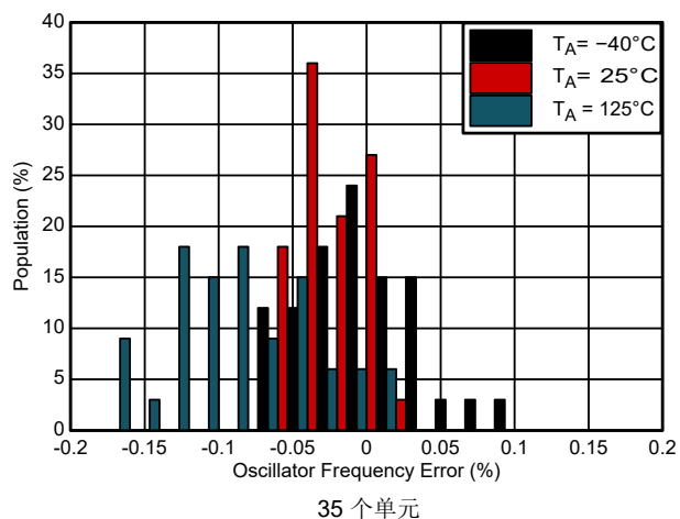
图 5-10. 内部振荡器频率直方图
