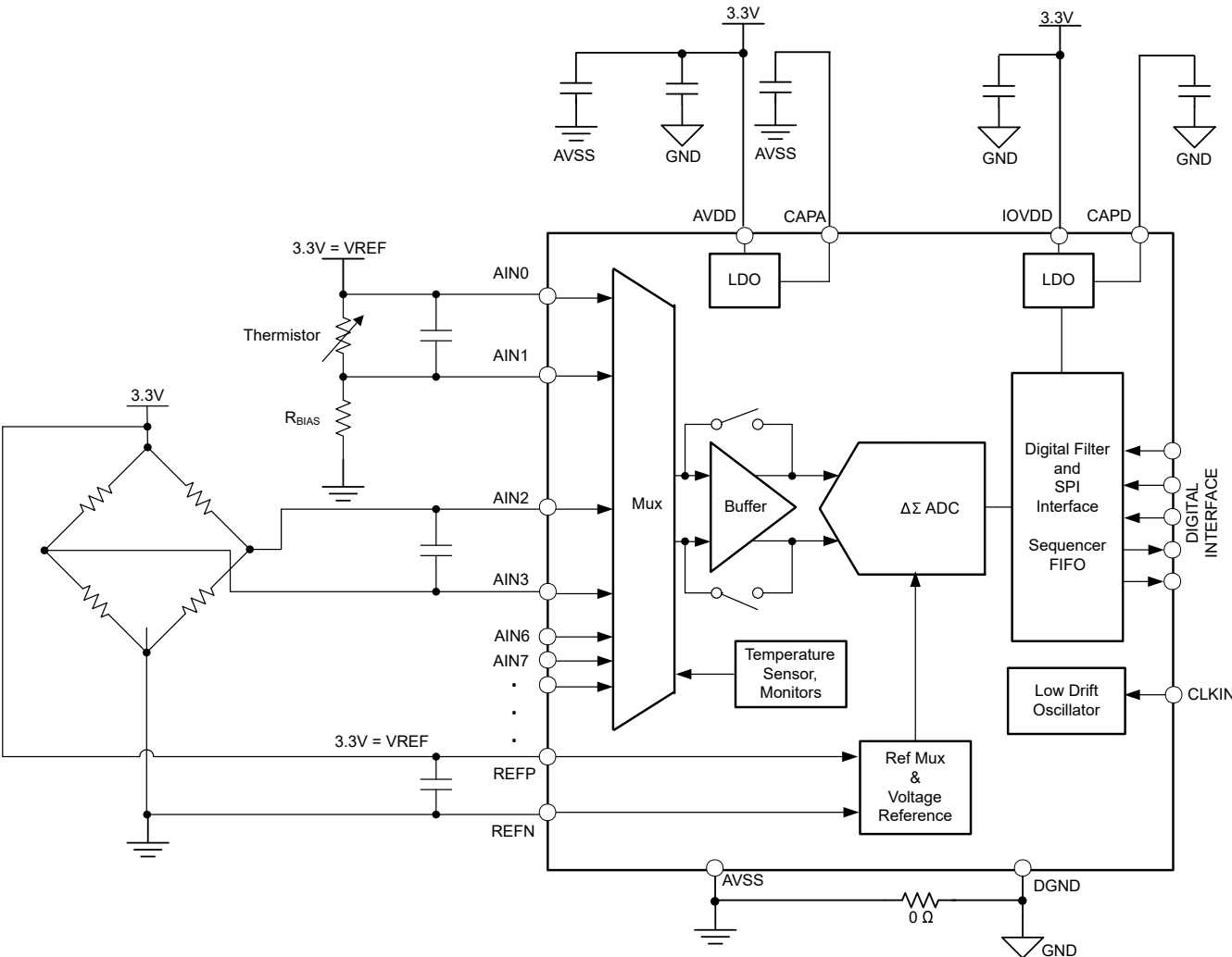
图 8-4. 使用 ADS125P08 进行电阻式电桥传感器测量，使用模拟电源作为桥励磁，使用热敏电阻进行电桥温度测量
