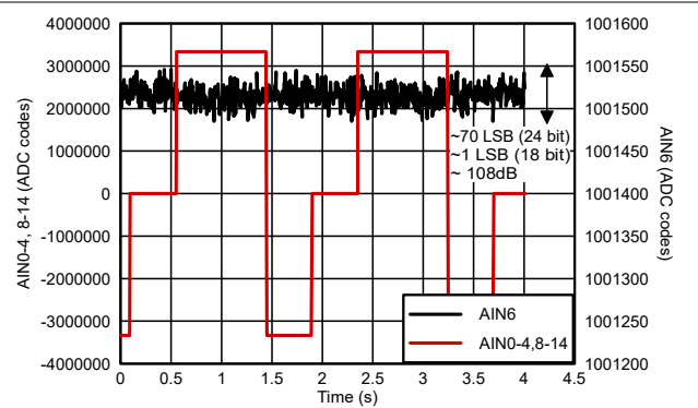
图 8-8. ADC 输入 AIN6 的串扰测量
