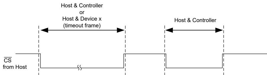
图 7-36. 超时图表
