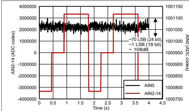
图 8-7. ADC 输入 AIN0 的串扰测量
