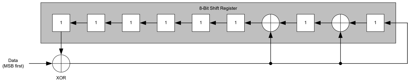
图 7-44. CRC 计算的可视化表示
