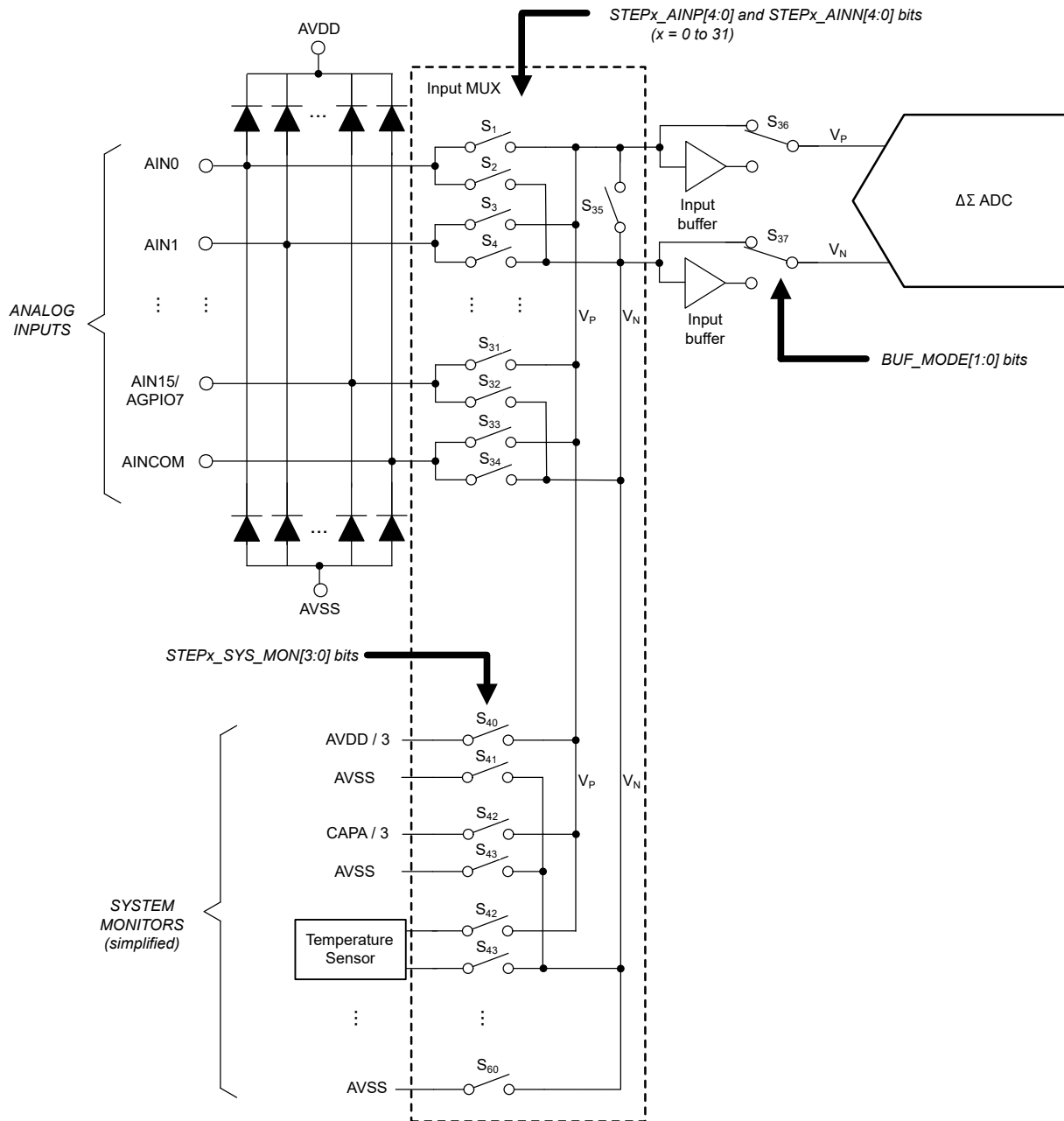
图 7-1. 输入多路复用器
