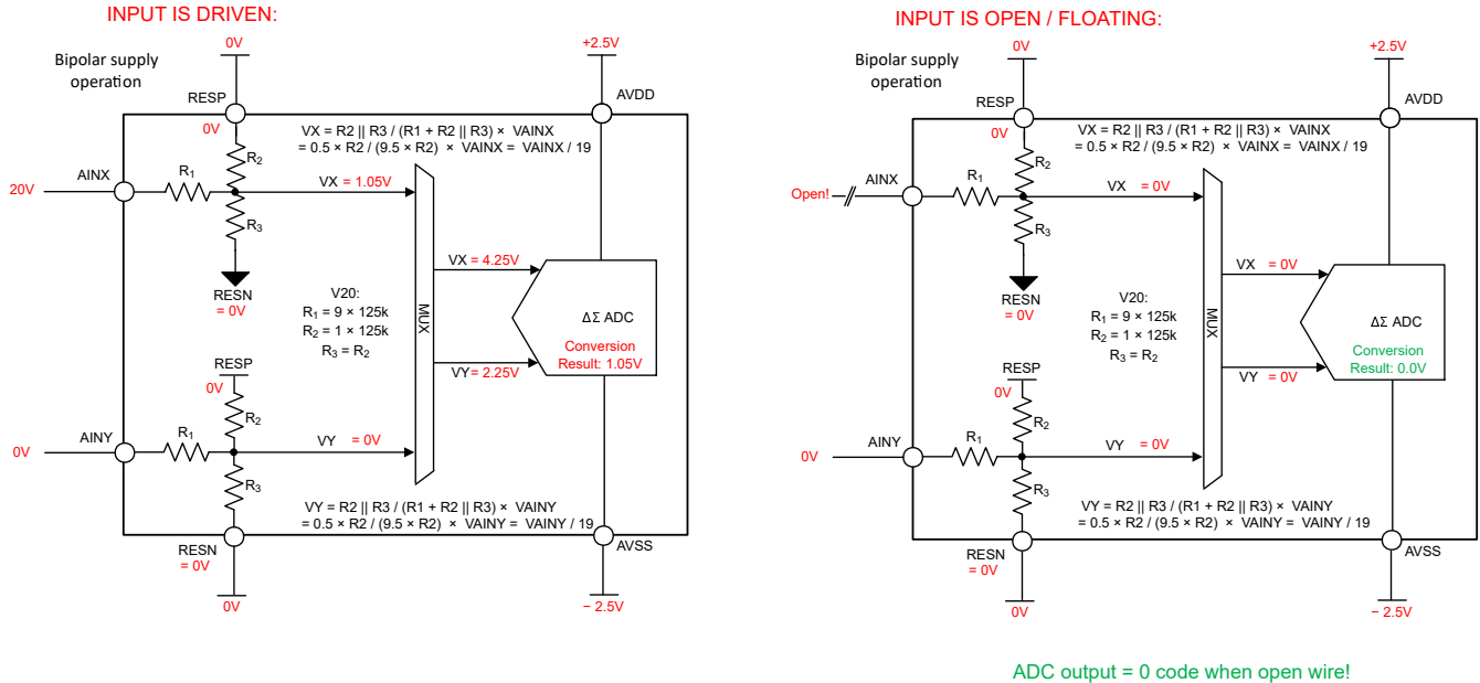
图 7-29. 开路条件下的 ADC 输出, RESP 和 RESN 连接至 GND
