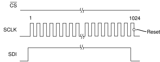
图 7-39. 复位模式 1 ( 3 线或 4 线 SPI 模式 )
