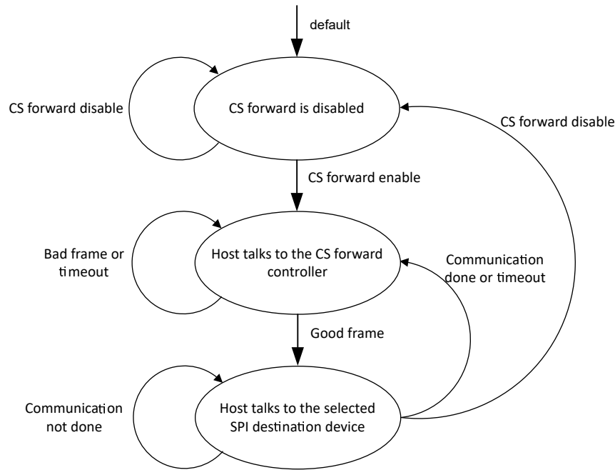
图 7-38. CS 转发状态图
