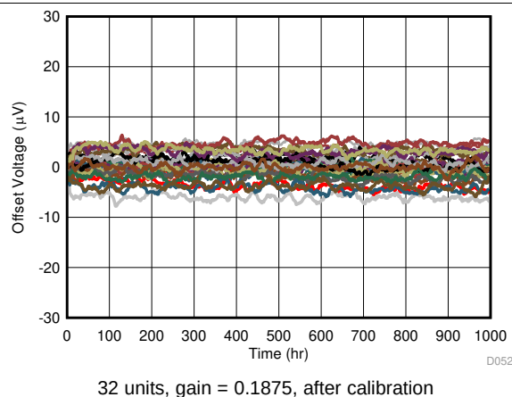
图 27. Offset Voltage Long-Term Drift
