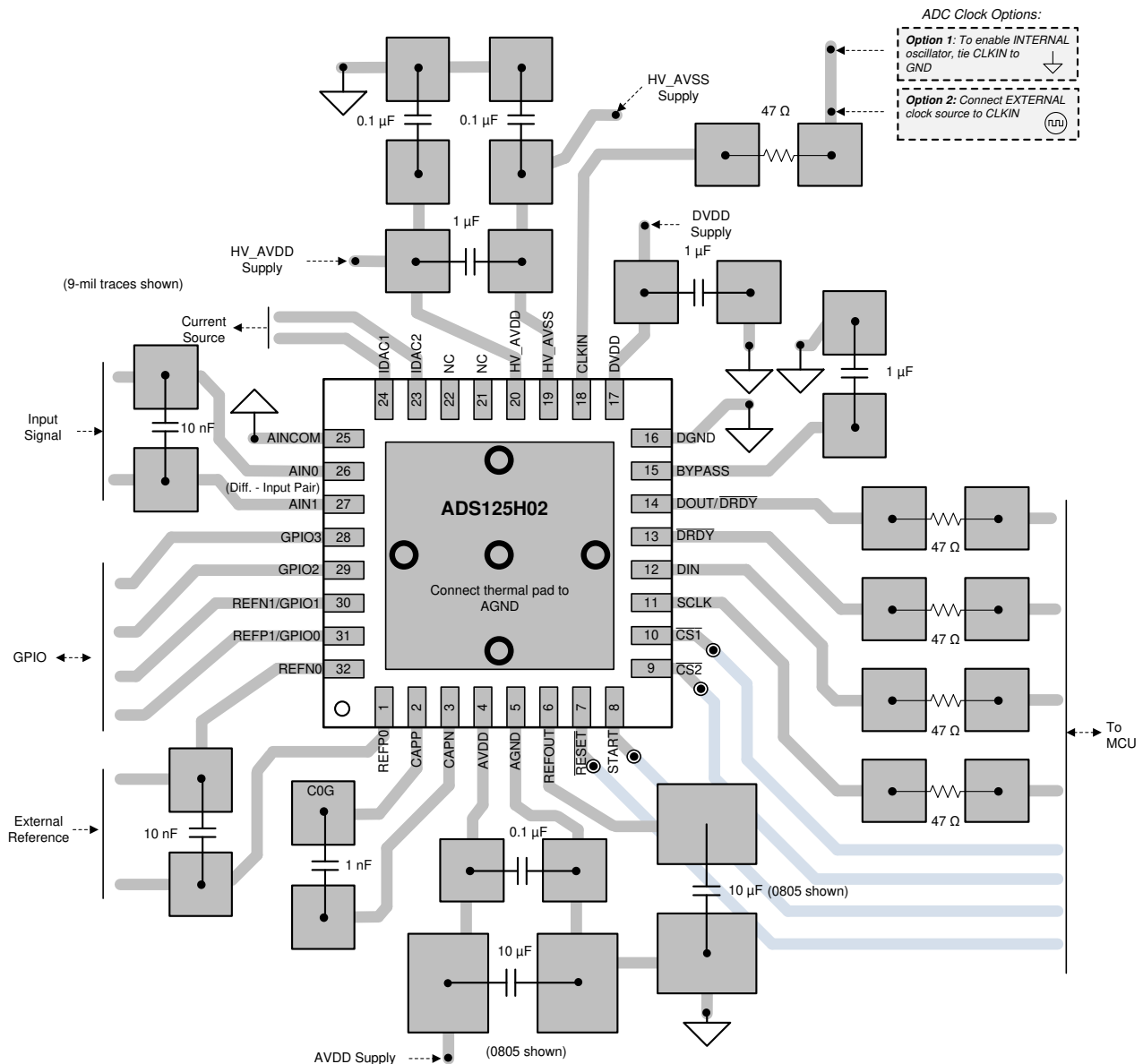
图 103. PCB Layout Example
