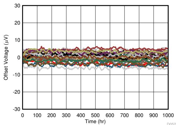
图 7-14. Offset Error Drift Distribution
