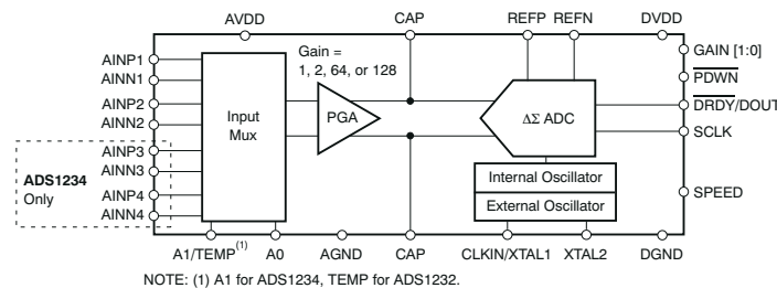
方框图
