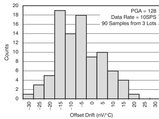
图 5-14. Offset Drift (25°C to 105°C)
