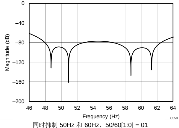
图 47. 滤波器响应详细视图 (DR = 20SPS)
