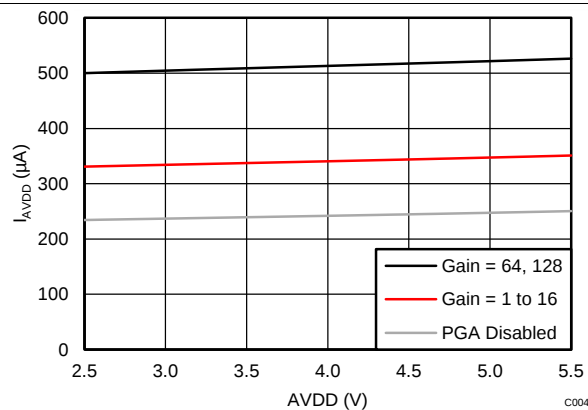
图 33. I_{AVDD} 与 AVDD 间的关系
