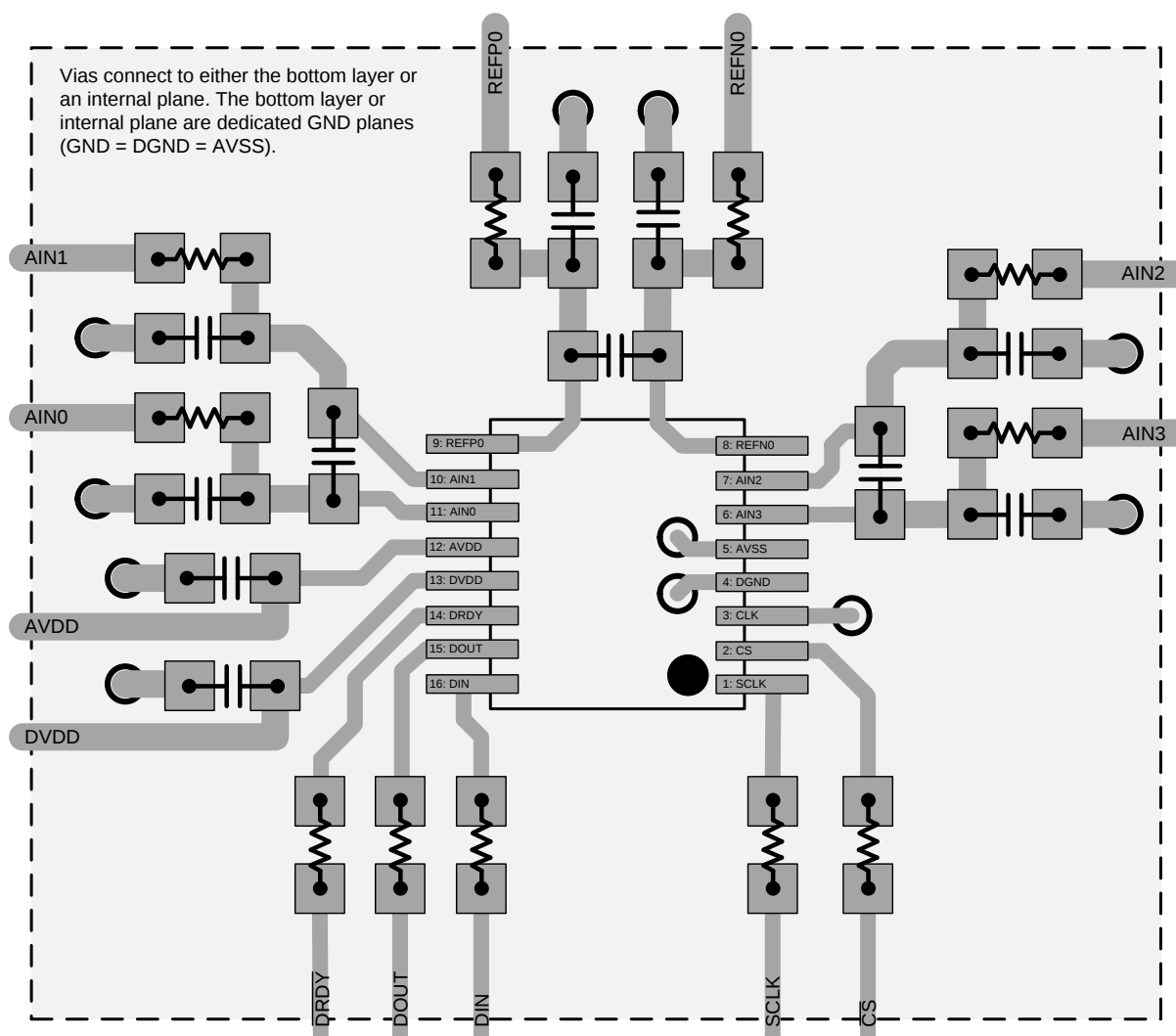
图 87. 布局示例
