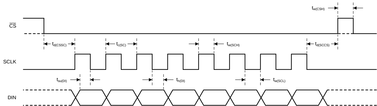
图 1. 串行接口时序要求
