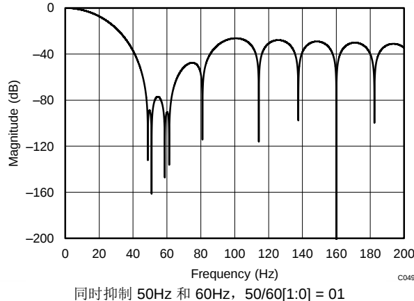
图 46. 滤波器响应 (DR = 20SPS)
