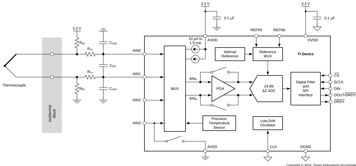
图 74. 热电偶测量
