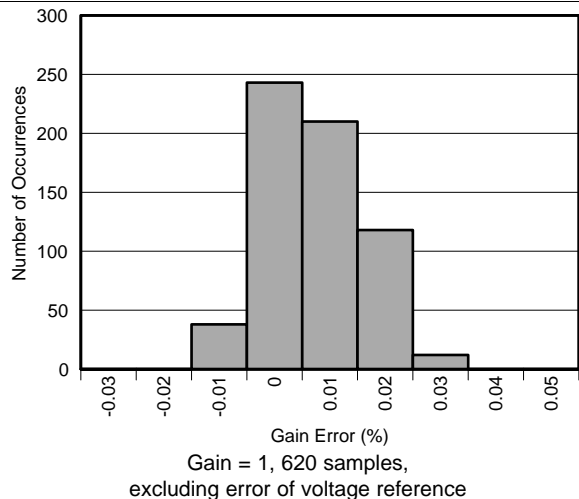
图 10. Gain Error Histogram
