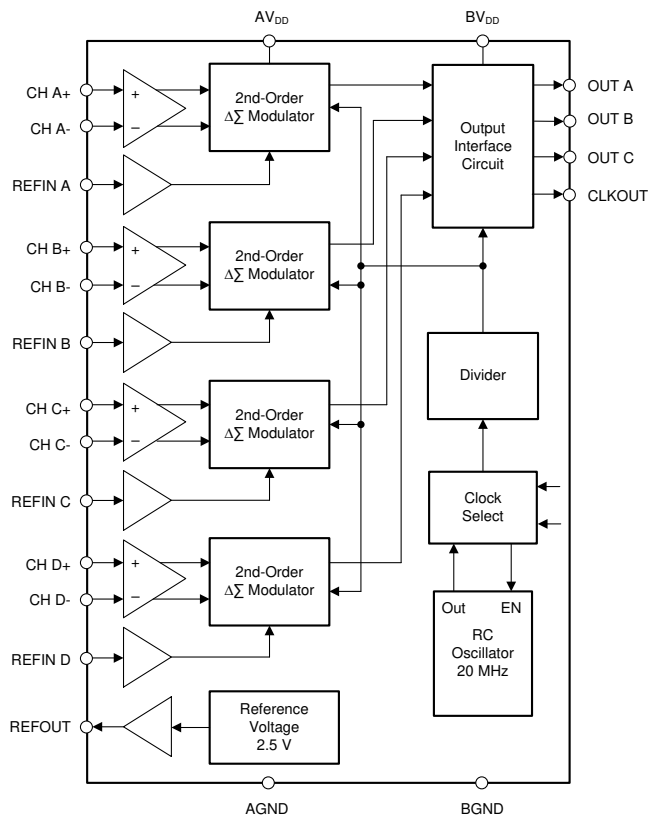
功能方框图
