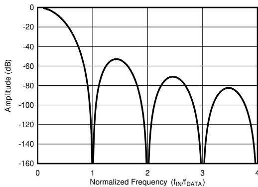
图 8-14. Sinc4 频率响应 (OSR = 32)
