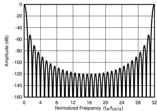
图 8-15. Sinc4 频率响应到 f_{MOD} (OSR = 32)
