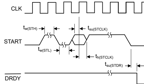
图 6-4. START Pin Timing
