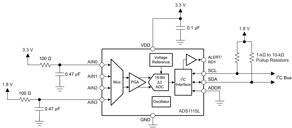
图 10-9. 监控两个电源电压轨：使用 ADS1115L
