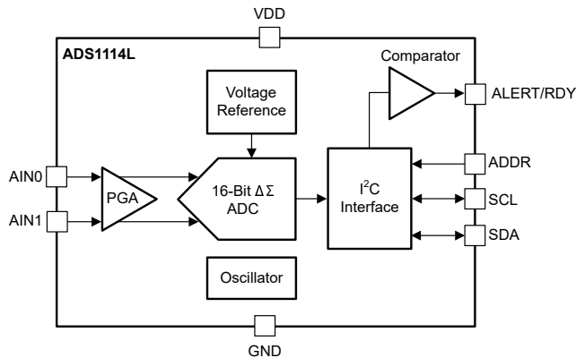
图 8-1. ADS1114L 方框图
