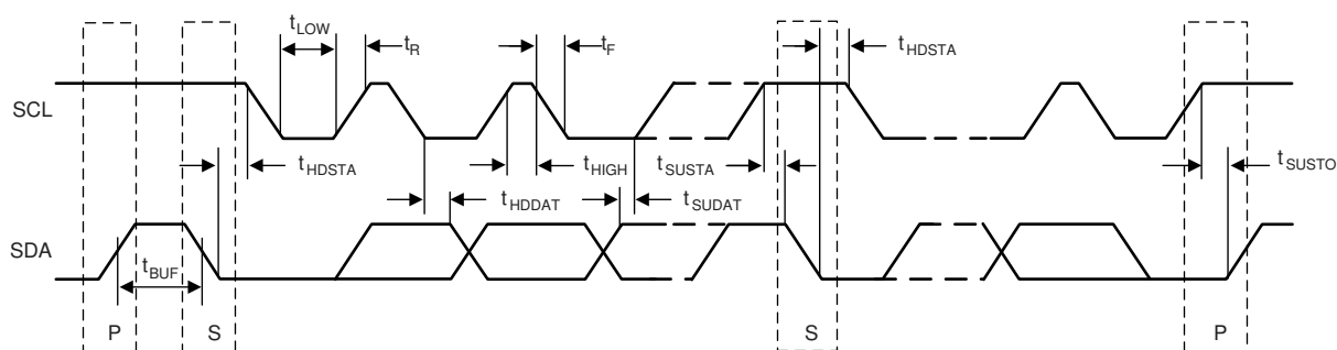
图 6-1. I 2 C Interface Timing
