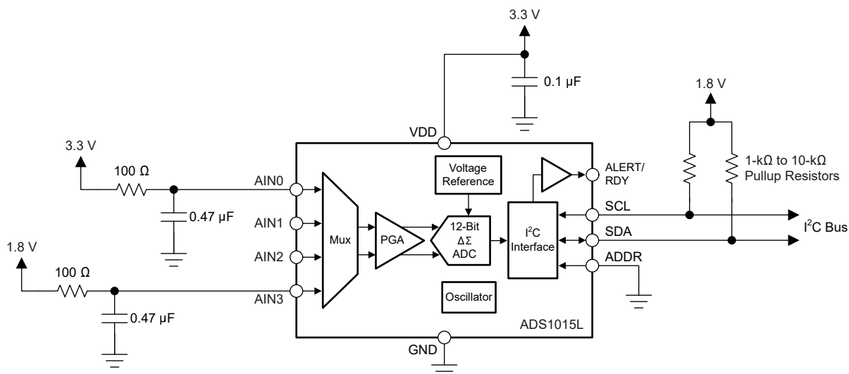
图 9-9. 监控两个电源电压轨：使用 ADS1015L
