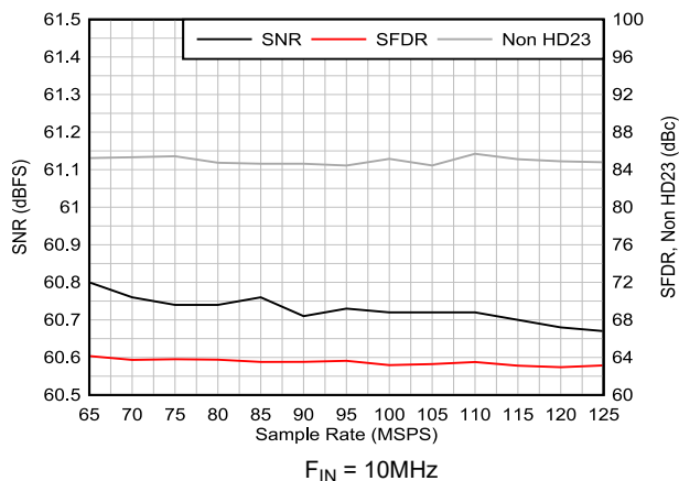
图 5-55. 交流性能与采样率间的关系
