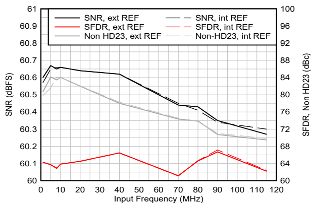
图 5-53. 交流性能与输入频率间的关系
